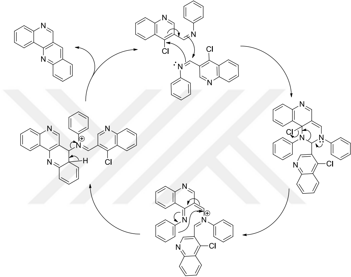
Şekil 6.4. Dibenzo[ b,h ][1,6]naftiridin eldesi oluşum mekanizması
