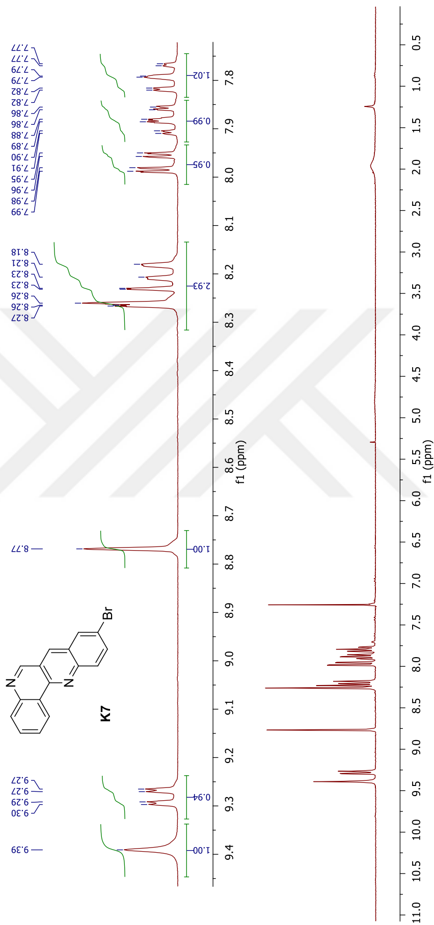
Ek 12: 9-bromodibenzo [b,h][1,6]naftiridin (K7) bileşiğinin ^1\text{H} NMR spektrumu
