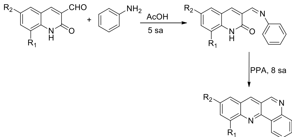
Şekil 2.9. Dibenzo[ b,h ][1,6]naftiridin oluşum reaksiyonu
