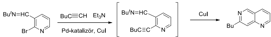
Şekil 2.6. 7-bütil-1,6-naftiridin oluşum reaksiyonu
