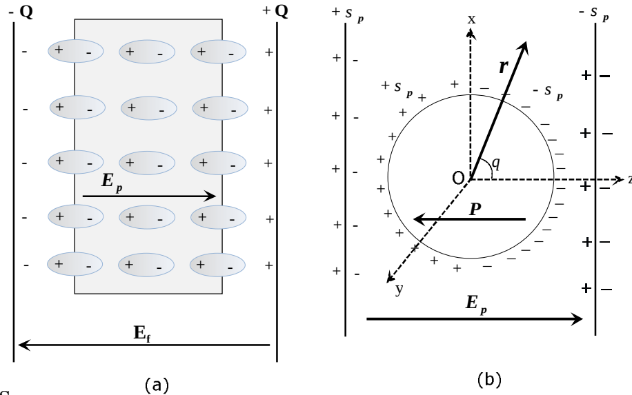
Ş Şekil 1.5. (a) arasında dielektrik bir madde bulunan yüklü bir kondansatör, (b) Dielektrik ortamda küresel oyuk
