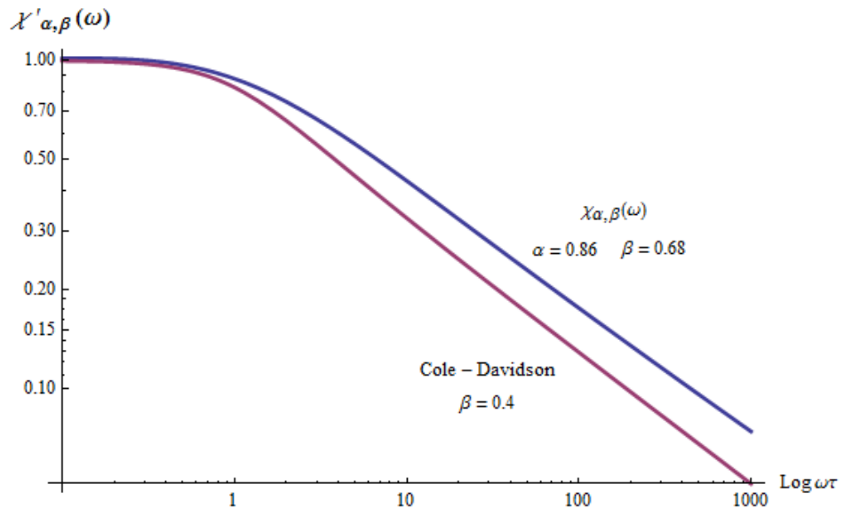
Şekil 4.12. Kesirli kompleks dielektrik fonksiyonu \chi_{\alpha,\beta}(\omega) ve Cole-Davidson denklemi reel eğrileri
