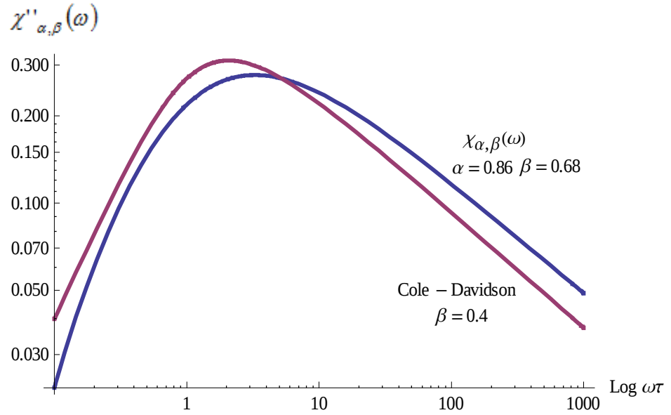
Şekil 4.11. Kesirli kompleks dielektrik fonksiyonu \chi_{\alpha,\beta}(\omega) ve Cole-Davidson denklemi kayıp eğrileri
