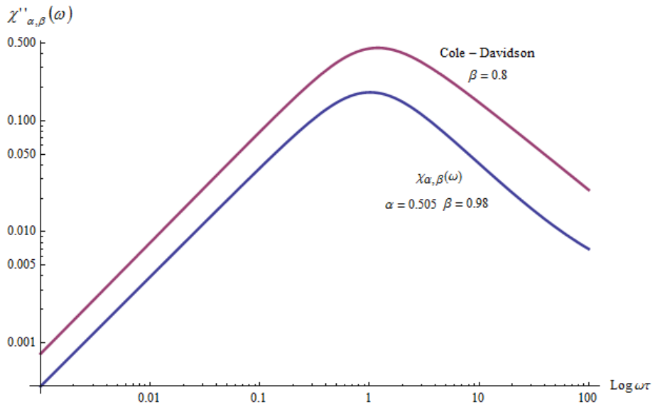
Şekil 4.13. Kesirli dielektrik fonksiyonu \chi_{\alpha,\beta}(\omega) ve Cole-Davidson denklemi kayıp eğrileri
