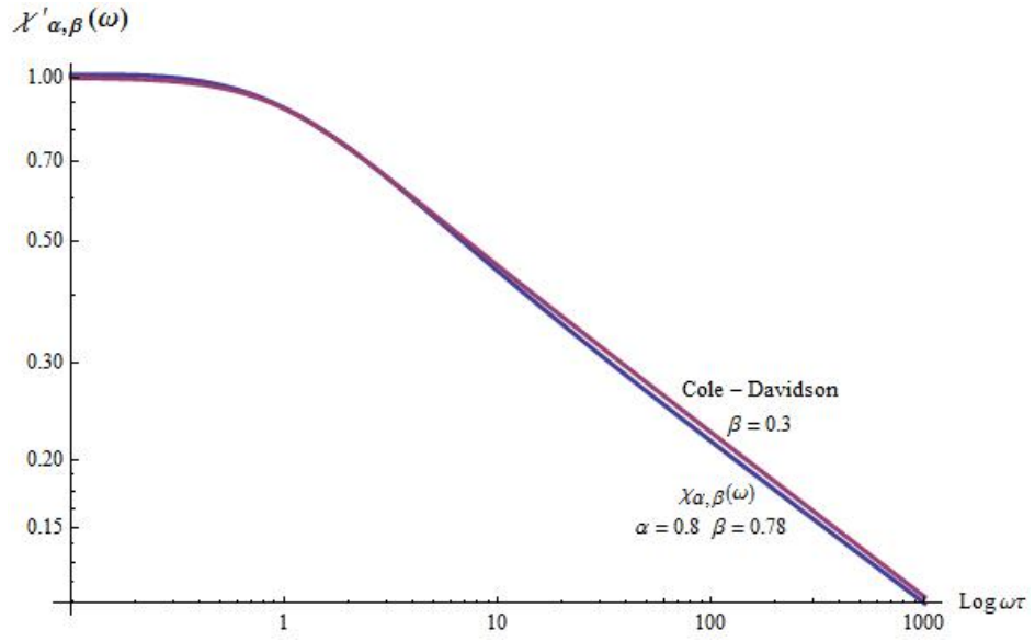
Şekil 4.10. Kesirli kompleks dielektrik fonksiyonu \chi'_{\alpha,\beta}(\omega) ve Cole-Davidson denklemi reel eğrileri
