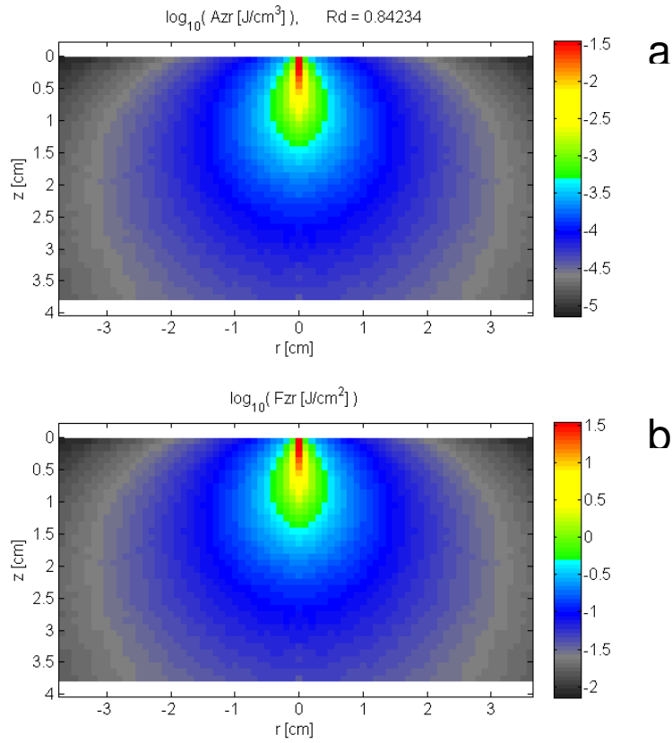
Şekil 11 : a) foton enerjisi b) akı yoğunluğu
