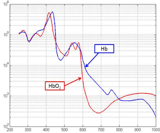
Şekil 5: Oksi ve Deoksi hemoglobinin molar uyarılma katsayıları
