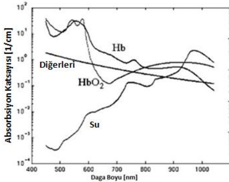
Şekil 2: Absorpsiyon katsayısının dalga boyuna göre değışimi
