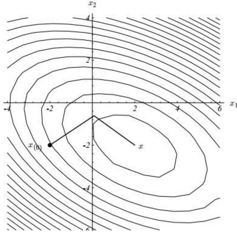
Şekil 17 : Conjugate Gradient metodu
