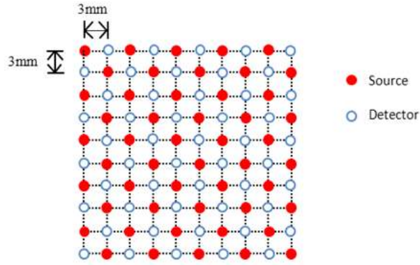
Şekil 9 : Kaynak detektör fiberlerinin prob üzerindeki yerleşimi
