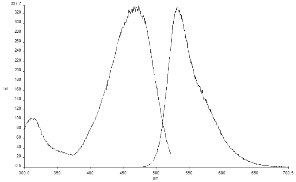
Şekil 3.92 DPP-1a2 türevinin tolüen çözütüsünde alınan emisyon-eksitasyon spektrumları
