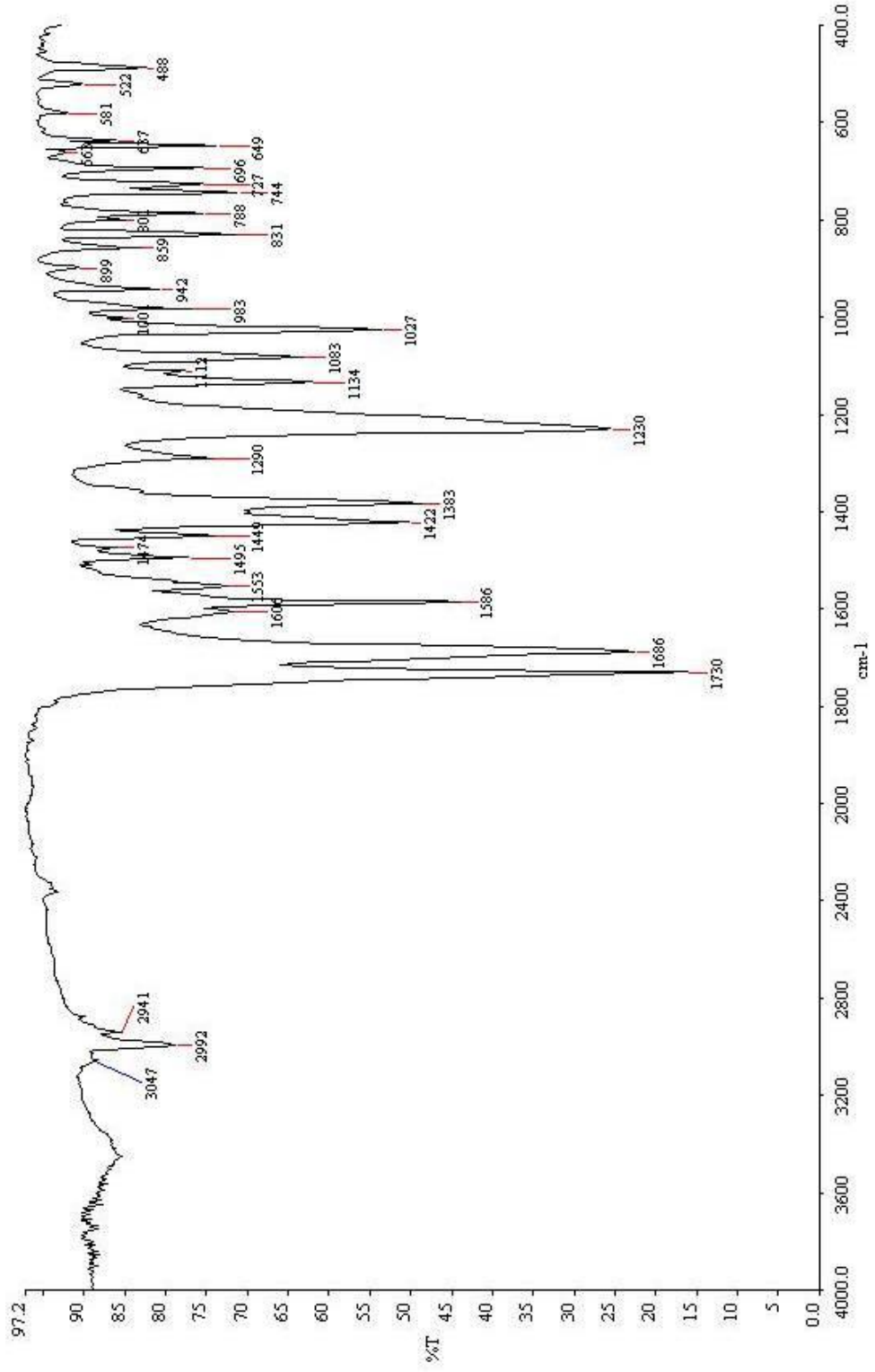
Şekil 3.31 Dietil 2,2'-(1,4-diokso-3-fenil-6-piridin-4-il-pirol-2,5-diil)diasetat (turuncu) (DPP-1b2) türevinin KBr de çekilen FT-IR spektrumu
