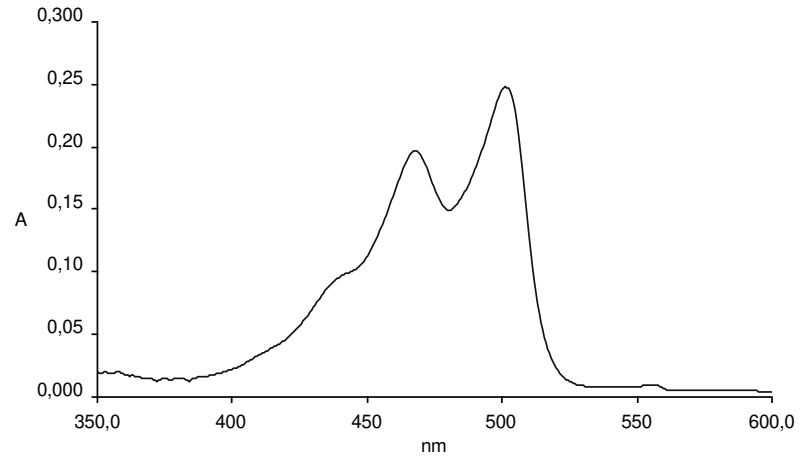
Şekil 3.163 Butil-DPP-H türevinin tetrahidrofur an çözücüsünde alınan absorpsiyon spektrumu
