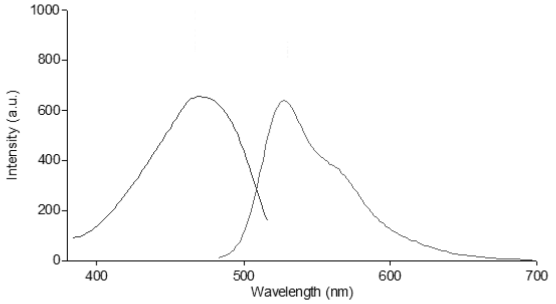
Şekil 3.182 Hekzil-DPP-Hekzil türevinin tetrahidrofuran çözücüsünde alınan emisyon-eksitasyon spektrumları
