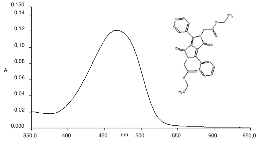
Şekil 3.103 DPP-1b2 türevinin tolüen çözütüsünde alınan absorpsiyon spektrumu
