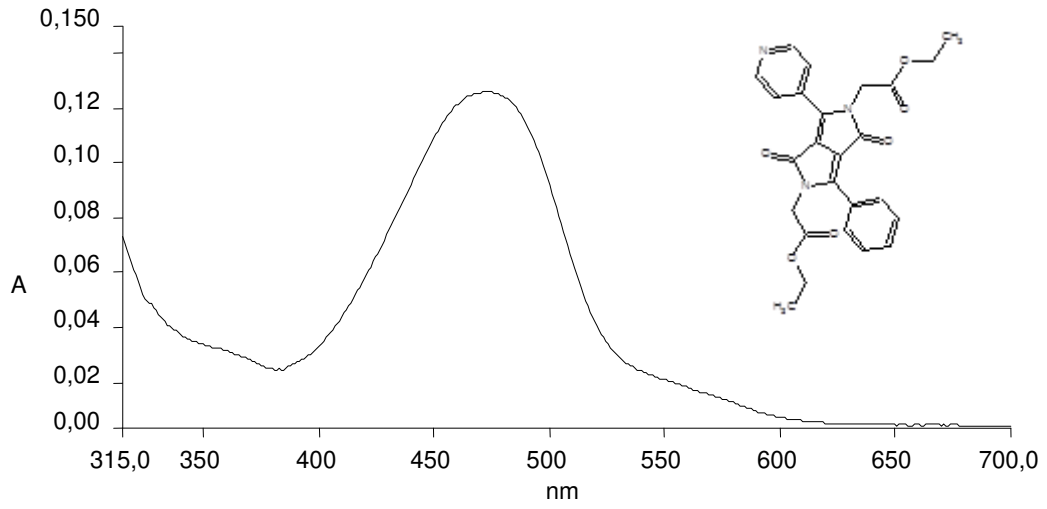
Şekil 3.105 DPP-1b2 türevinin PVC katı matriksinde alınan absorpsiyon spektrumu
