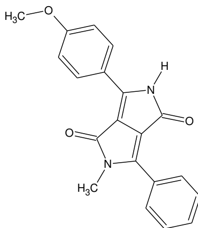
Şekil 3.53 3-fenil,6-metoksifenil-2-hidro-5-metilpirolo[3,4-c]pirol-1,4-dion türevi (DPP-3a1)
