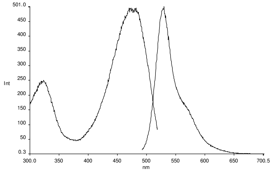
Şekil 3.144 DPP-3a2 türevinin kloroform çözücüsünde alınan emisyon-eksitasyon spektrumları
