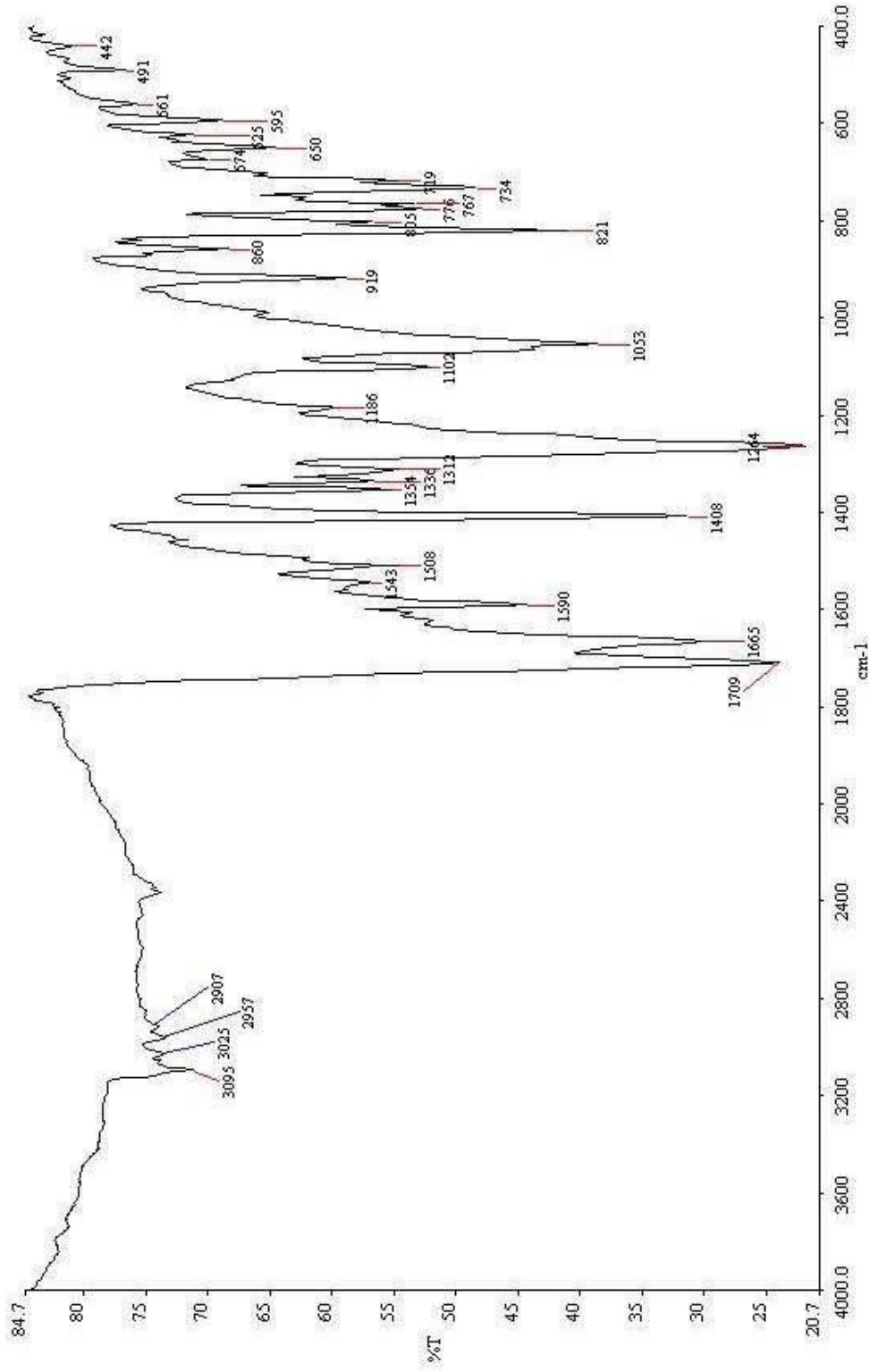
Şekil 3.50 3-tolil-6-piridil-2,5-ditiyofenilkarbonilpirolo [3,4-clpirol-1,4-dion (DPP-2c2) türevinin KBr’de çekilmiş FT-IR spektrumu
