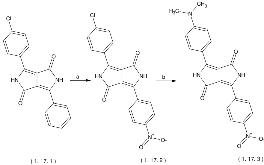
Şekil 1.17 DPP'deki klorürün nükleofilik aromatik sübstütüsyonu ve nitrolama a) \text{KNO}_3, \text{H}_2\text{SO}_4, 0-5^\circ\text{C}, 1 \text{ sa.} ; b) \text{Me}_2\text{NH}, \text{N-metil-2-pirrolidon}, 180^\circ\text{C}, 10 \text{ sa.} , otoklavda.
