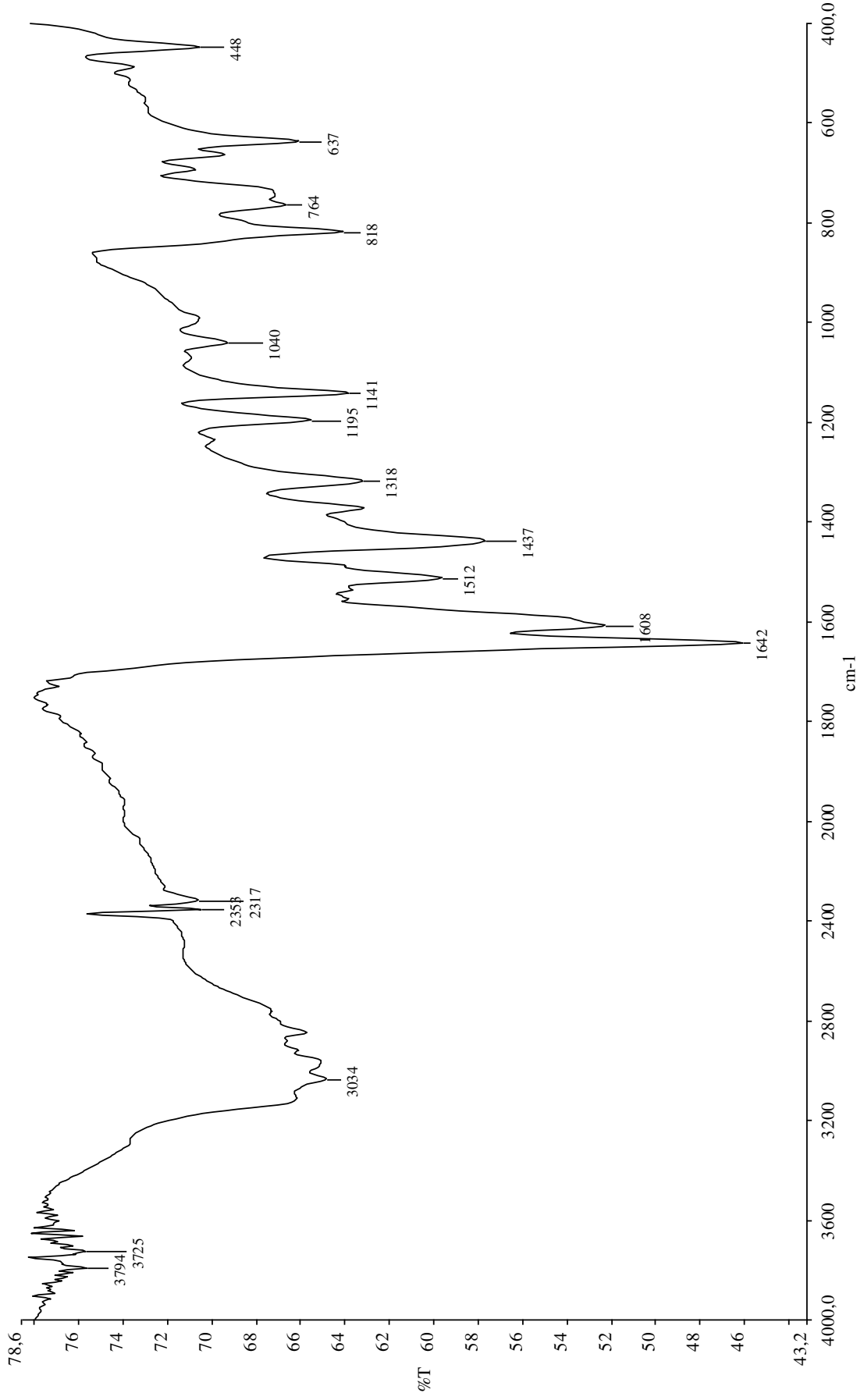
Şekil 3.23 3-bifenil-6-piridil-2,5-dihidropirolol[3,4-c]pirol-1,4-dion (DPP-7) türevinin KBr de çekilen FT-IR spektrumu
