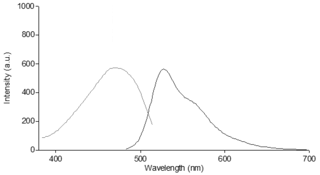
Şekil 3.194 Dodesil-DPP-Dodesil türevinin tetrahidrofuran çözücüsünde alınan emisyon-eksitasyon spektrumları
