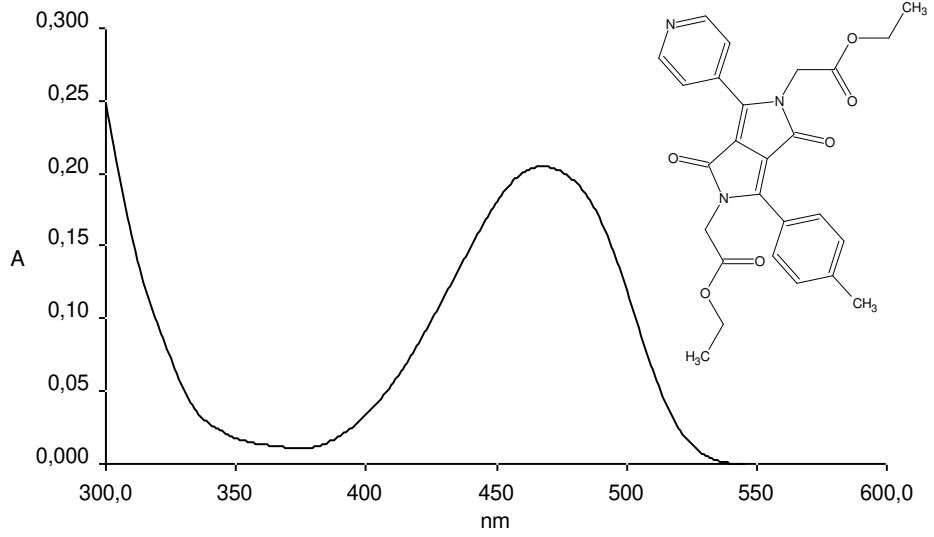
Şekil 3.119 DPP-2b2 türevinin kloroform çözücüsünde alınan absorpsiyon spektrumu
