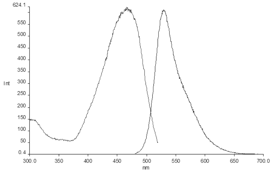
Şekil 3.104 DPP-1b2 türevinin tolüen çözütüsünde alınan emisyon- eksitasyon spektrumları
