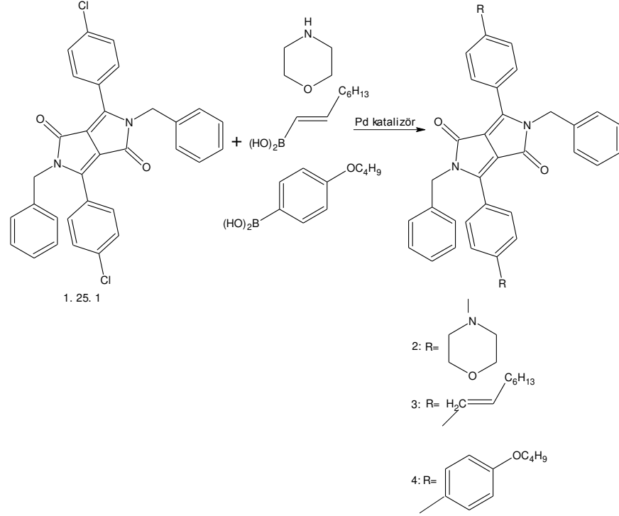
Şekil 1.25 Çapraz bağlama ile farklı DPP türevlerinin sentezi
