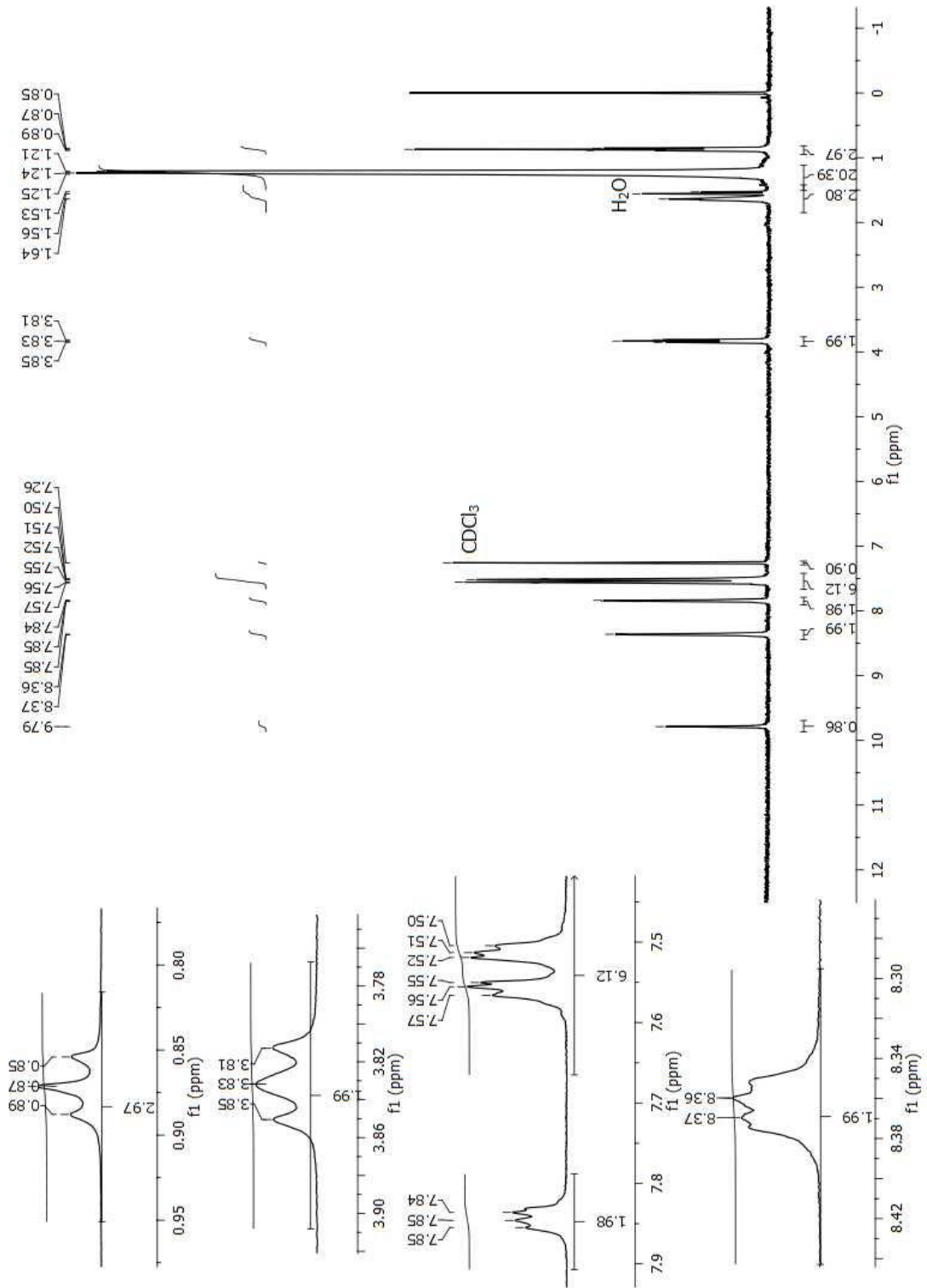
Şekil 3.79 3,6-difenil-2-hidro-5-dodesilpirolo[3,4-c]pirol-1,4-dion türevinin \text{CDCl}_3 'da çekilen ^1\text{H} -NMR spektrumu
