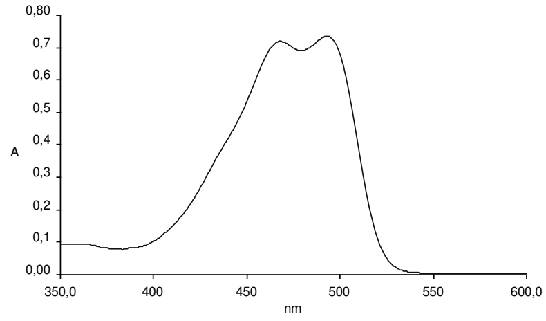
Şekil 3.175 Hekzil-DPP-H türevinin tetrahidrofuran çözücüsünde alınan absorpsiyon spektrumu
