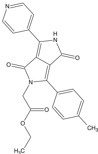
Şekil 3.41 Etil[6-(4-metilfenil)-1,4-diokso-3-piridin-4-yl-4,5-dihidropirrol-2(1H)-yl]asetat (DPP-2b1) Türevi
