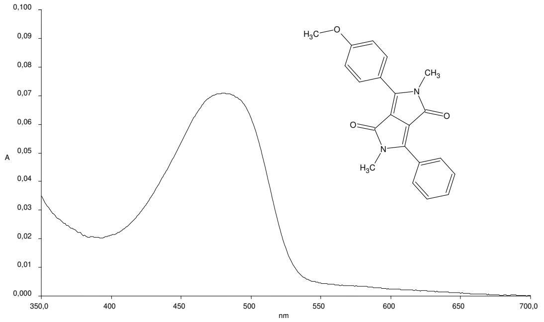
Şekil 3.139 DPP-3a2 türevinin dimetilformamid çözücüsünde alınan absorpsiyon spektrumu
