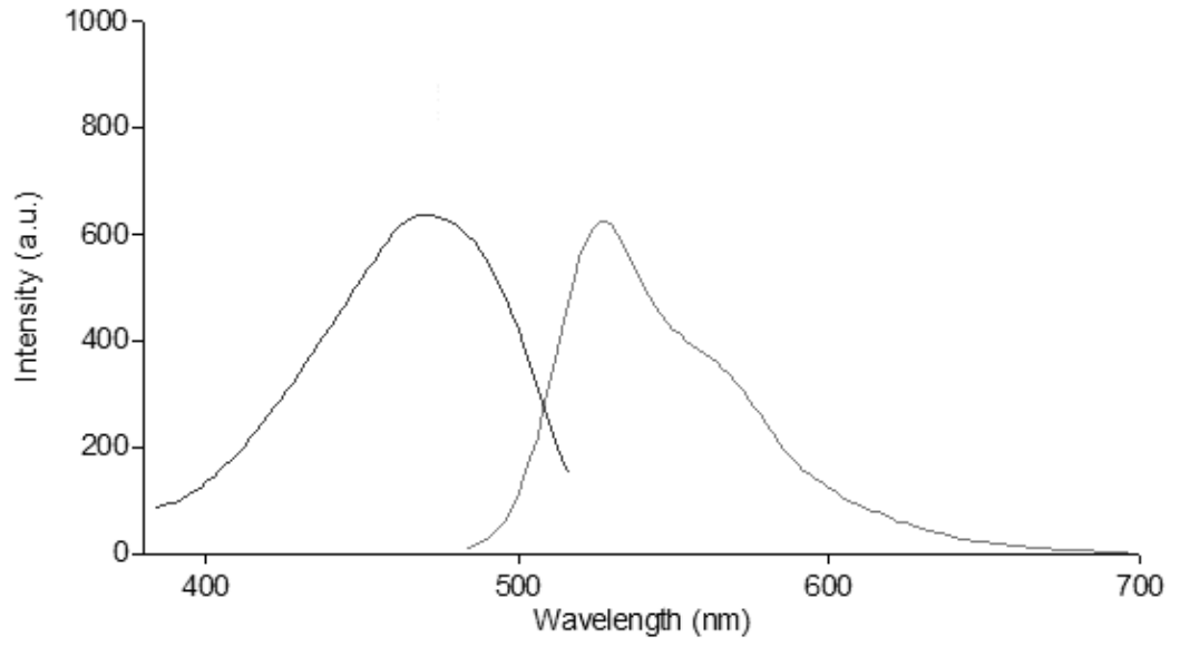
Şekil 3.170 Butil-DPP-Butil türevinin tetrahidrofuran çözücüsünde alınan emisyon-eksitasyon spektrumları
