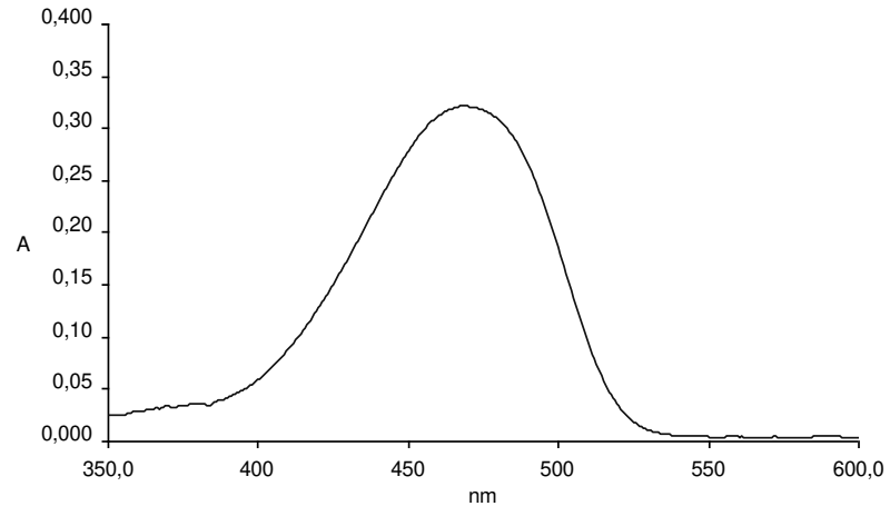
Şekil 3.181 Hekzil-DPP-Hekzil türevinin tetrahidrofuran çözücüsünde alınan absorpsiyon spektrumu
