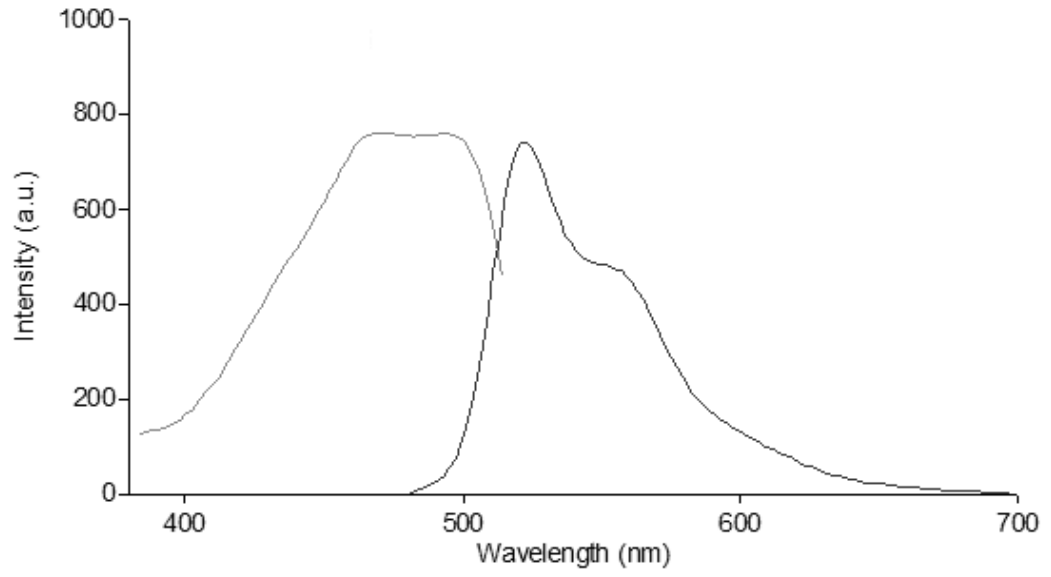
Şekil 3.188 Dodesil-DPP-H türevinin tetrahidrofuran çözücüsünde alınan emisyon-eksitasyon spektrumları
