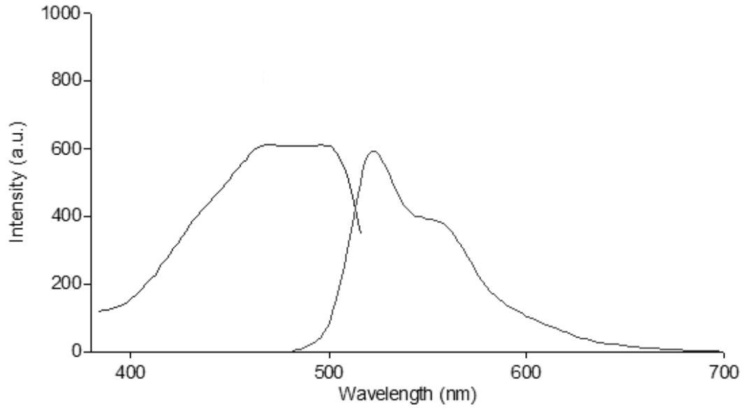
Şekil 3.176 Hekzil-DPP-H türevinin tetrahidrofuran çözücüsünde alınan emisyon-eksitasyon spektrumları
