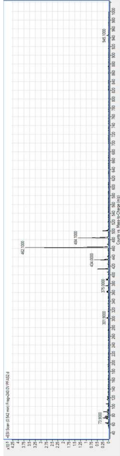
Şekil 3.35 Dietil 2,2'-(1,4-dikso-3-fenil-6-piridin-4-il-pirol-3,4-c)pirol-2,5-diil)diasetat (turuncu) (DPP-1b2) türevinin LC-MS spektrumu
