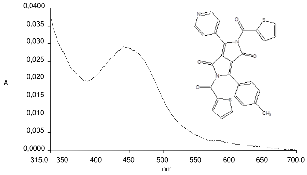
Şekil 3.137 DPP-2c2 türevinin PVC katı matriksinde alınan absorpsiyon spektrumu
