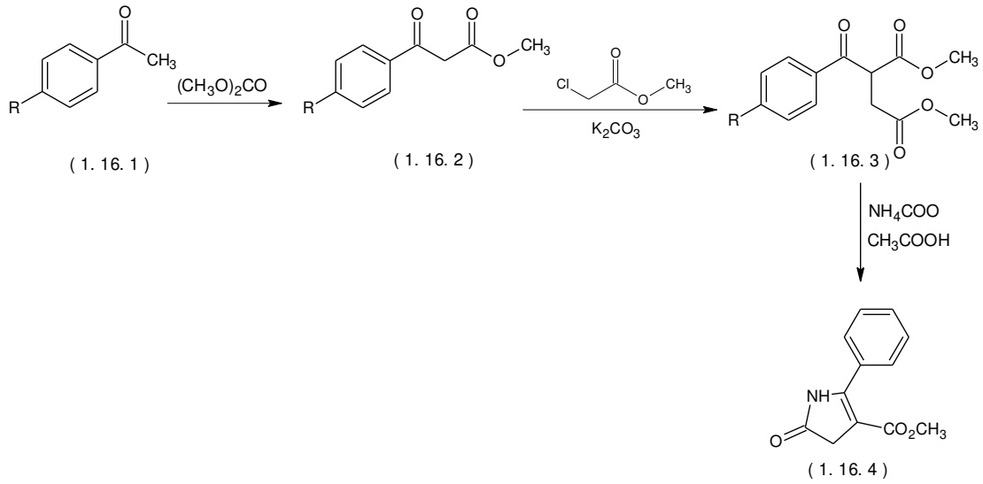
Şekil 1.16 Langhals ve Potrawa tarafından önerilen pirolinon ester sentezi
