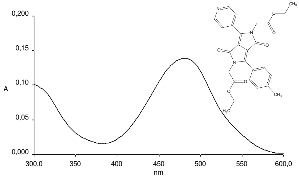
Şekil 3.123 DPP-2b2 türevinin tolüen çözütüsünde alınan absorpsiyon spektrumu
