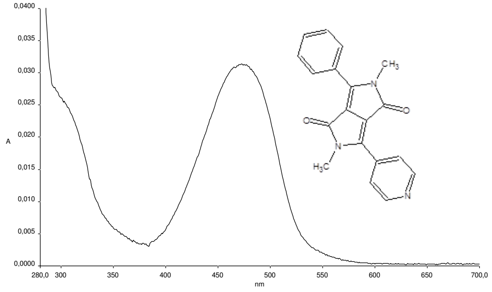
Şekil 3.91 DPP-1a2 türevinin tolüen çözütüsünde alınan absorpsiyon spektrumu
