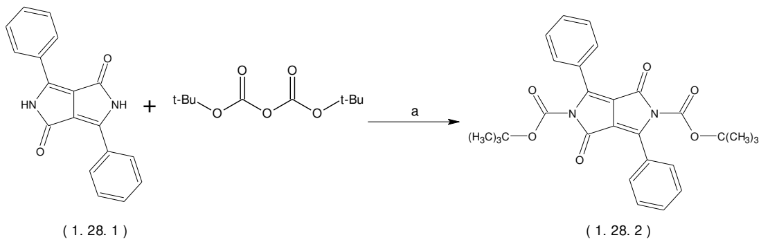
Şekil 1.28 Di-ter-butil dikarbonat ile DPP'nin açılması
