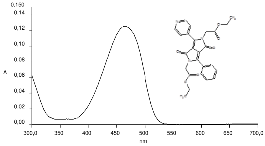
Şekil 3.101 DPP-1b2 türevinin tetrahidrofuran çözücüsünde alınan absorpsiyon spektrumu
