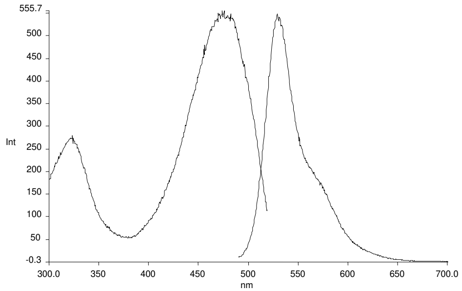
Şekil 3.140 DPP-3a2 türevinin dimetilformamid çözücüsünde alınan emisyon-eksitasyon spektrumları
