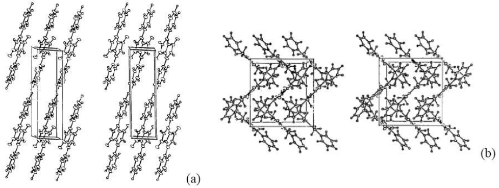
Şekil 1.33 (a) DPP-triklinik (b) DPP-Me-diküçükseksen'lerin kristal yapılarının birim hücre içinde stereo gösterimi (Mizuguchi ve diğer., 1992)
