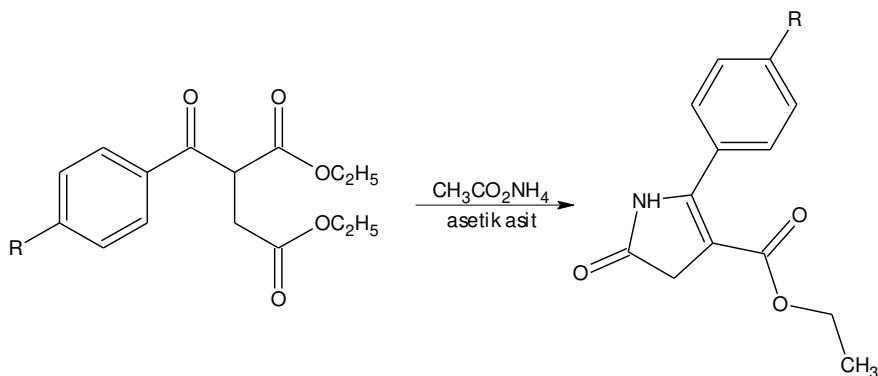
Şekil 2.3 2-aril-3-etoksikarbonil-2-pirolin-5-on türevinin genel sentez reaksiyonu
