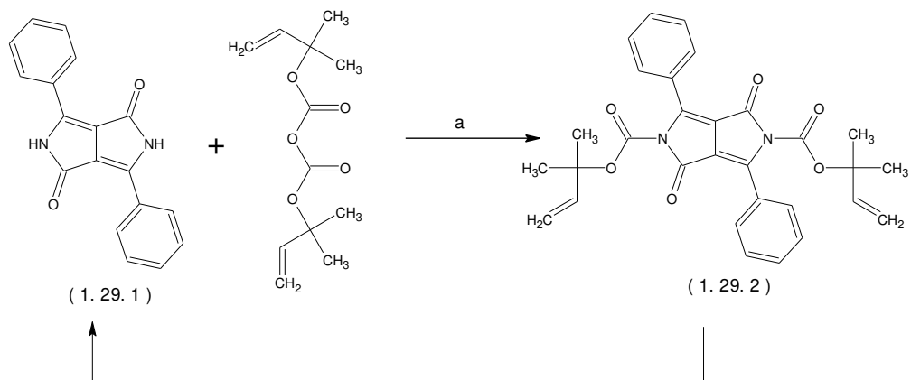
Şekil 1.29 DPP'nin di(2-metil-3-büten-2-yl) dikarbonat ile açılması ve bozunması
