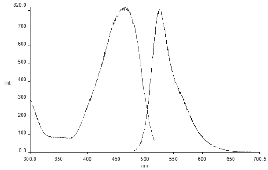
Şekil 3.102 DPP-1b2 türevinin tetrahidrofuran çözücüsünde alınan emisyon- eksitasyon spektrumları
