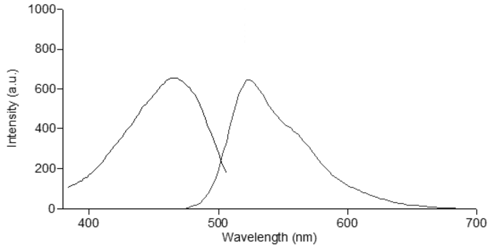
Şekil 3.180 Hekzil-DPP-Hekzil türevinin asetonitril çözücüsünde alınan emisyon-eksitasyon spektrumları
