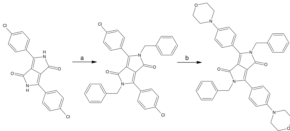
Şekil 1.24 Pd katalizörlü aminleme reaksiyonu (a) benzil bromür, K 2 CO 3 , DMF, 120 °C, %70 verim; (b) Pd(OAc) 2 /SPhos, t-BuONa, toluen, 100 °C, % 88 verim.
