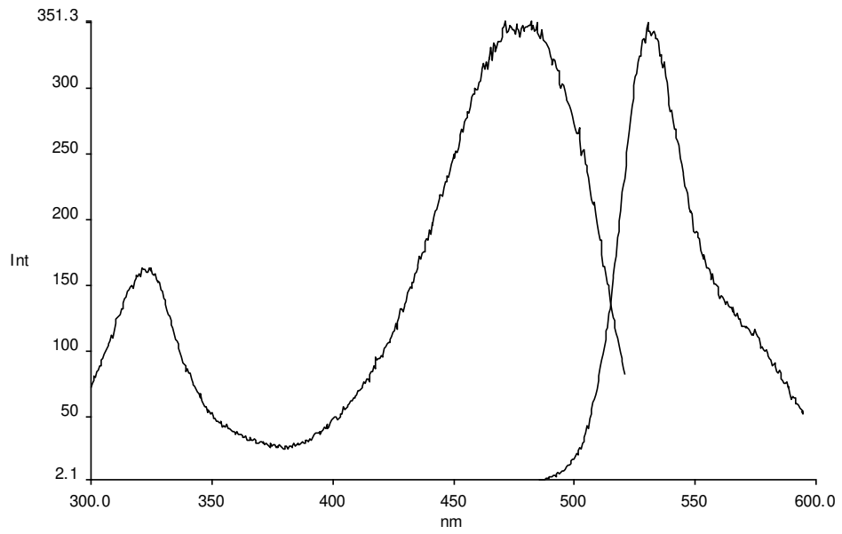
Şekil 3.148 DPP-3a2 türevinin tolüen çözütüsünde alınan emisyon-eksitasyon spektrumları
