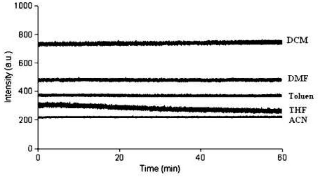
Şekil 3.203 Dodesil-DPP-Dodesil türevinin farklı çözücü sistemlerinde alınan fotokararlılıkları
