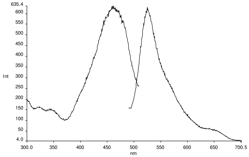
Şekil 3.106 DPP-1b2 türevinin PVC katı matriksinde alınan emisyon- eksitasyon spektrumları
