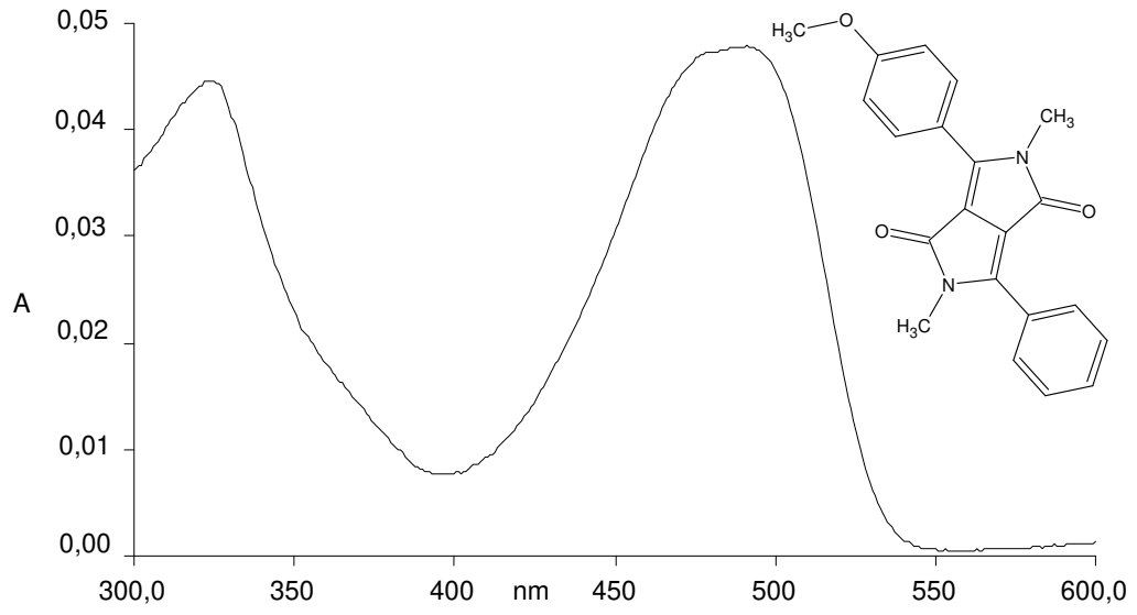
Şekil 3.147 DPP-3a2 türevinin tolüen çözütüsünde alınan absorpsiyon spektrumu
