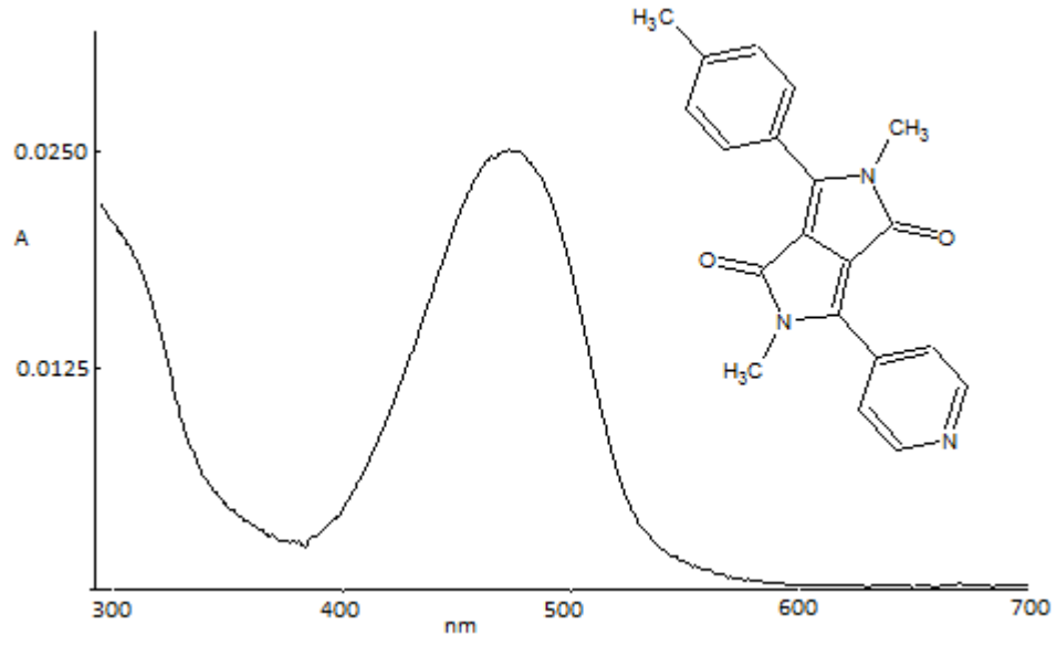
Şekil 3.111 DPP-2a2 türevinin tetrahidrofuran çözücüsünde alınan absorpsiyon spektrumu
