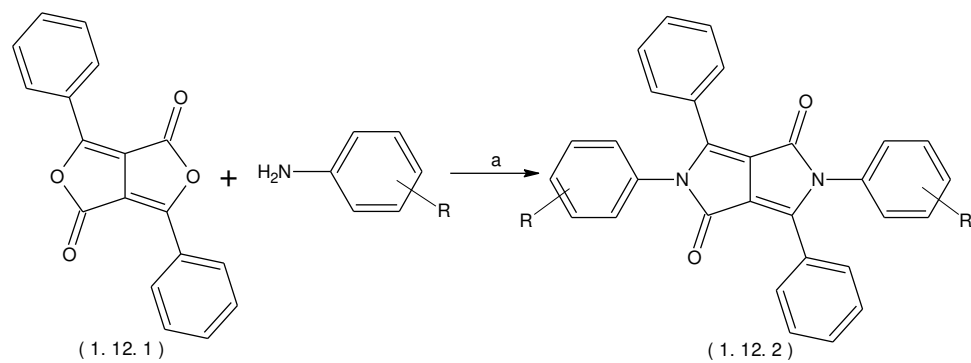
Şekil 1.12 3,6-difenil-1H,4H-furo[3,4-c]furan-1,4-dion'un anilinle kondenzasyonu (R: H, 4-Me, 2,3- Me 2 , 4-t-Bu) a) DCC, CF 3 COOH, CHCl 3 , oda sıc., 3 gün
