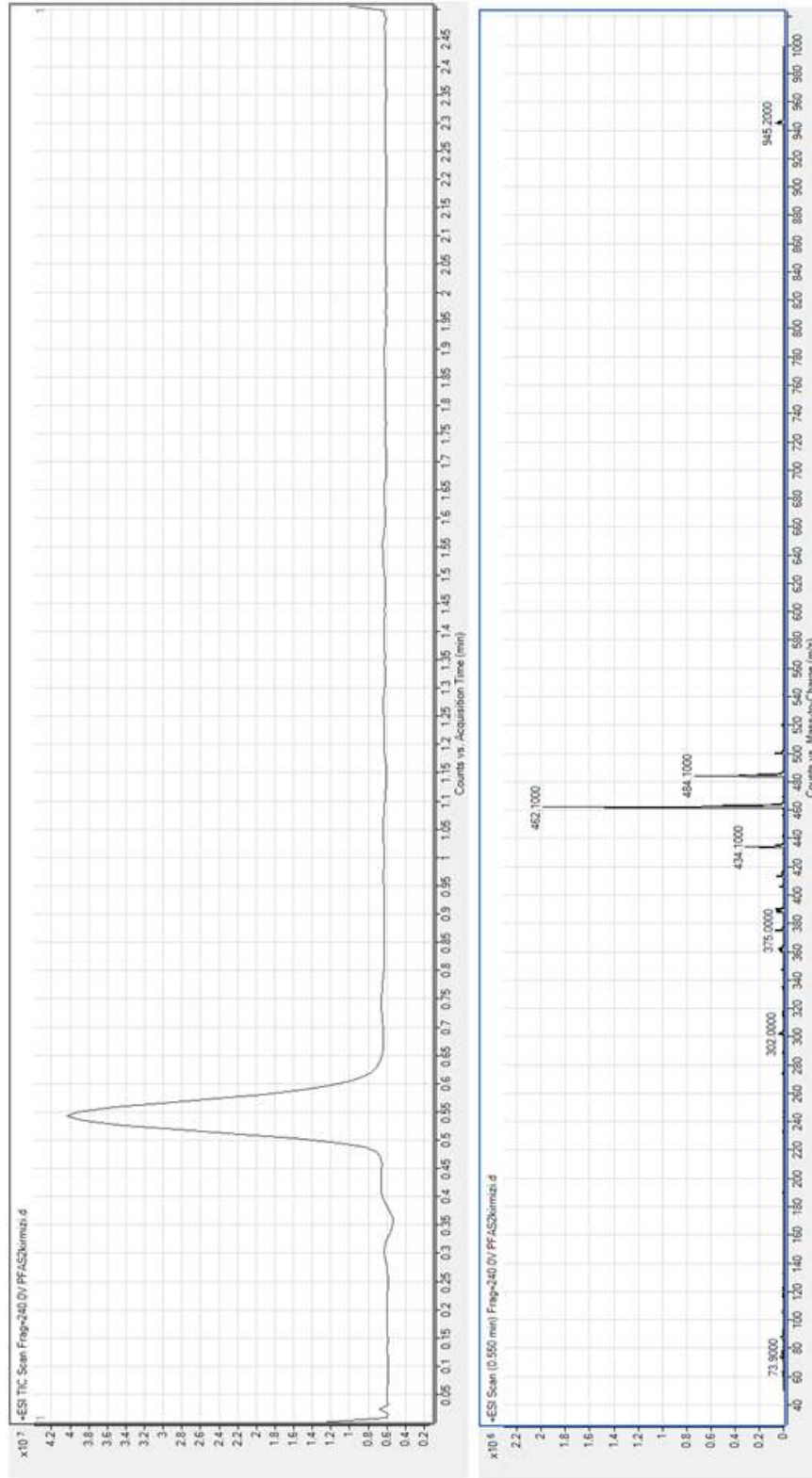
Şekil 3.36 Dietil 2,2'-(1,4-diookso-3-fenil-6-piridin-4-il-pirol[3,4-c]pirol-2,5-dii)diasetat (kırmızı) (DPP-1b2) türevinin LC-MS spektrumu
