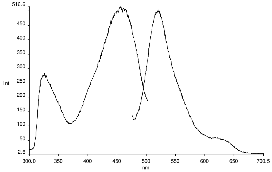
Şekil 3.138 DPP-2c2 türevinin PVC katı matriksinde alınan emisyon-eksitasyon spektrumları
