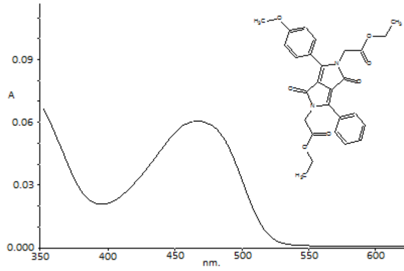
Şekil 3.151 DPP-3b2 türevinin dimetilformamid çözütüsünde alınan absorpsiyon spektrumu
