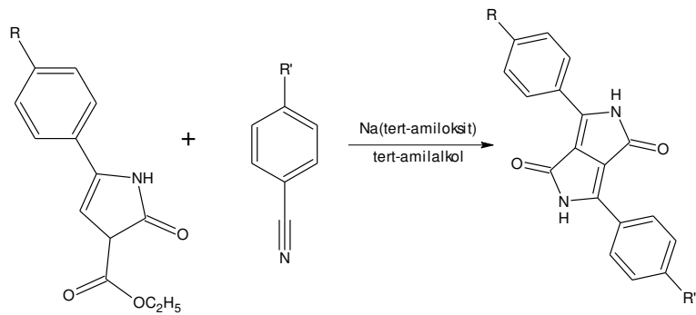
Şekil 2.4 Antisimetrik Diketopirolopirol türevinin sentez reaksiyonu
