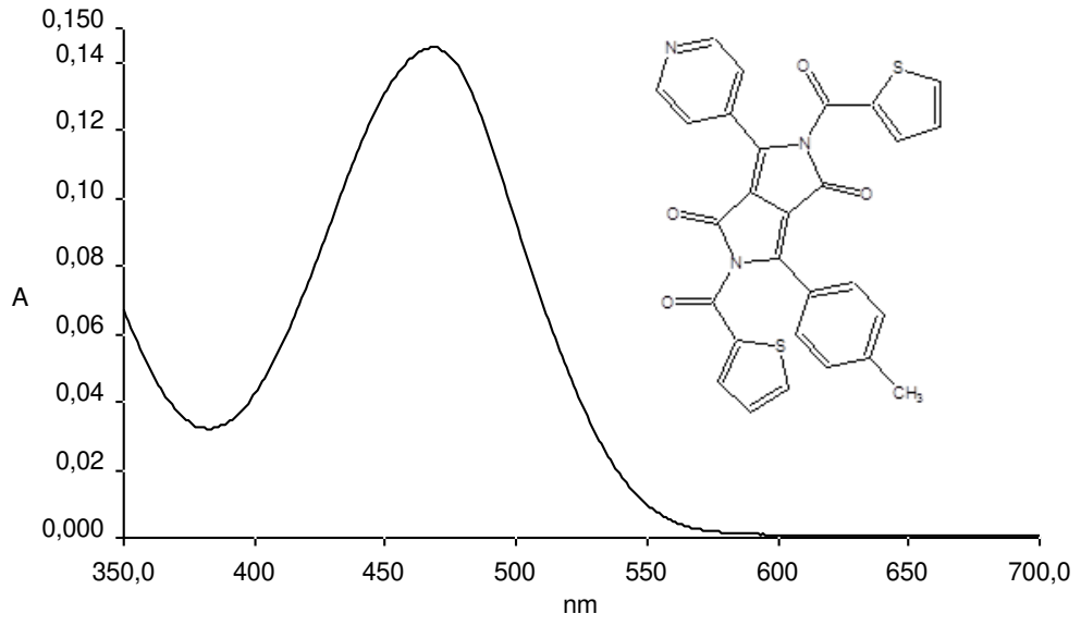
Şekil 3.135 DPP-2c2 türevinin tolüen çözütüsünde alınan absorpsiyon spektrumu
