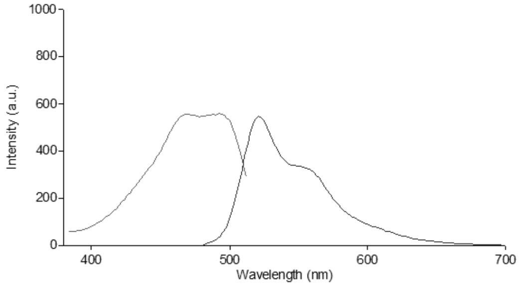
Şekil 3.164 Butil-DPP-H türevinin tetrahidrofur an çözücüsünde alınan emisyon-eksitasyon spektrumları
