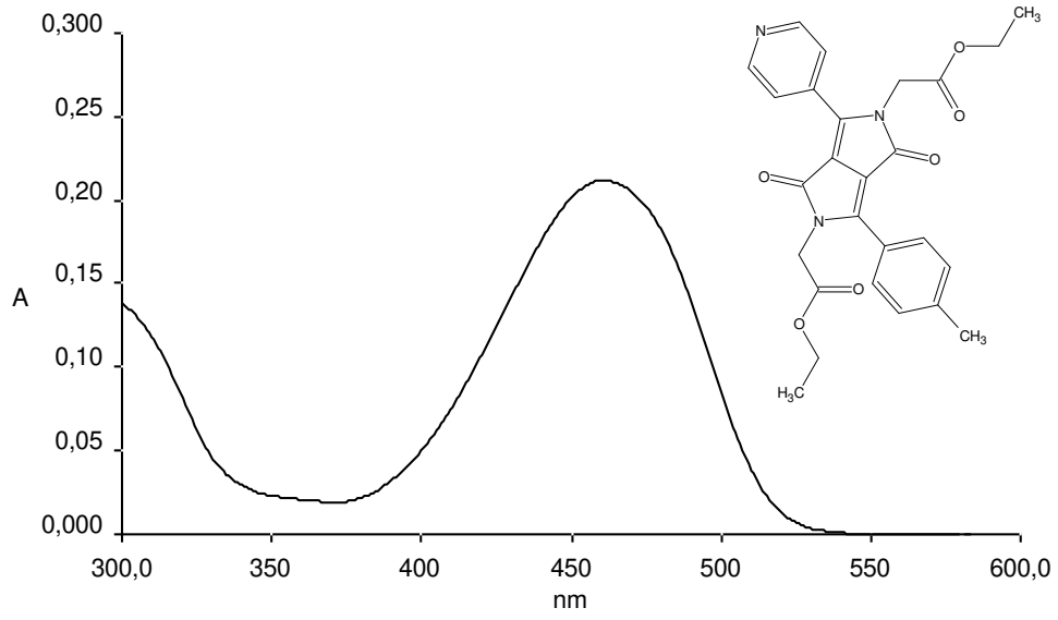
Şekil 3.117 DPP-2b2 türevinin asetonitril çözücüsünde alınan absorpsiyon spektrumu
