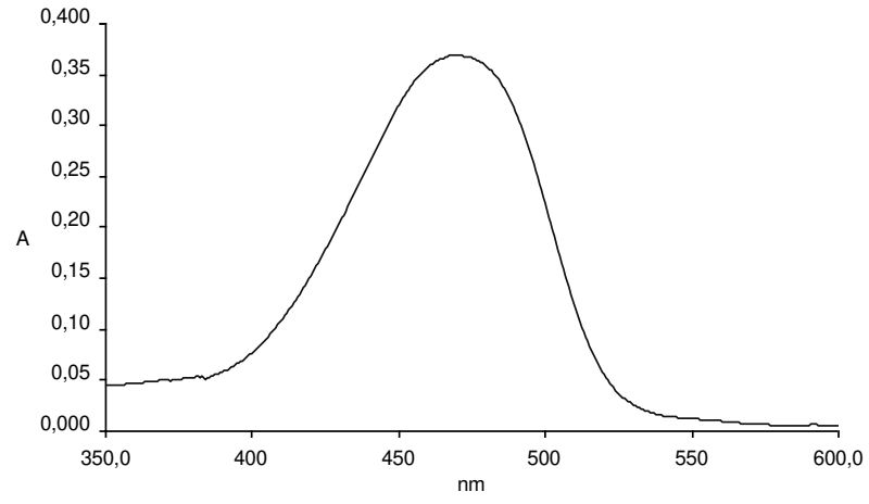
Şekil 3.193 Dodesil-DPP-Dodesil türevinin tetrahidrofuran çözücüsünde alınan absorpsiyon spektrumu
