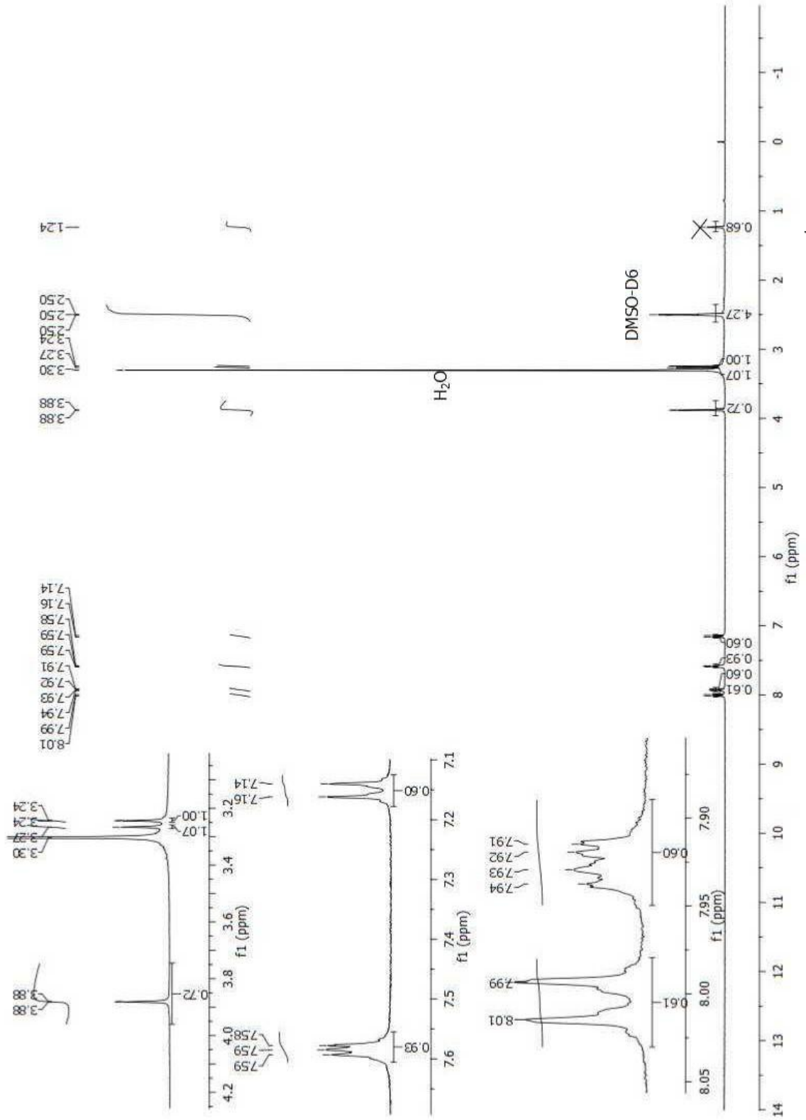
Şekil 3.57 3-fenil-6-metoksifenil-2,5-dimetilpirolo [3,4-c]pirol-1,4-dion (DPP-3a2) türevinin DMSO- \text{D}_6 'da çekilmiş ^1\text{H} -NMR spektrumu
