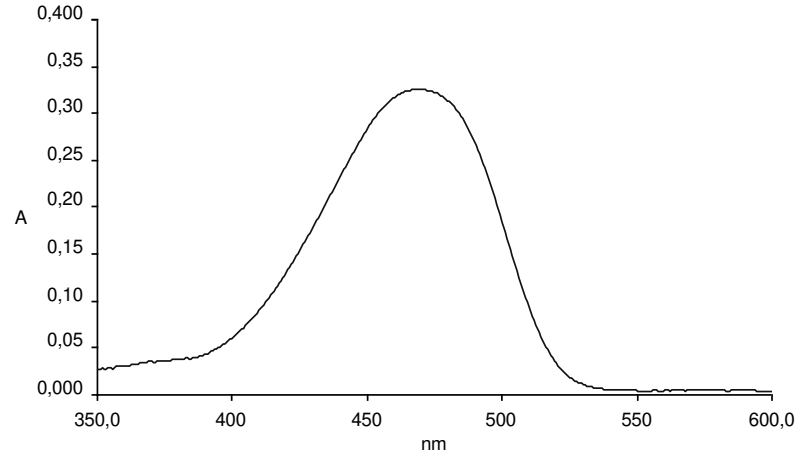
Şekil 3.169 Butil-DPP-Butil türevinin tetrahidrofuran çözücüsünde alınan absorpsiyon spektrumu
