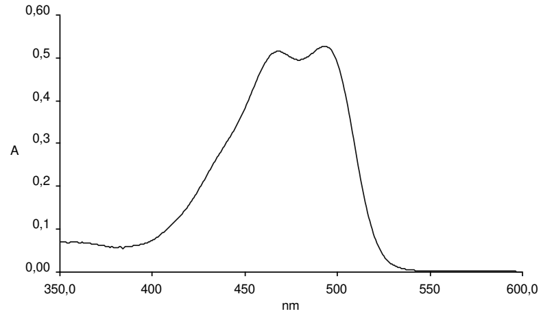
Şekil 3.187 Dodesil-DPP-H türevinin tetrahidrofuran çözücüsünde alınan absorpsiyon spektrumu
