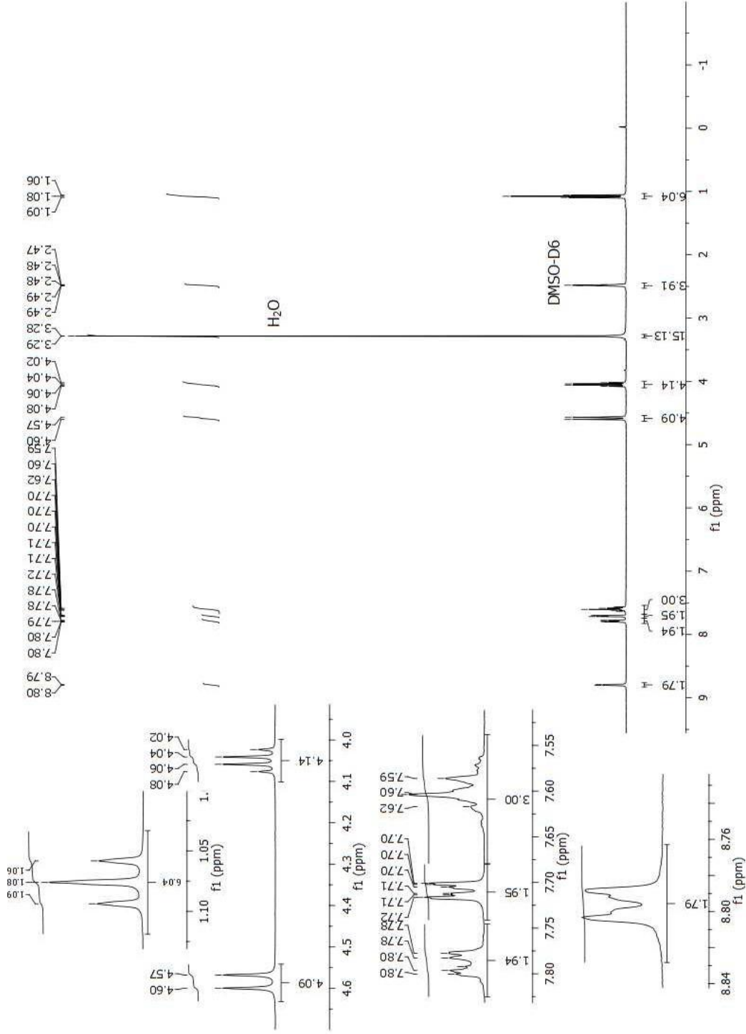
Şekil 3.33 Dietil 2,2'-(1,4-diokso-3-fenil-6-piridin-4-il-pirol-3,4-c)pirol-2,5-diil)diasetat (turuncu) (DPP-1b2) türevinin DMSO-D 6 'da çekilen 1 H-NMR spektrumu
