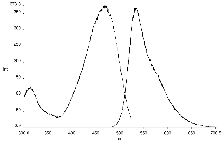
Şekil 3.124 DPP-2b2 türevinin tolüen çözütüsünde alınan emisyon- eksitasyon spektrumları
