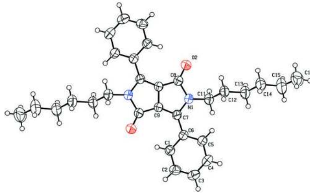
Şekil 1.35 N,N'-dihekzil DPP türevi (Sevinçek ve diğer, 2010).
