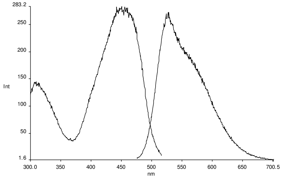
Şekil 3.136 DPP-2c2 türevinin tolüen çözütüsünde alınan emisyon-eksitasyon spektrumları
