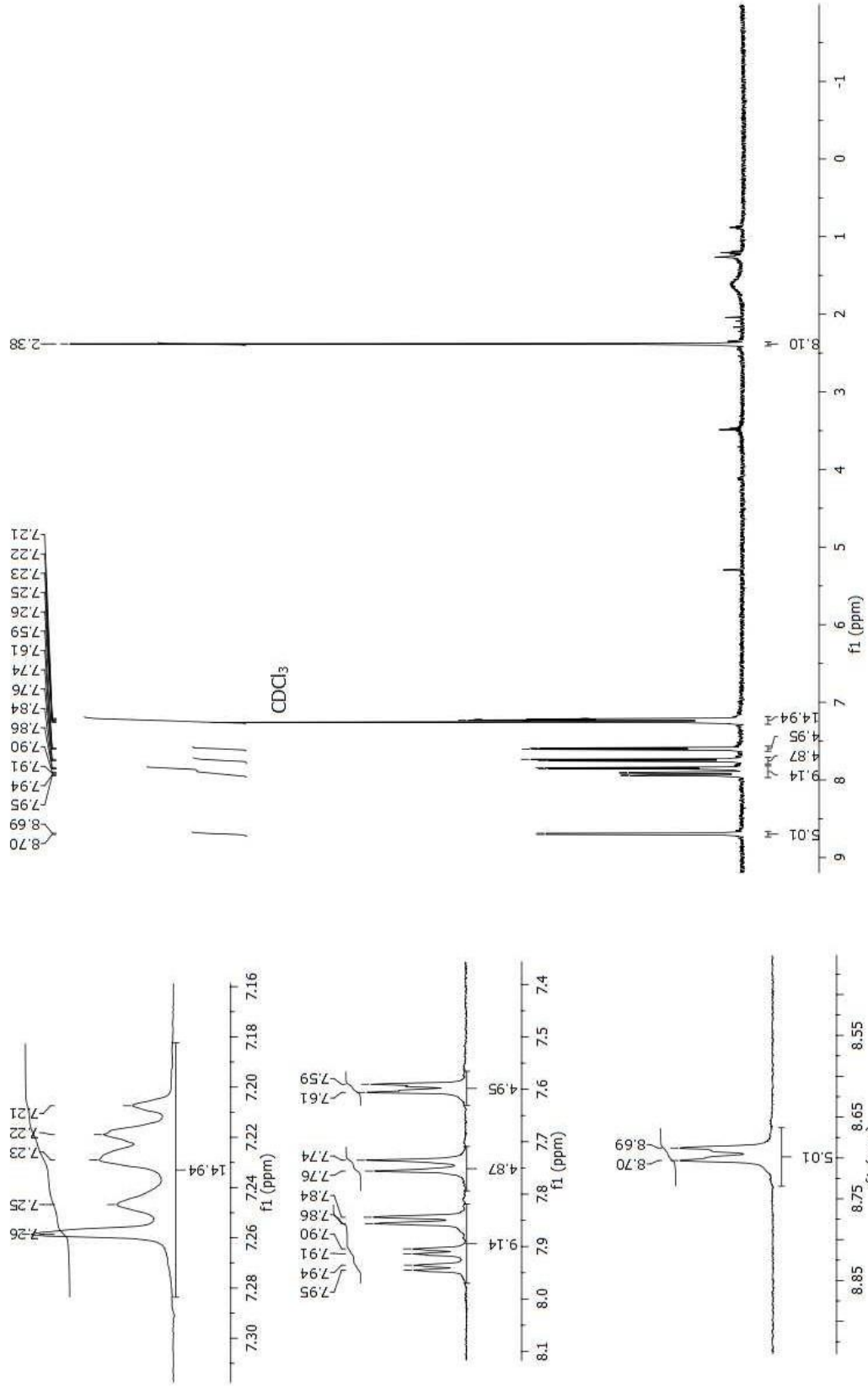
Şekil 3.51 3-tolil-6-piridil-2,5-ditiyofenilkarbonilpirolo [3,4-c]pirol-1,4-dion (DPP-2c2) türevinin \text{CDCl}_3 'de çekilmiş ^1\text{H} -NMR spektrumu
