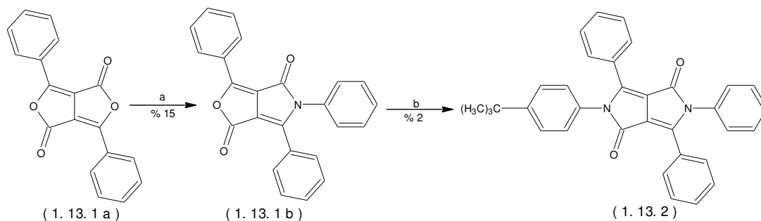
Şekil 1.13 Antisimetrik N,N'-diaryl DPP sentezi
