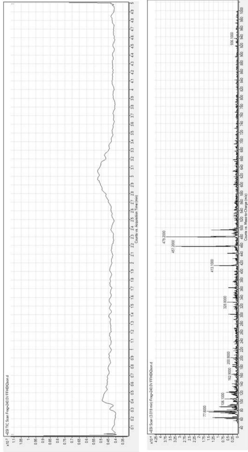
Şekil 3.76 3,6-difenil-2,5-diheksilpirolo[3,4-c]pirol-1,4-dion türevinin LC-MS spektrumu
