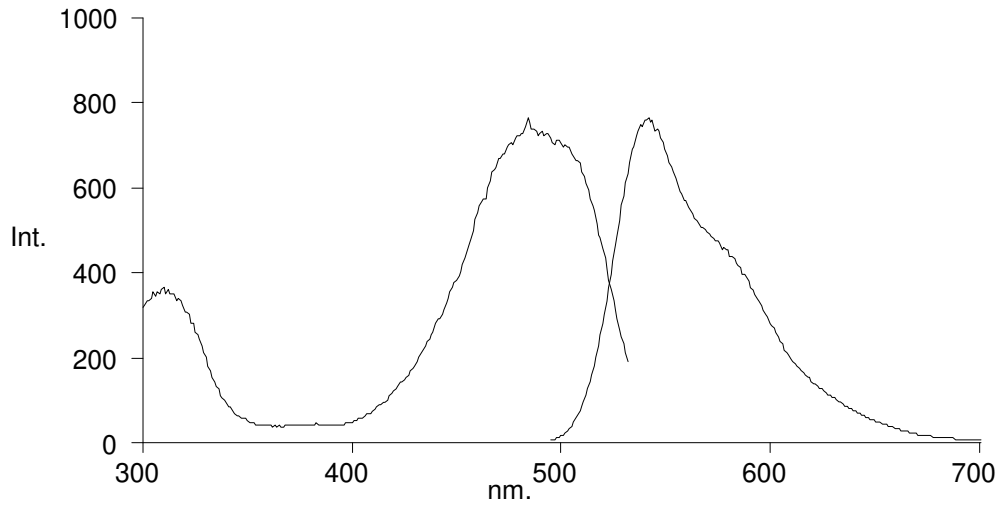
Şekil 3.112 DPP-2a2 türevinin tetrahidrofuran çözücüsünde alınan emisyon- eksitasyon spektrumları
