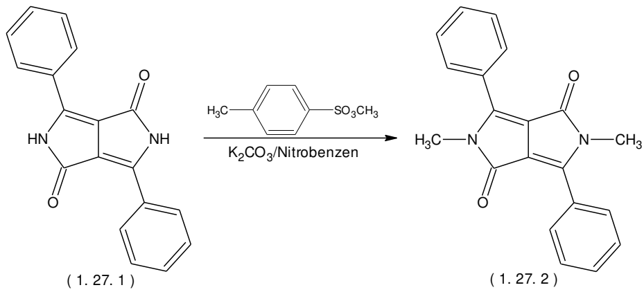
Şekil 1.27 DPP'nin N-metilasyonu
