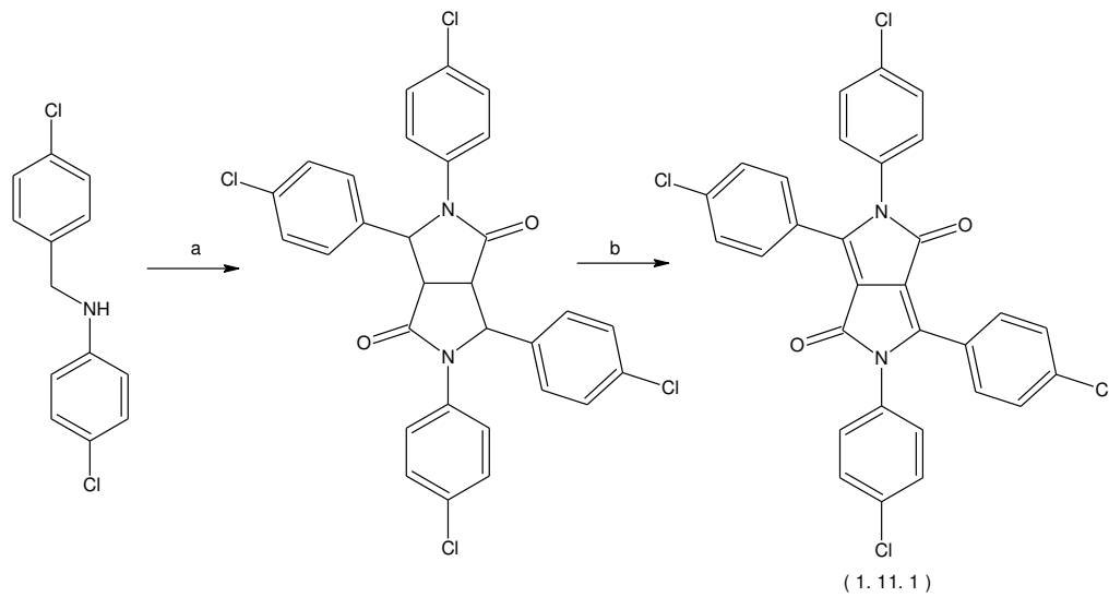
Şekil 1.11 Benzilanilin'den DPP sentezi
