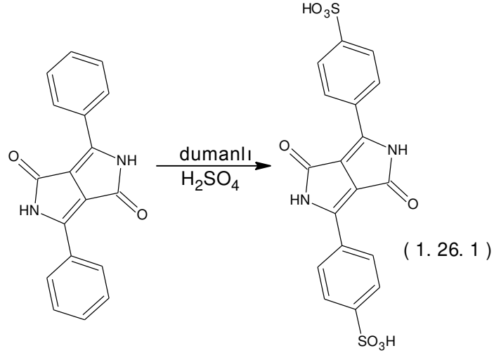
Şekil 1.26 DPP'nin Sülfolanması
