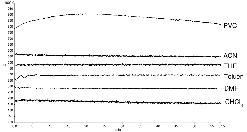
Şekil 3.196 DPP-1b2 türevinin farklı çözücü sistemlerinde alınan fotokararlılıkları
