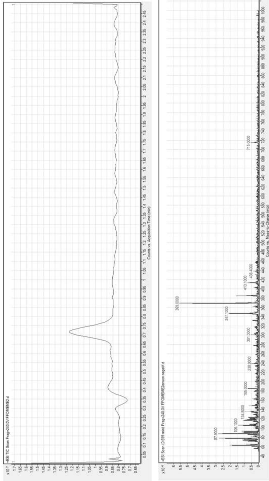
Şekil 3.58 3-fenil-6-metoksifenil-2,5-dimetilpirolo [3,4-c]pirol-1,4-dion (DPP-3a2) türevinin LC-MS spektrumu
