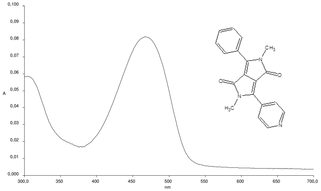
Şekil 3.83 DPP-1a2 türevinin dimetilformamid çözücüsünde alınan absorpsiyon spektrumu
