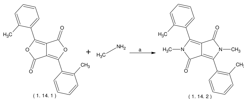
Şekil 1.14 Furo[3,4-c]furan-1,4-dion ile alifatik aminin reaksiyonu
