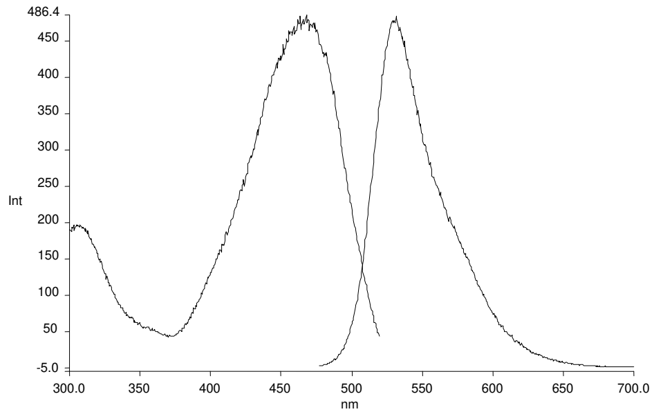
Şekil 3.84 DPP-1a2 türevinin dimetilformamid çözücüsünde alınan emisyon-eksitasyon spektrumları
