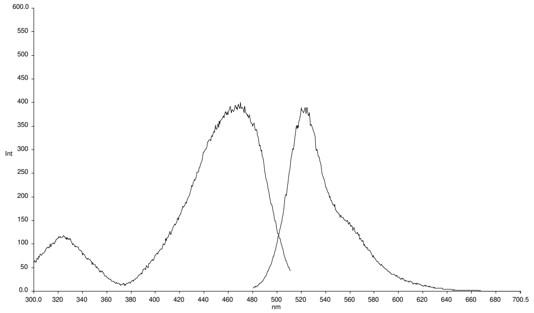
Şekil 3.152 DPP-3b2 türevinin dimetilformamid çözütüsünde alınan emisyon-eksitasyon spektrumları
