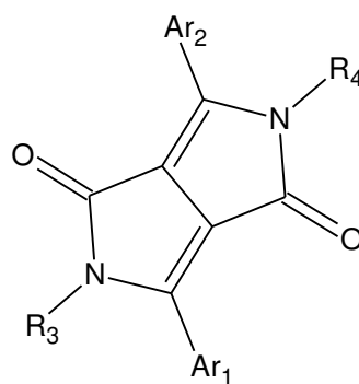
Şekil 4.1 Sentezlenen DPP türevlerinin genel gösterimi
