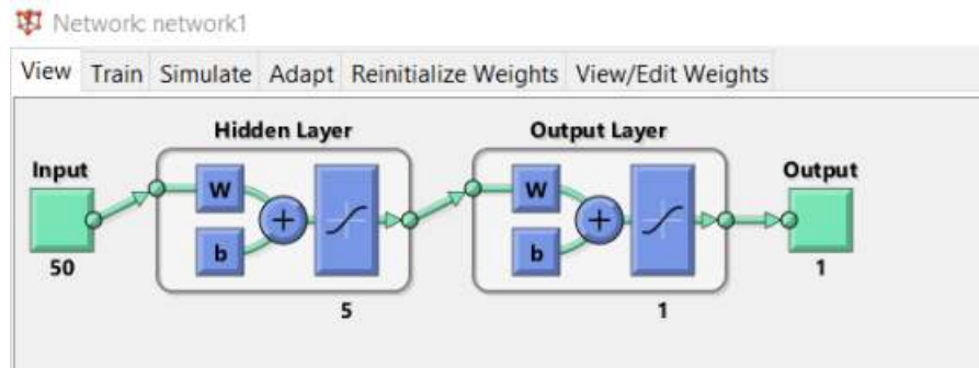
Şekil 4.22. Ağ mimarisi.
