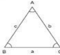
Şekil 2.5 Üçgende Alan Hesaplaması
