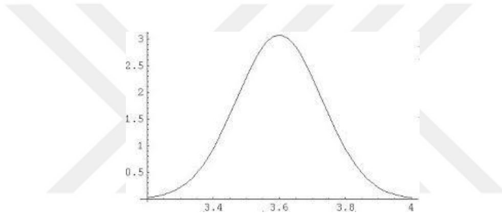
Şekil 2.1 Normal Dağılım Eğrisi
