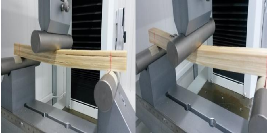
Şekil 2.14 : Elastikiyet modülü ve eğilme direncinin belirlenmesi
