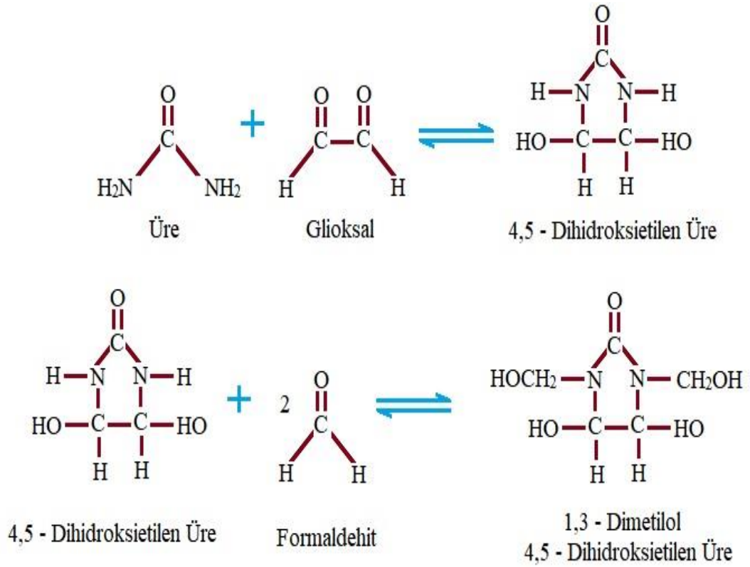
Şekil 1.5 : DMDHEU oluşumu [26].
