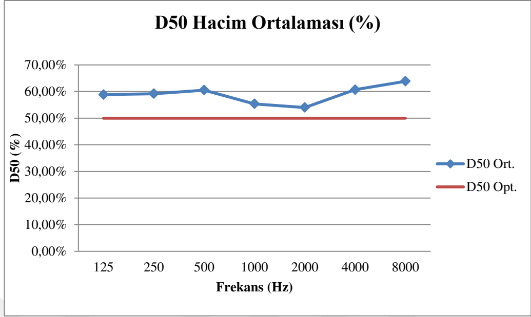
Şekil 4.95 Hacim genelinde ortalama D50 değerinin frekanslara göre değişimi.
