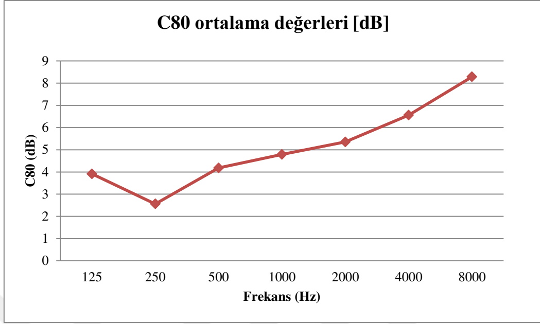
Şekil 4.54 Hacim genelinde netlik parametresinin frekanslara göre deęiřimi.
