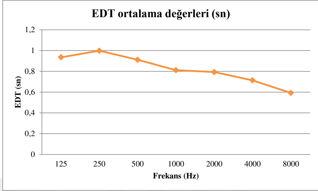
Şekil 4.52 Hacim genelinde EDT parametresinin frekanslara göre deęişimi.
