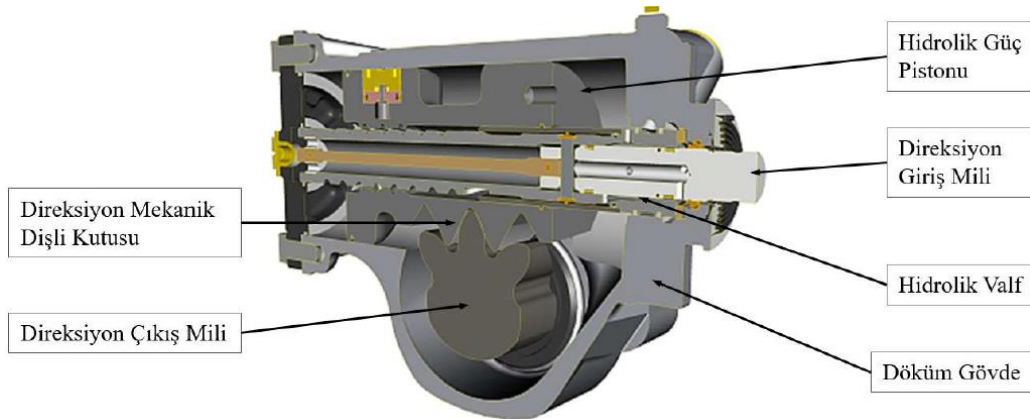
Şekil 3. 1. Direksiyon kutusu ve parçalarının görünümü (Uymaz, 2019)
