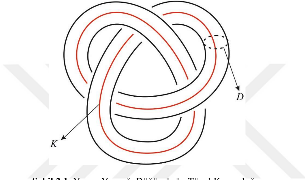
Şekil 2.1. Yonca Yaprığı Düğümünün Tünel Komşuluğu.
