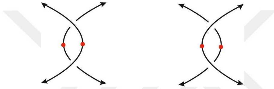
Şekil 4.17. Bir disoriented II. tip Reidemeister hareketi.
