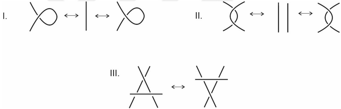
Şekil 2.3. Reidemeister hareketleri.
