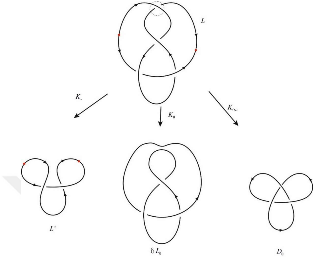
Şekil 4.6. İki disoriented kavşaklı sekiz şekilli düğümün bir ayrışımı.
