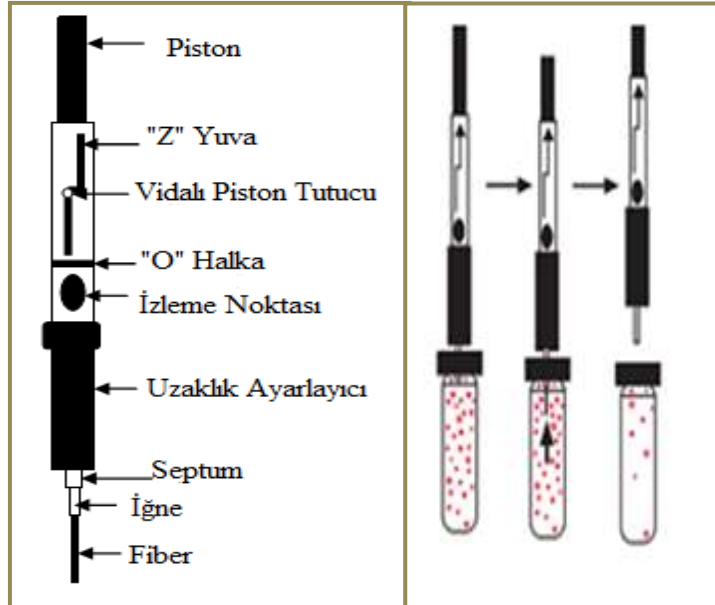
Şekil 2. Katı faz mikroekstraksiyon enjektörü ve sistemi
