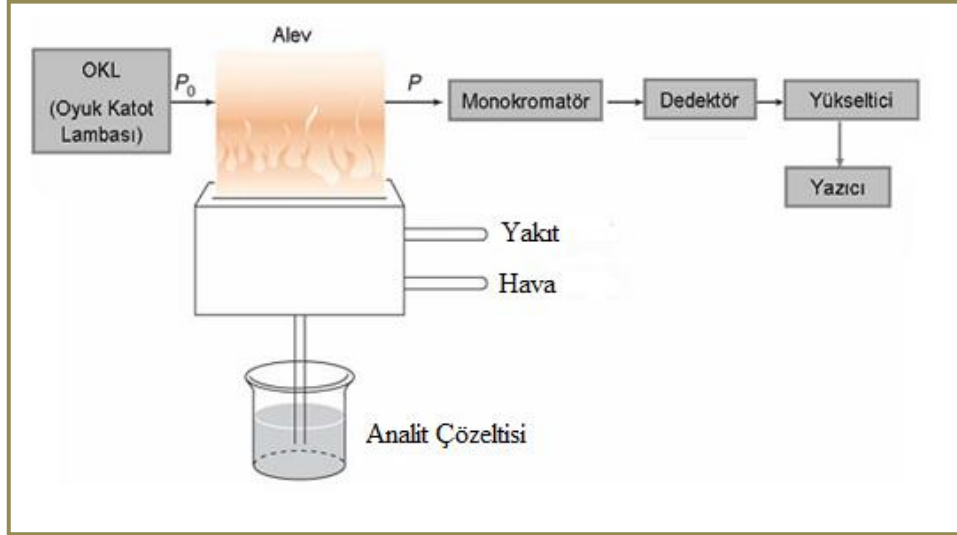
Şekil 9. Atomik absorpsiyon spektrometresi blok diyagramı
