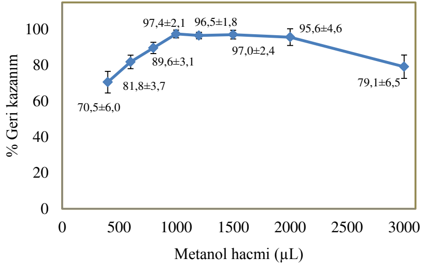
Şekil 48. \text{Au}^{3+} (0,5 µg) iyonlarının geri kazanımı üzerine metanol hacminin etkisi; 0,2 mol L -1 \text{HNO}_3 'li ortam, numune hacmi: 10 mL, L3 miktarı: 0,5 mg (% 0,4 (a/v), 125 µL), \text{CCl}_4 : 125 µL, bekleme süresi: 5 dk, santrifüj hızı: 3000 rpm, santrifüj süresi: 3 dk, N:3
