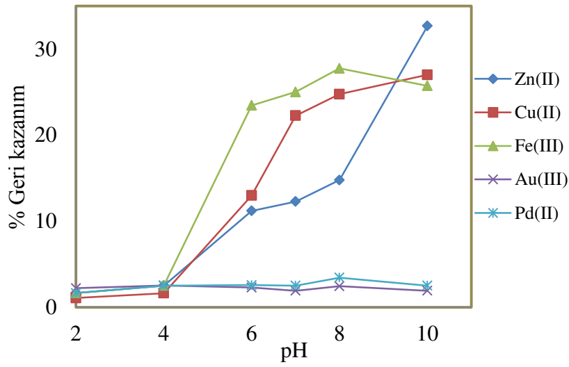
Şekil 26. L1 ile Zn^{2+} (0,1 \mu g ), Cu^{2+} (0,5 \mu g ), Fe^{3+} (0,5 \mu g ), Au^{3+} (0,5 \mu g ) ve Pd^{2+} (0,5 \mu g ) iyonlarının geri kazanımı üzerine pH etkisi; numune hacmi: 10 mL, L1 miktarı: 0,5 mg (% 0,4 (a/v), 125 \mu L ), CH_3OH : 1000 \mu L , CHCl_3 : 250 \mu L bekleme süresi: 5 dk, santrifüj hızı: 3000 rpm, santrifüj süresi: 3 dk, N:3
