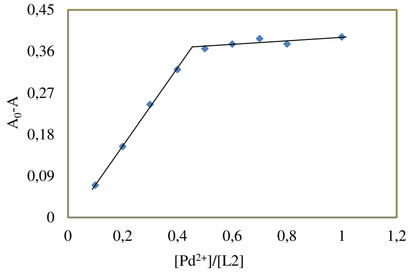
Şekil 22. L2- \text{Pd}^{2+} için mol oranlar grafiği, (380 nm)
