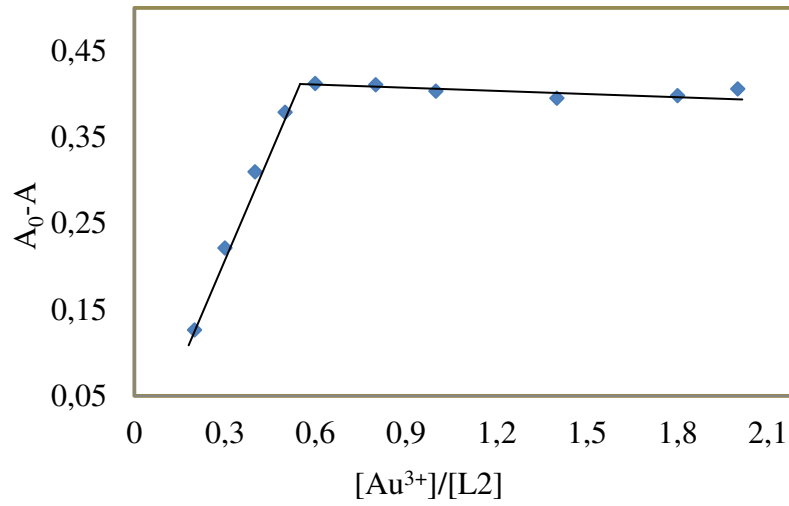
Şekil 20. L2-Au 3+ için mol oranlar grafiği, (380 nm)
