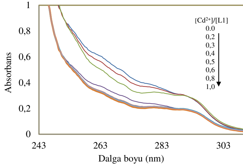
Şekil 17. 240-310 nm arasındaki L1 absorpsiyonu üzerine değişen \text{Cd}^{2+} konsantrasyonunun etkisi; [\text{L1}] : 6,0 \times 10^{-5} \text{ mol L}^{-1} , [\text{Cd}^{2+}] : 1,2 \times 10^{-5} - 6,0 \times 10^{-5} \text{ mol L}^{-1}
