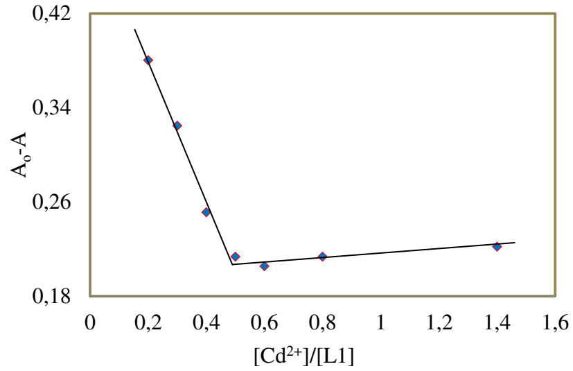
Şekil 18. L1- \text{Cd}^{2+} için mol oranlar grafiği, (275 nm)
