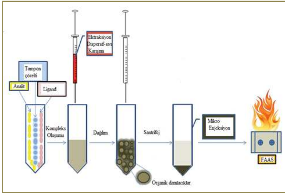
Şekil 6. Dispersif sıvı-sıvı mikroekstraksiyon sistemi
