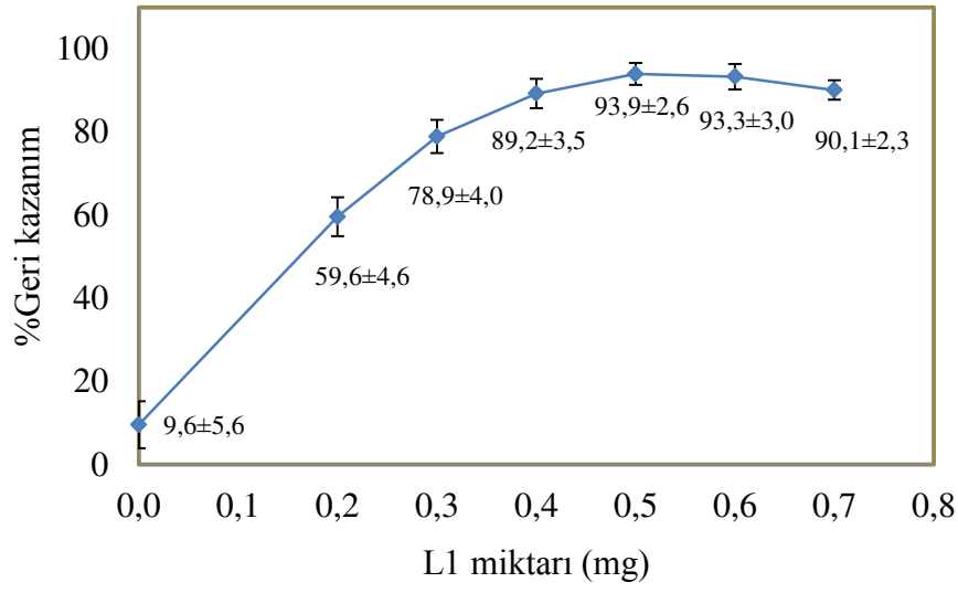
Şekil 37. \text{Cd}^{2+} ( 0,075 \mu\text{g} ) iyonlarının geri kazanımı üzerine L1 miktarının etkisi; pH=6,5, numune hacmi: 10 mL, \text{CH}_3\text{OH} : 1000 \mu\text{L} , \text{CHCl}_3 : 250 \mu\text{L} , bekleme süresi: 5 dk, santrifüj hızı: 3000 rpm, santrifüj süresi: 3 dk, N:3
