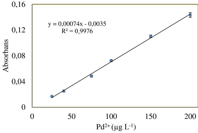
Şekil 57. L2 ile DSSME yöntemi uygulandıktan sonra 25-200 \mu\text{g L}^{-1} \text{Pd}^{2+} aralığında elde edilen kalibrasyon doğrusu; pH= 1,5, numune hacmi 10 mL, L2 miktarı: 0,5 mg, \text{C}_2\text{H}_5\text{OH} : 1200 \mu\text{L} , \text{CCl}_4 : 125 \mu\text{L} , bekleme süresi: 5 dk, santrifüj hızı: 3000 rpm, santrifüj süresi: 3 dk, N:3
