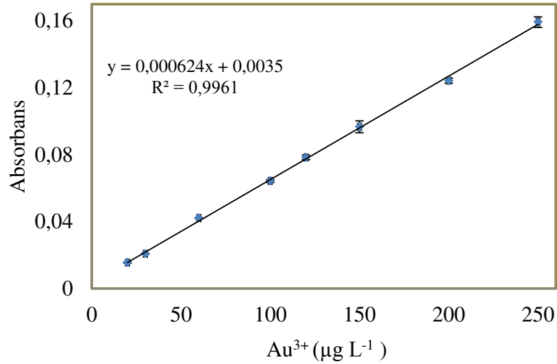
Şekil 58. L3 ile DSSME yöntemi uygulandıktan sonra 20-250 \mu\text{g L}^{-1} \text{Au}^{3+} aralığında elde edilen kalibrasyon doğrusu; 0,2 mol \text{L}^{-1} \text{HNO}_3 ortam, numune hacmi 10 mL, L3 miktarı: 0,5 mg, \text{CH}_3\text{OH} : 1000 \mu\text{L} , \text{CCl}_4 : 125 \mu\text{L} , bekleme süresi: 5 dk, santrifüj hızı: 3000 rpm, santrifüj süresi: 3 dk, N:3
