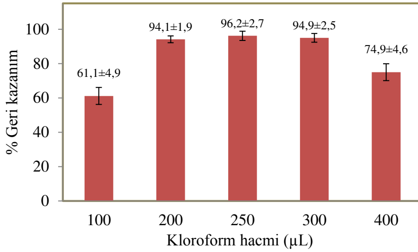
Şekil 49. \text{Cd}^{2+} (0,075 µg) iyonlarının geri kazanımı üzerine kloroform hacmi etkisi; pH=6,5, numune hacmi: 10 mL, L1 miktarı: 0,5 mg (% 0,4 (a/v), 125 µL), \text{CH}_3\text{OH} : 1000 µL, bekleme süresi: 5 dk, santrifüj hızı: 3000 rpm, santrifüj süresi: 3 dk, N:3
