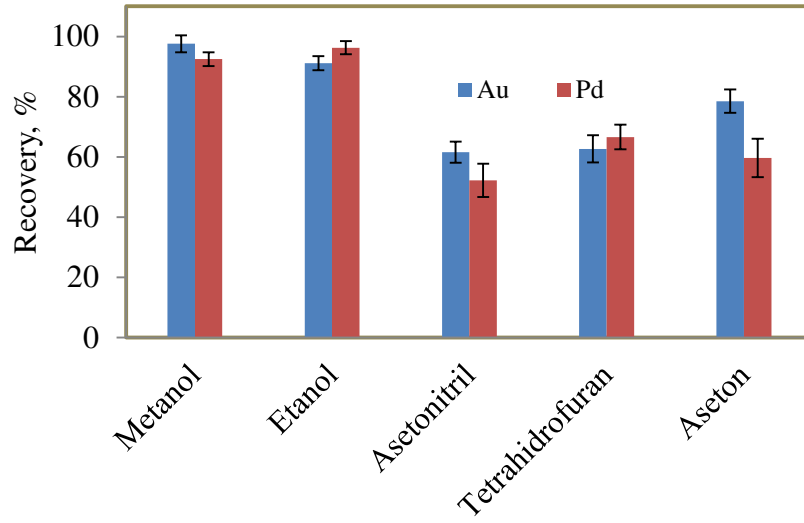
Şekil 42. \text{Au}^{3+} (0,5 \mu\text{g} ) ve \text{Pd}^{2+} (0,5 \mu\text{g} ) iyonlarının geri kazanımı üzerine dispersif sıvısı türü etkisi; \text{Au}^{3+} için pH=5,5, \text{Pd}^{2+} için pH= 1,5, numune hacmi: 10 mL, L2 miktarı: 0,5 mg (% 0,4 (a/v), 125 \mu\text{L} ), dispersif sıvı hacmi: 1200 \mu\text{L} , \text{CCl}_4 : 125 \mu\text{L} , bekleme süresi: 5 dk, santrifüj hızı: 3000 rpm, santrifüj süresi: 3 dk, N:3
