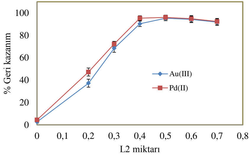
Şekil 38. \text{Au}^{3+} ( 0,5 \mu\text{g} ) ve \text{Pd}^{2+} ( 0,5 \mu\text{g} ) iyonlarının geri kazanımı üzerine L2 etkisi; \text{Au}^{3+} için \text{pH} = 5,5 , \text{Pd}^{2+} için \text{pH} = 1,5 , numune hacmi: 10 \text{ mL} , \text{Au}^{3+} için 1200 \mu\text{L} \text{CH}_3\text{OH} , \text{Pd}^{2+} için 1200 \mu\text{L} \text{C}_2\text{H}_5\text{OH} , \text{CCl}_4 : 125 \mu\text{L} , bekleme süresi: 5 \text{ dk} , santrifüj hızı: 3000 \text{ rpm} , santrifüj süresi: 3 \text{ dk} , N:3
