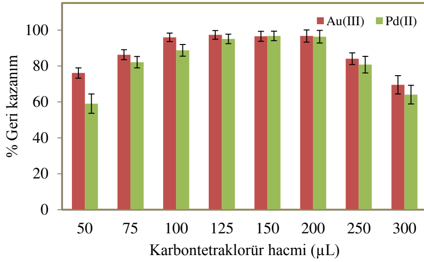
Şekil 50. \text{Au}^{3+} (0,5 µg) ve \text{Pd}^{2+} (0,5 µg) iyonlarının geri kazanımı üzerine karbondiklorür hacminin etkisi; \text{Au}^{3+} için pH=5,5, \text{Pd}^{2+} için pH=1,5, numune hacmi: 10 mL, L2 miktarı: 0,5 mg (% 0,4 (a/v), 125 µL), \text{Au}^{3+} için \text{CH}_3\text{OH} hacmi: 1200 µL, \text{Pd}^{2+} için \text{C}_2\text{H}_5\text{OH} hacmi: 1200 µL, bekleme süresi: 5 dk, santrifüj hızı: 3000 rpm, santrifüj süresi: 3 dk, N:3
