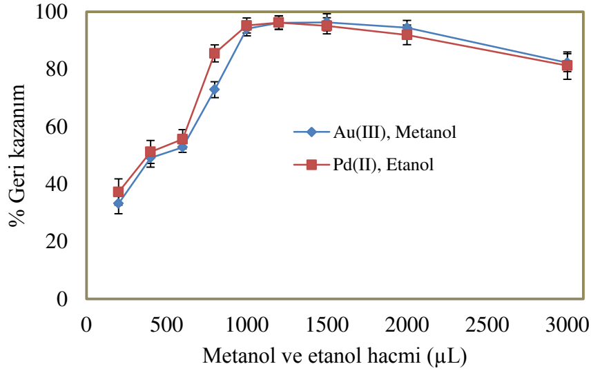
Şekil 47. \text{Au}^{3+} (0,5 µg) ve \text{Pd}^{2+} (0,5 µg) iyonlarının geri kazanımı üzerine metanol ve etanol hacminin etkisi; \text{Au}^{3+} için metanol, pH=5,5 \text{Pd}^{2+} için etanol, pH=1,5, numune hacmi: 10 mL L2 miktarı: 0,5 mg (% 0,4 (a/v), 125 µL), \text{CCl}_4 : 125 µL, bekleme süresi: 5 dk, santrifüj hızı: 3000 rpm, santrifüj süresi: 3 dk, N:3
