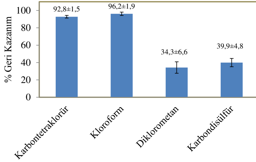
Şekil 41. \text{Cd}^{2+} (0,075 \mu\text{g} ) iyonlarının geri kazanımı üzerine ekstraksiyon sıvısı türünün etkisi; pH=6,5, numune hacmi: 10 mL, L1 miktarı: 0,5 mg (% 0,4 (a/v), 125 \mu\text{L} ), \text{CH}_3\text{OH} : 1000 \mu\text{L} , ekstraksiyon sıvısı: 250 \mu\text{L} , bekleme süresi: 5 dk, santrifüj hızı: 3000 rpm, santrifüj süresi: 3 dk, N:3
