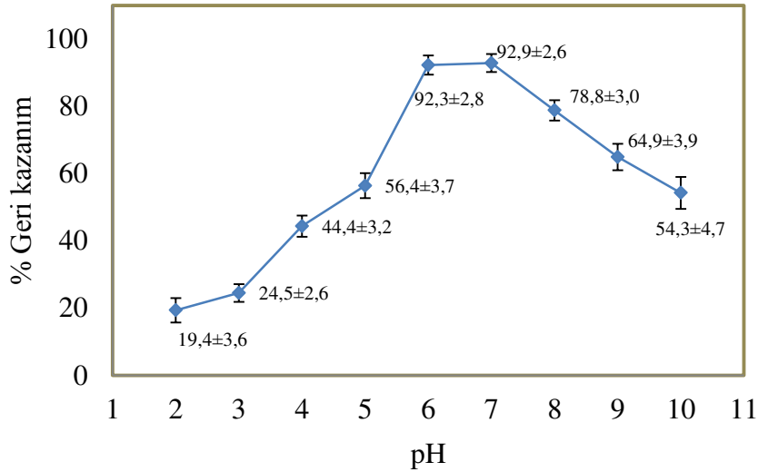
Şekil 27. L1 ile Cd^{2+} (0,075 \mu g ) iyonlarının geri kazanımı üzerine pH etkisi; numune hacmi: 10 mL, L1 miktarı: 0,5 mg (% 0,4 (a/v), 125 \mu L ), CH_3OH : 1000 \mu L , CHCl_3 : 250 \mu L bekleme süresi: 5 dk, santrifüj hızı: 3000 rpm, santrifüj süresi: 3 dk, N:3
