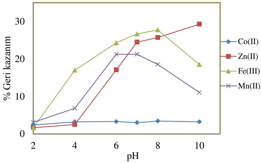
Şekil 33. L3 ile \text{Co}^{2+} (0,5 \mu\text{g} ), \text{Zn}^{2+} (0,1 \mu\text{g} ), \text{Fe}^{3+} (0,5 \mu\text{g} ) ve \text{Mn}^{2+} (0,1 \mu\text{g} ) iyonlarının geri kazanımı üzerine pH etkisi; numune hacmi: 10 mL, L3 miktarı: 0,5 mg (% 0,4 (a/v), 125 \mu\text{L} ), \text{CH}_3\text{OH} : 1000 \mu\text{L} , \text{CCl}_4 : 125 \mu\text{L} , bekleme süresi: 5 dk, santrifüj hızı: 3000 rpm, santrifüj süresi: 3 dk, N:3
