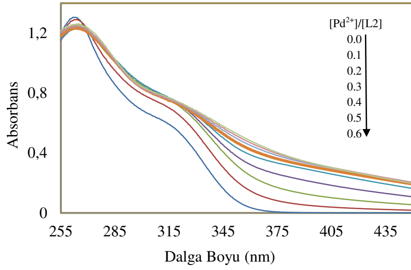
Şekil 21. 240-440 nm arasındaki L2 absorpsiyonu üzerine değişen \text{Pd}^{2+} konsantrasyonunun etkisi; [\text{L2}] : 5 \times 10^{-6} \text{ mol L}^{-1} , [\text{Pd}^{2+}] : 5,0 \times 10^{-7} – 4,0 \times 10^{-6} \text{ mol L}^{-1}
