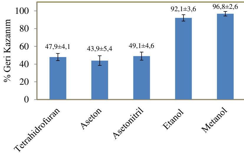
Şekil 40. \text{Cd}^{2+} ( 0,075\mu\text{g} ) iyonlarının geri kazanımı üzerine dispersif sıvı türünün etkisi; pH=6,5, numune hacmi: 10 mL, L1 miktarı: 0,5 mg (% 0,4 (a/v), 125 \mu\text{L} ), dispersif sıvı: 1000 \mu\text{L} , \text{CHCl}_3 : 250 \mu\text{L} , bekleme süresi: 5 dk, santrifüj hızı: 3000 rpm, santrifüj süresi: 3 dk, N:3
