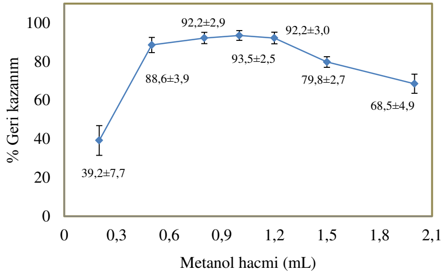
Şekil 46. \text{Cd}^{2+} ( 0,075 \mu\text{g} ) iyonlarının geri kazanımı üzerine metanol hacminin etkisi; \text{pH}=6,5 , numune hacmi: 10 mL, L1 miktarı: 0,5 mg (% 0,4 (a/v), 125 \mu\text{L} ), 250 \mu\text{L} \text{CHCl}_3 bekleme süresi: 5 dk, santrifüj hızı: 3000 rpm, santrifüj süresi: 3 dk, N:3
