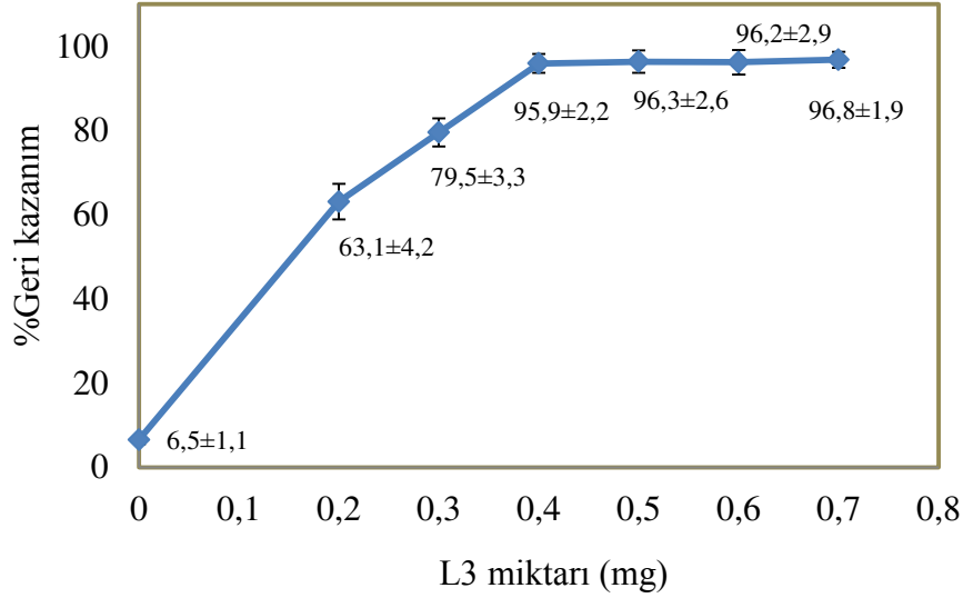
Şekil 39. \text{Au}^{3+} ( 0,5 \mu\text{g} ) iyonlarının geri kazanımı üzerine L3 miktarının etkisi; 0,2 \text{ mol L}^{-1} \text{HNO}_3 ortam, numune hacmi: 10 \text{ mL} , \text{CH}_3\text{OH} : 1000 \mu\text{L} , \text{CCl}_4 : 125 \mu\text{L} , bekleme süresi: 5 \text{ dk} , santrifüj hızı: 3000 \text{ rpm} , santrifüj süresi: 3 \text{ dk} , N:3
