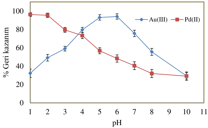
Şekil 30. L2 ile \text{Au}^{3+} (0,5 \mu\text{g} ) ve \text{Pd}^{2+} (0,5 \mu\text{g} ) iyonlarının geri kazanımı üzerine pH etkisi; numune hacmi: 10 mL, L2 miktarı: 0,5 mg (% 0,4 (a/v), 125 \mu\text{L} ), \text{Au}^{3+} için 1200 \mu\text{L} \text{CH}_3\text{OH} , \text{Pd}^{2+} için 1200 \mu\text{L} \text{C}_2\text{H}_5\text{OH} , 125 \mu\text{L} \text{CCl}_4 , bekleme süresi: 5 dk, santrifüj hızı: 3000 rpm, santrifüj süresi: 3 dk, N:3
