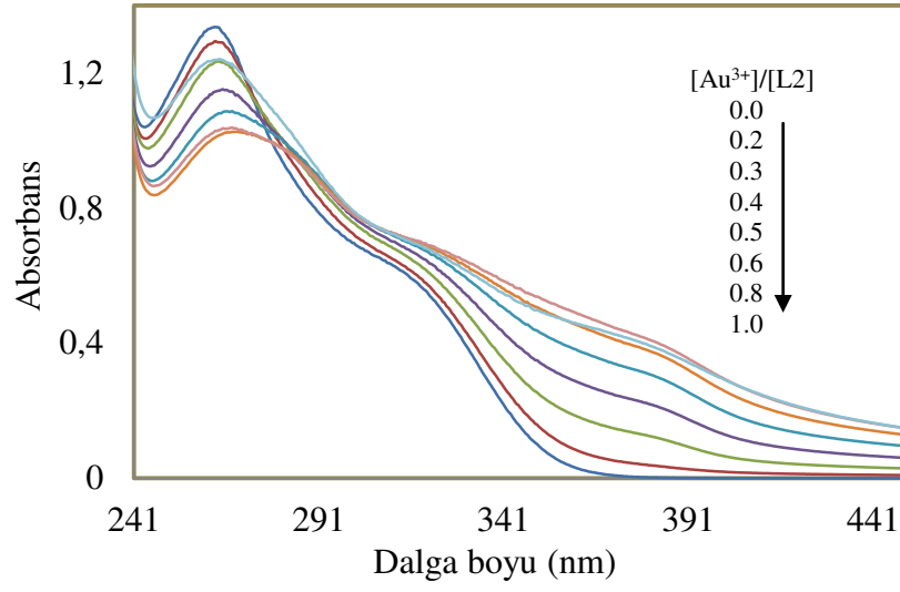
Şekil 19. 240-440 nm arasındaki L2 absorpsiyonu üzerine değişen Au 3+ konsantrasyonunun etkisi; [L2]: 5,0 \times 10^{-6} mol L -1 , [Au 3+ ]: 1,0 \times 10^{-6} – 1,0 \times 10^{-5} mol L -1
