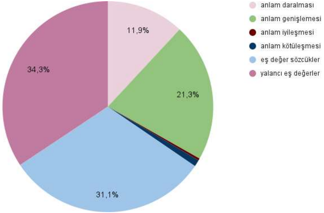
Şekil 4.3. Anlam olayları
