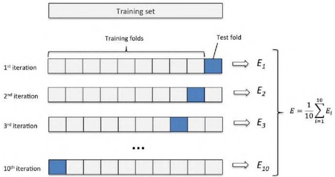
Şekil 4.8 Çapraz doğrulama (Rosaen 2016)
