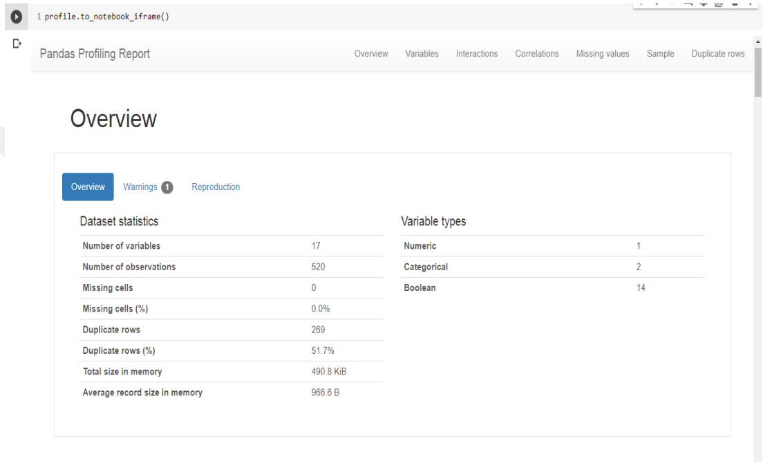
Şekil 4.7 Profil Reports
