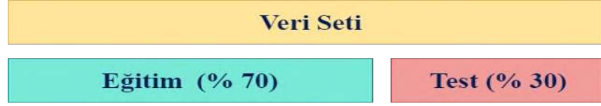
Şekil 4.9 Hold-out diyagramı
