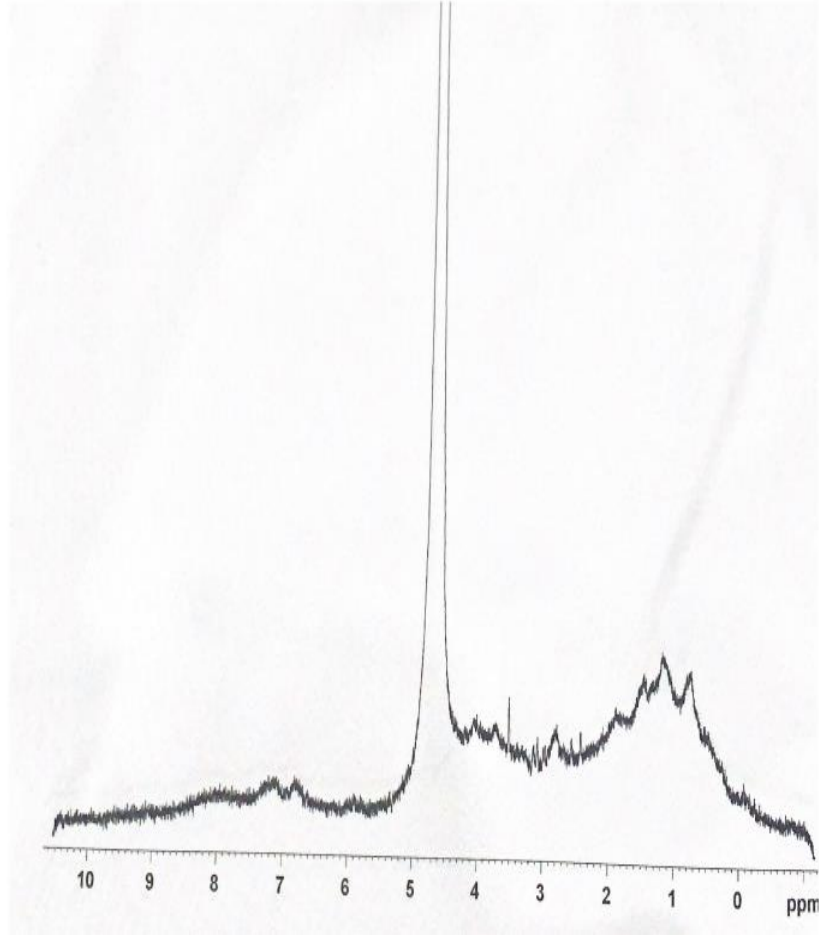
řekil 4.1. D 2 O ile hazırlanan diyabetli kan örneğinin 400 MHz NMR spektrumu
