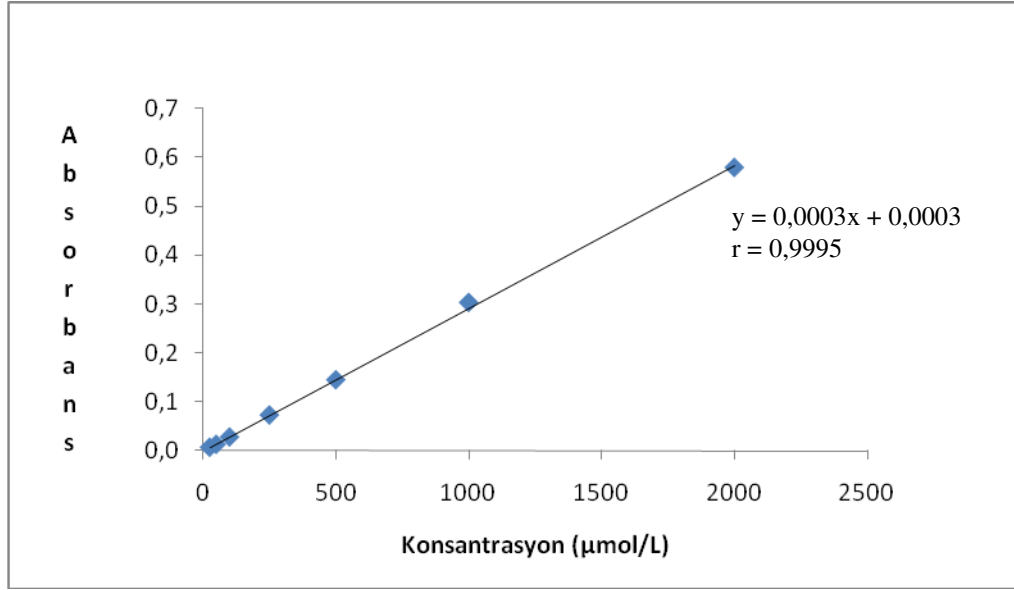
Şekil 6. Total tiyol grupları (TSH) kalibrasyon grafiği
