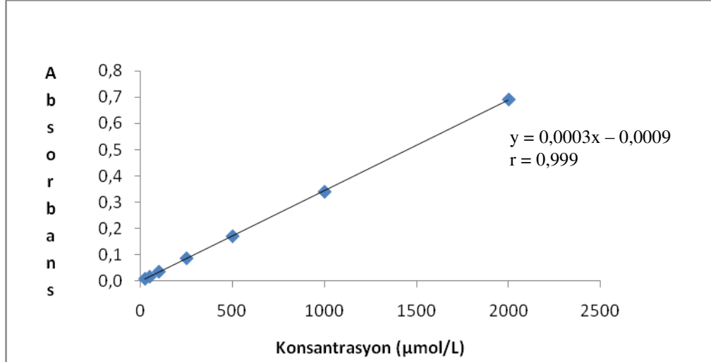
Şekil 5: Hücresel glutatyon (GSH) kalibrasyon grafiği.
