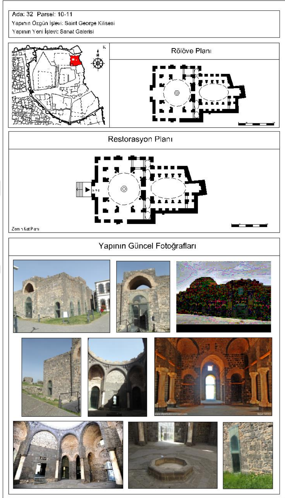
Şekil 4.40. Sanat Galerisi (Saint George Kilisesi) Bina Şeması
