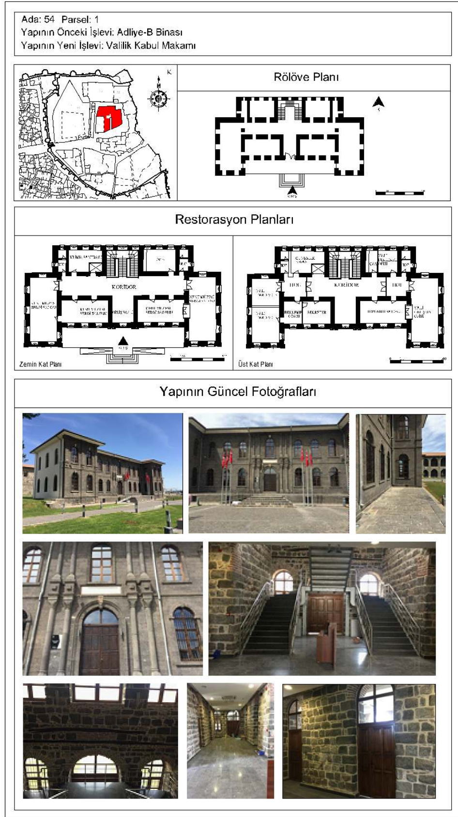
Şekil 4.42. Valilik Kabul Makamı ve Kent Müzesi Sergi Salonu (Adliye B Binası) Bina Şeması
