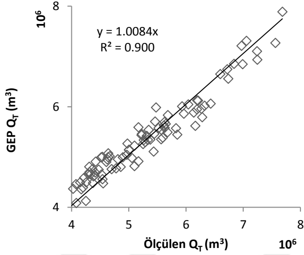
Şekil 4.3. Eğitim seti için tahmin edilen değerlerin ölçülen değerlerle karşılaştırılması
