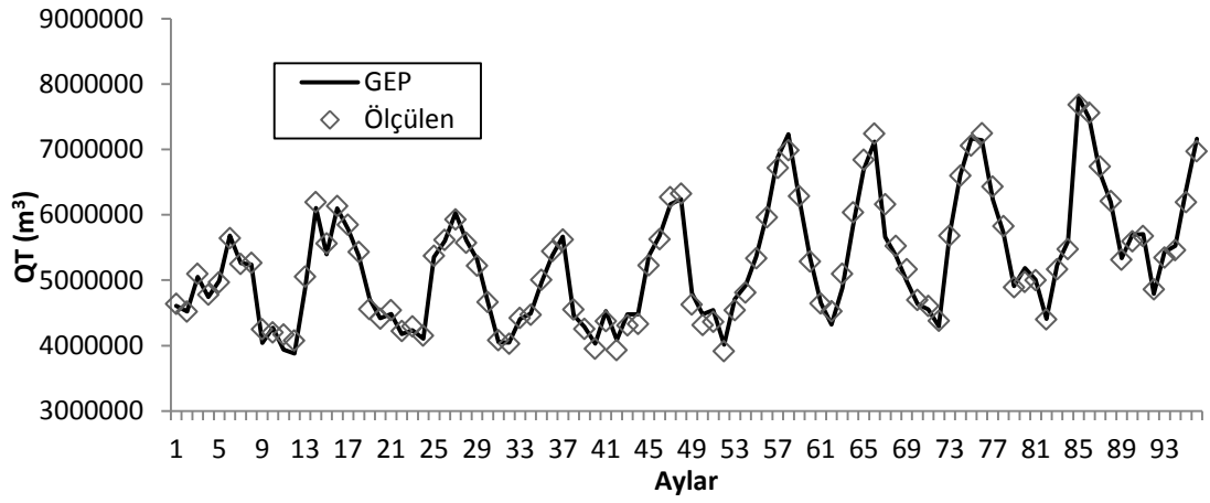
Şekil 4.12. GEP Model 3'ün eğitim aşamasındaki model değerleri ile gerçek değerlerin karşılaştırılması
