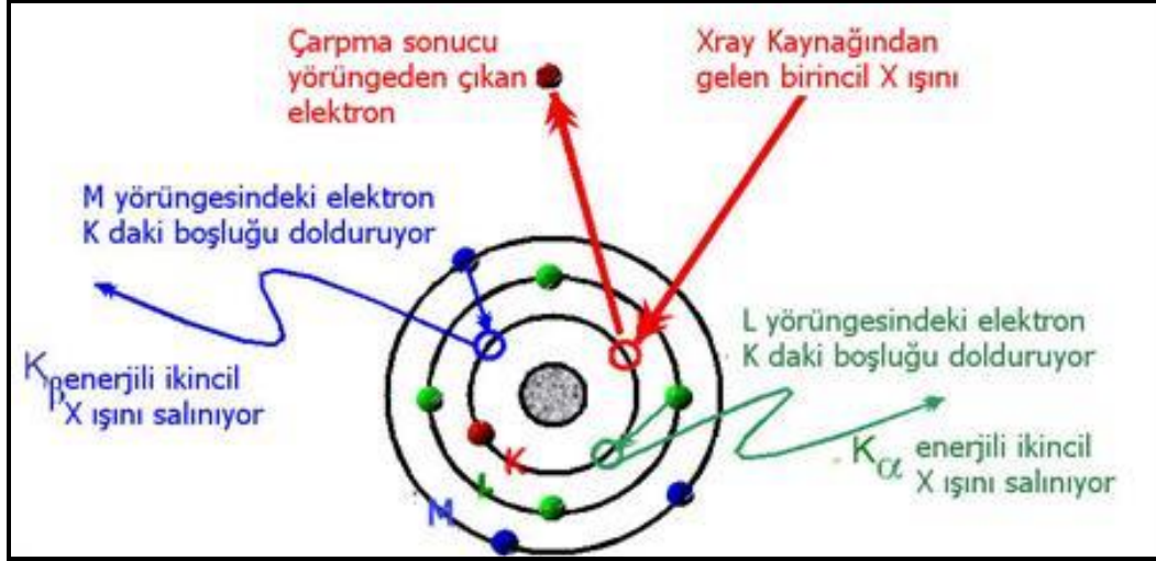
Şekil 3-2: XRF çalışma mekanizması (Aydın, 2017).
