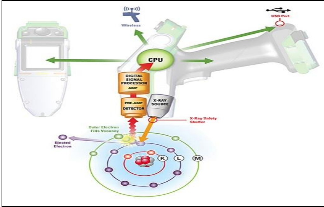
Şekil 3-4: XRF cihazında örnek analizi gösterimi (Aydın, 2017).
