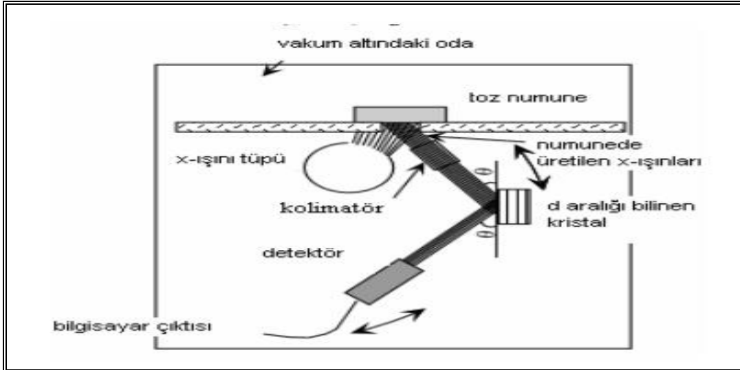
Şekil 3-10:WD-XRF Spektroskopisinin çalışma diyagramı (Arkalı, 2010)
