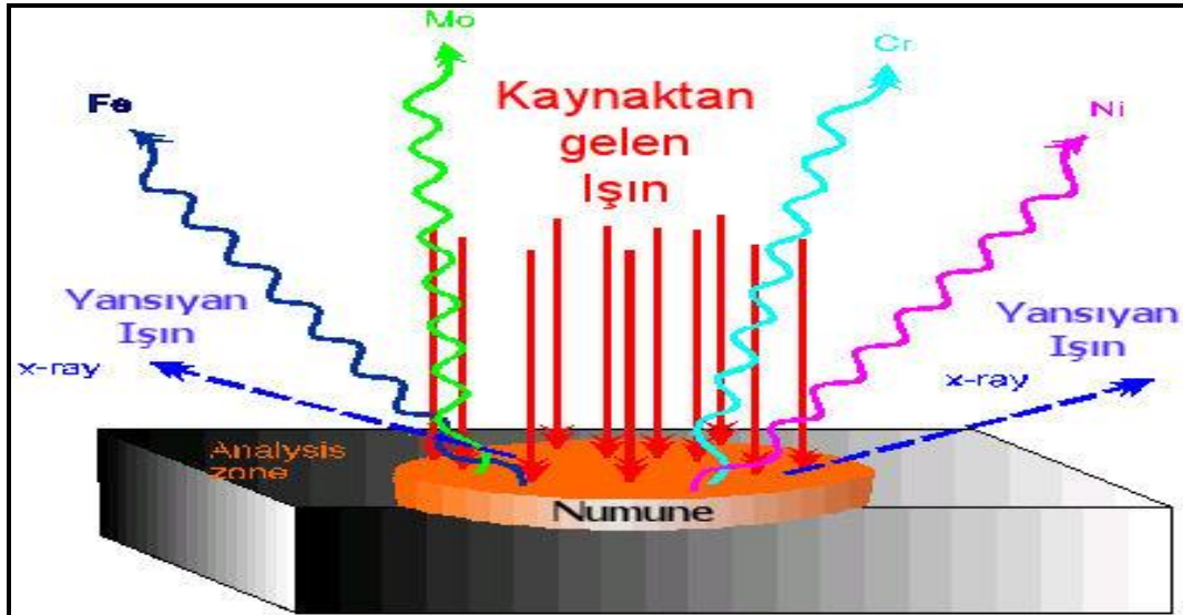
Şekil 3-3: XFR alaşım tespiti gösterimi (Aydın, 2017).
