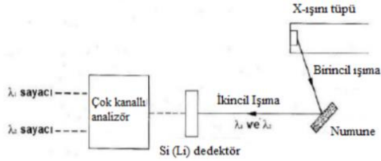
Şekil 3. 2. ED-XRF Spektrometresinin şematik görünümü (Küçük ve ark, 2017).
