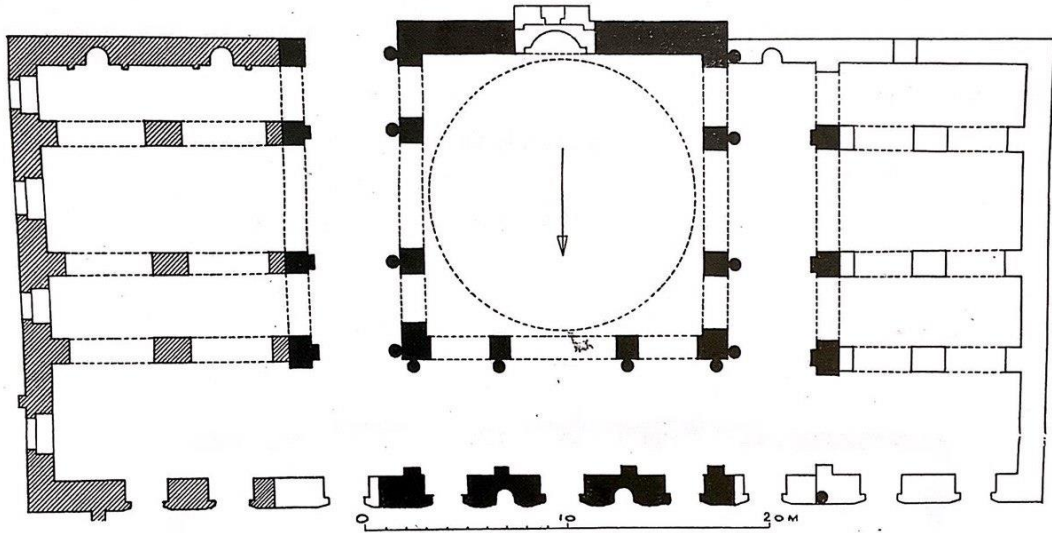
Şekil 10. Silvan Ulu Camii Planı 715
