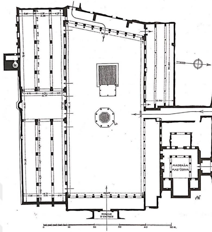
Şekil 7. Ulu Cami Planı. 712
