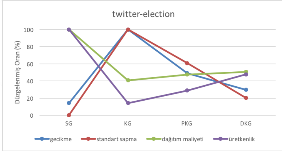
Şekil 20. twitter-election performans karşılaştırması
