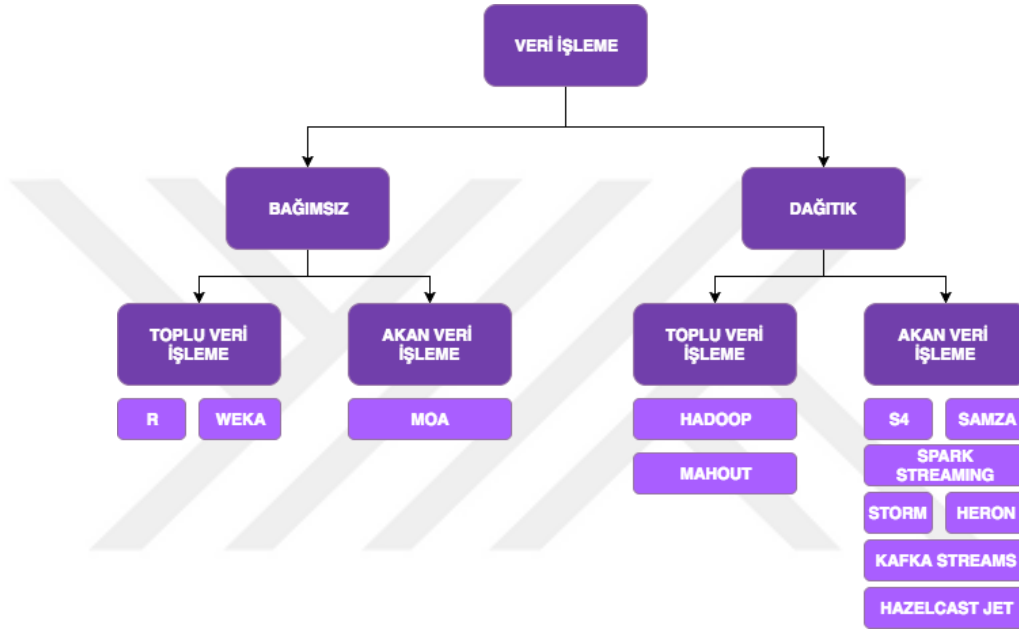
Şekil 2. Veri İşleme Uygulamaları
