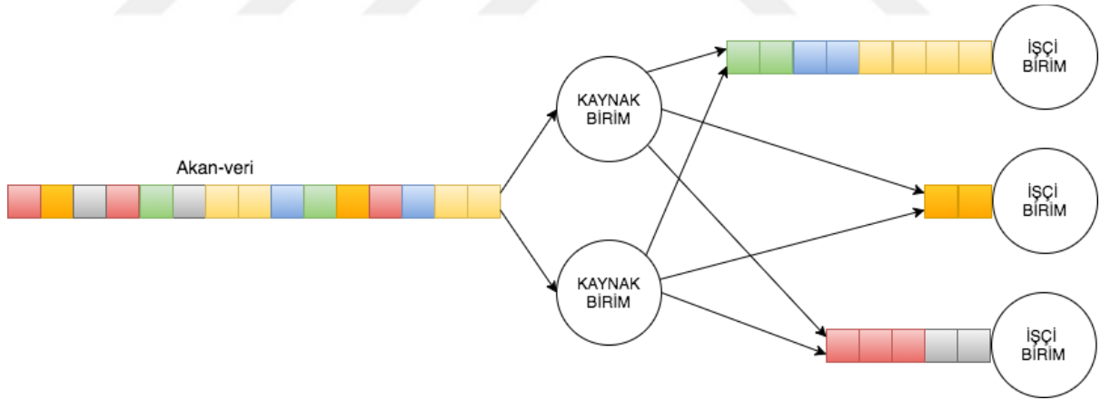
Şekil 14. Yükün Dengesiz Dağıtımı [26]
