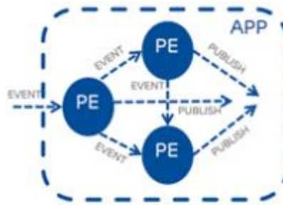
Şekil 4. S4 Mimarisi [4]
