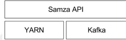
Şekil 3. Samza Mimarisi [3]
