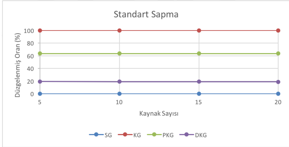
Şekil 55. Standart Sapma değerlerinin Kaynak Birim sayılarına göre değişimi
