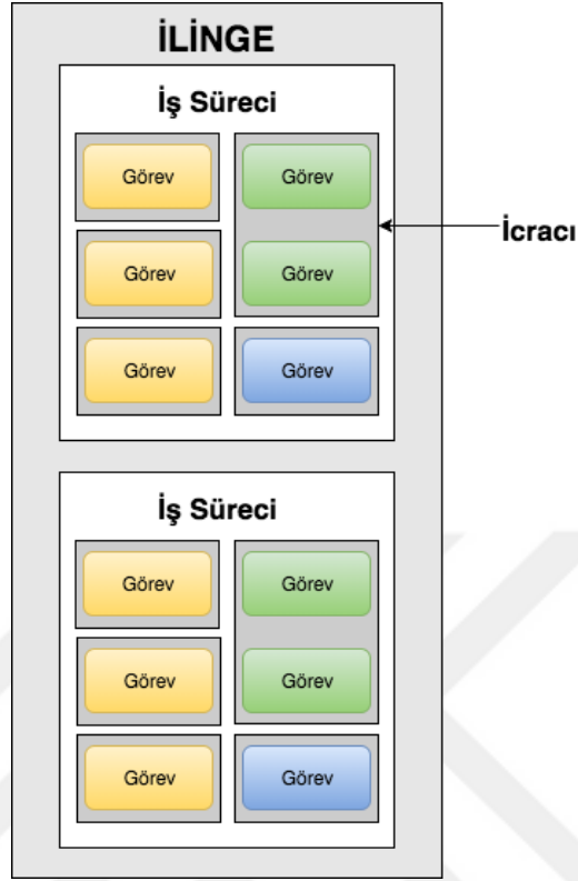
Şekil 13. Storm İlingesi [15]
