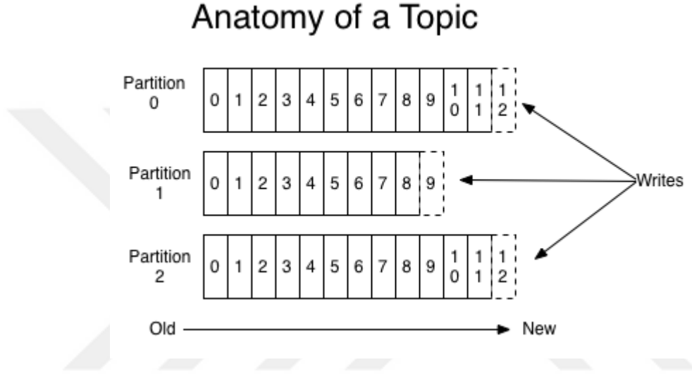
Şekil 18. Kafka mimarisi [8]
