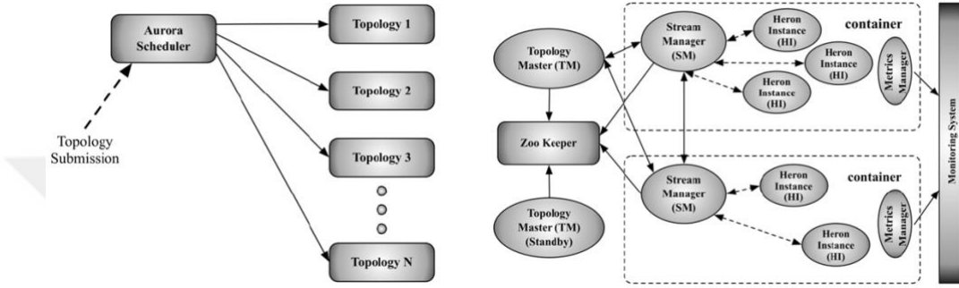
Şekil 7. Heron Mimarisi [7]
