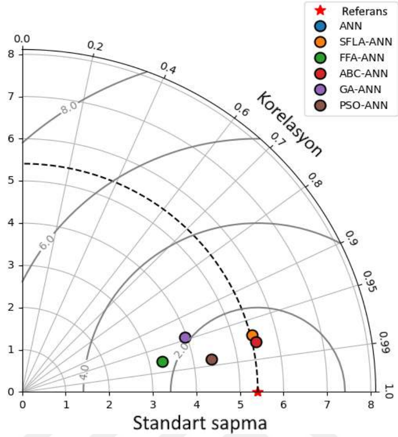
Şekil 25. Taylor diyagramı ile taşkın tahmin modellerinin karşılaştırılması
