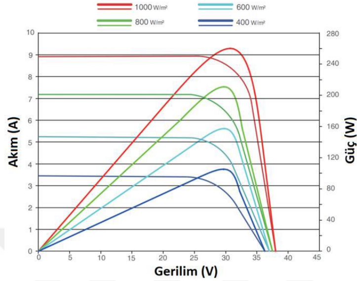
Şekil 3.6. PV panellerin ışıma bağlı akım, gerilim, güç değişim değerleri [51].
