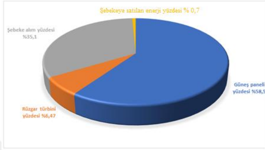
Şekil 4.17. Simülasyon-1 için güneş radyasyonu ortalaması 7,8 kWh/m 2 /gün ve rüzgâr hızı ortalaması 4,56 m/s olan simülasyonun analizine bağlı elektrik üretim kaynakları sonucu.
