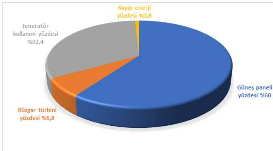
Şekil 4.21. Simülasyon-2 için güneş radyasyonu ortalaması 7,8 kWh/m 2 /gün ve rüzgâr hızı ortalaması 4,56 m/s olan simülasyon analizine bağlı elektrik üretim kaynakları sonucu
