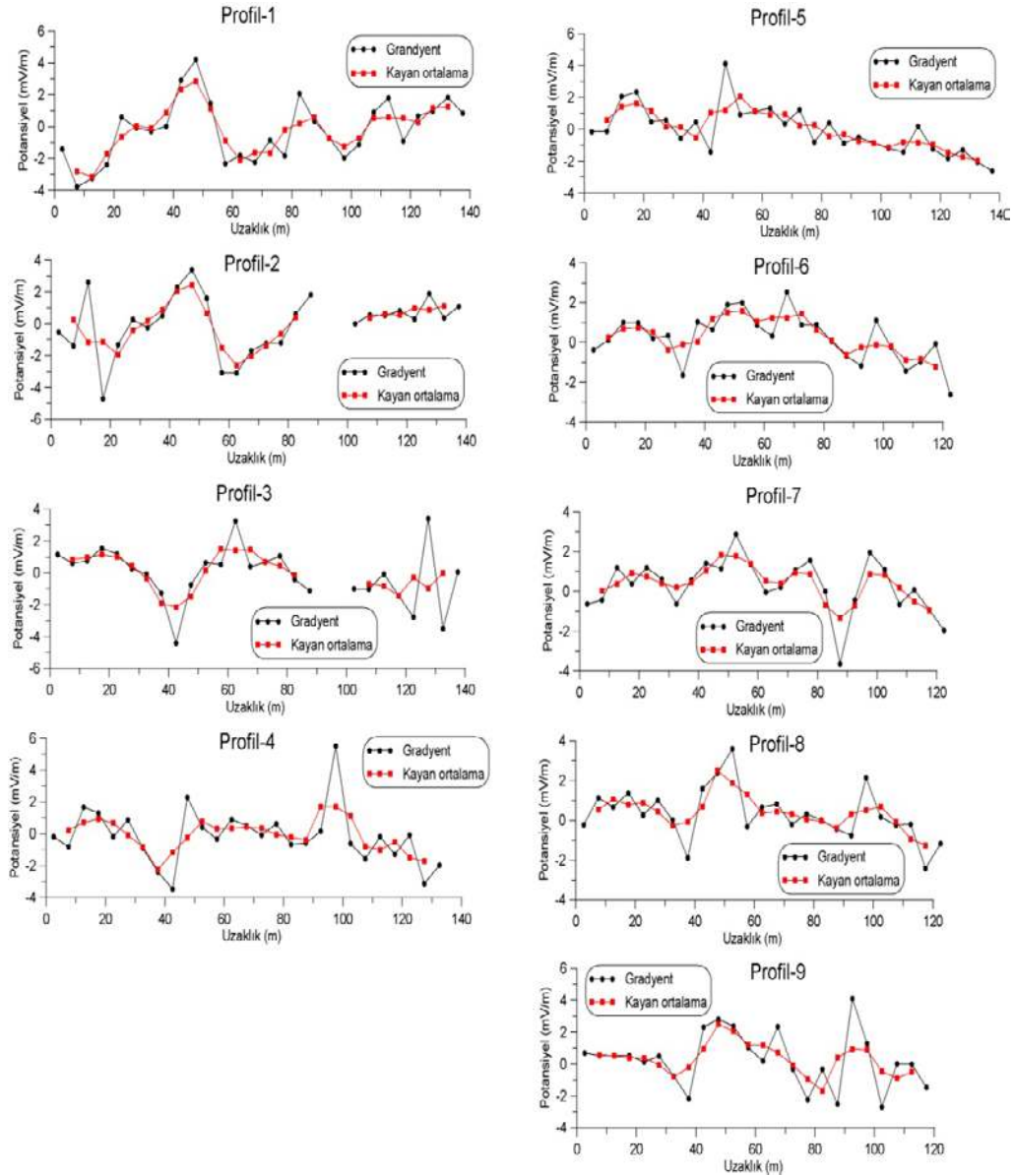
Şekil 5.6 İcmeler bölgesi doğal potansiyel yöntemi ile gradyent ölçümlerinden elde edilen grafikler.
