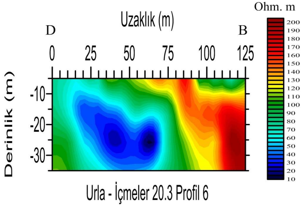
Şekil 5.40 İmeler bölgesi 20,3 kHz 6. profil EM-VLF sonuçları.
