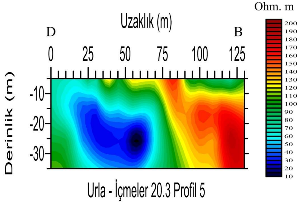
Şekil 5.39 İmeler bölgesi 20,3 kHz 5. profil EM-VLF sonuçları.
