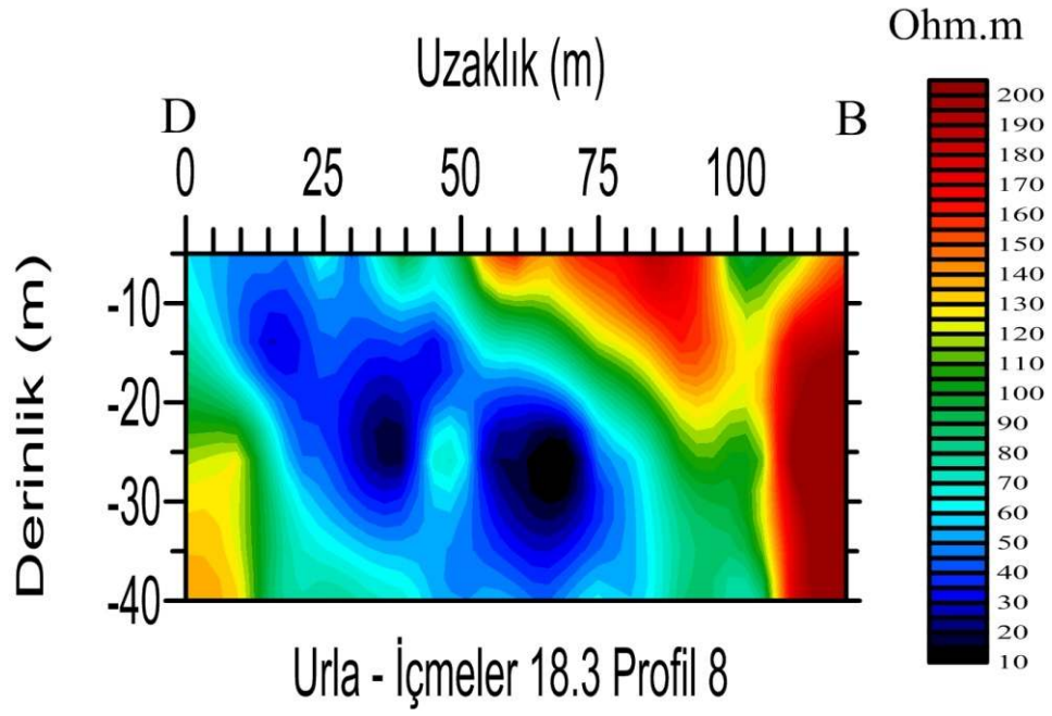
Şekil 5.33 İçmeler bölgesi 18,3kHz 8. profil EM-VLF sonuçları.
