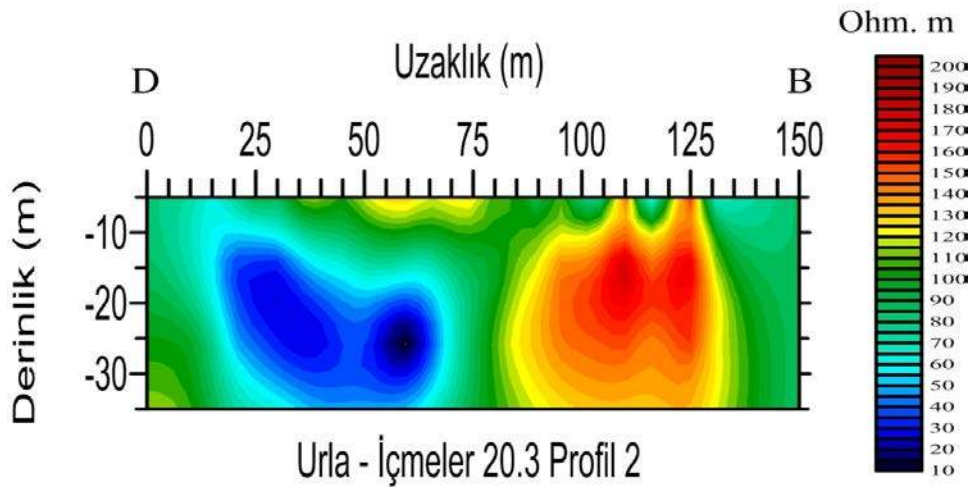
Şekil 5.36 İmeler bölgesi 20,3 kHz 2. profil EM-VLF sonuçları.
