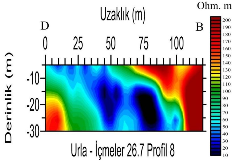
Şekil 5.51 İçmeler bölgesi 26,7 kHz 8. profil EM-VLF sonuçları.
