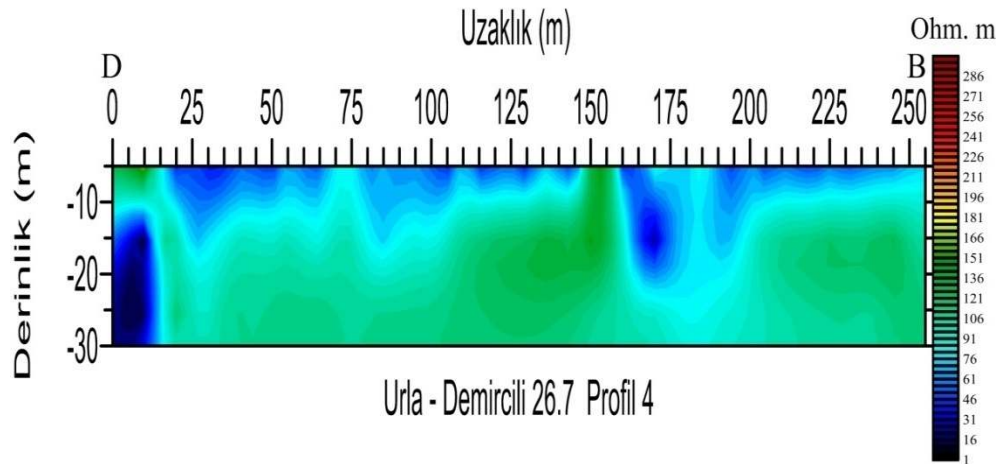
Şekil 5.64 Demircili bölgesi 26,7 kHz 4. profil EM-VLF sonuçları
