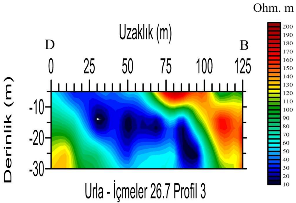
Şekil 5.46 İçmeler bölgesi 26,7 kHz 3. profil EM-VLF sonuçları.
