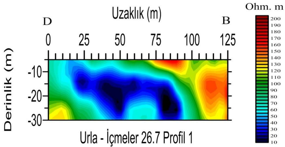
Şekil 5.44 İçmeler bölgesi 26,7 kHz 1. profil EM-VLF sonuçları.
