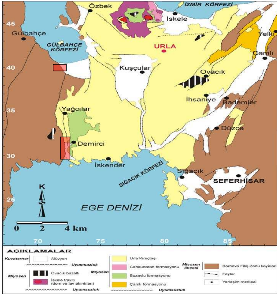
Şekil 4.1 Urla çevresinin temel kayalarını gösteren jeoloji haritası (İnci ve Sözbilir, 2004). Çalışma alanları kırmızı dikdörtgenler ile belirtilmiştir.
