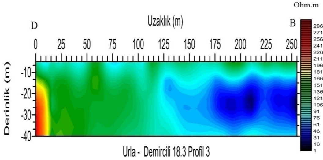
Şekil 5.55 Demircili bölgesi 18,3 kHz 3. profil EM-VLF sonuçları
