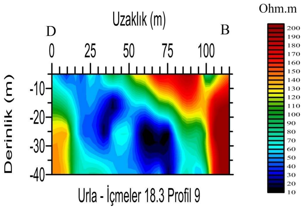
Şekil 5.34 İçmeler bölgesi 18,3kHz 9. profil EM-VLF sonuçları.
