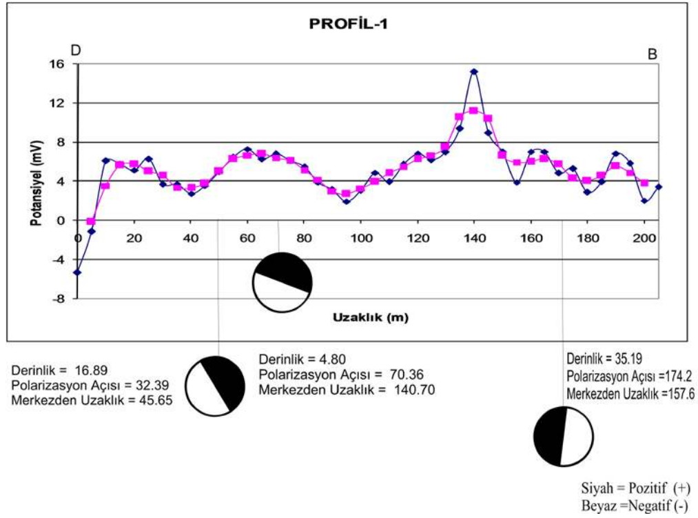
Şekil 5.22 Demircili bölgesi 1. profil doğal potansiyel ters-çözüm sonuçları.
