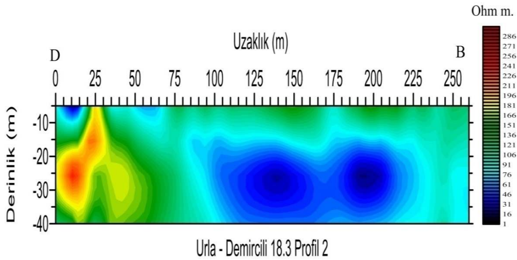
Şekil 5.54 Demircili bölgesi 18,3 kHz 2. profil EM-VLF sonuçları
