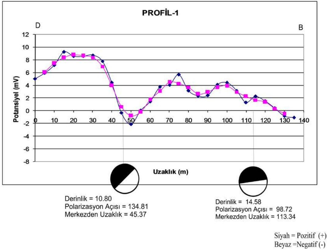
Şekil 5.14 İçmeler bölgesi 1. profil doğal potansiyel ters-çözüm sonuçları.
