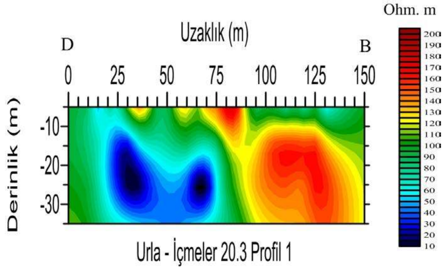
Şekil 5.35 İmeler bölgesi 20,3 kHz 1. profil EM-VLF sonuçları.
