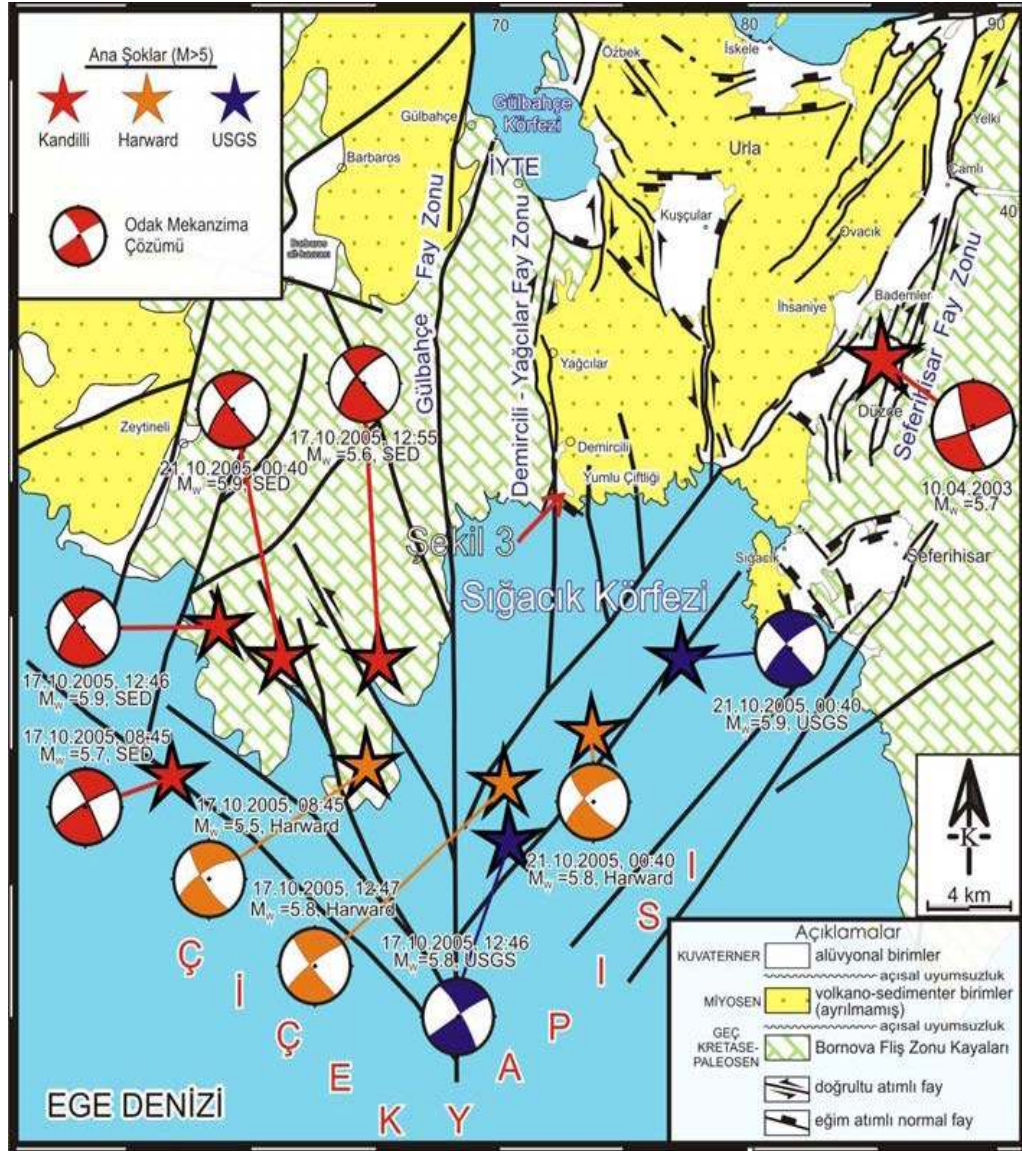
Şekil 4.4 Ekim-2005 ve Nisan-2003 depremlerinin ana şoklar harita üzerinde gösterilmiştir (Sözbilir vd. 2009).
