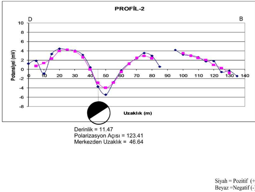
Şekil 5.15 İçmeler bölgesi 2. profil doğal potansiyel ters-çözüm sonuçları.
