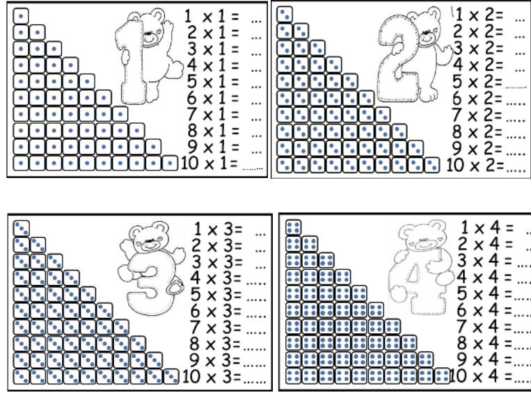
Şekil 9. Çarpım tablosunun toplama işlemi ile modellenmesi
