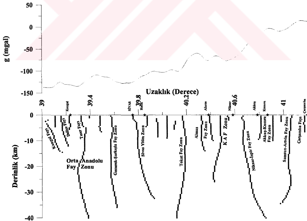
Şekil 26. 37^\circ boylamı üzerinde alınan BB’ gravite anomalisi profiline (Şekil 12) alçak geçişli süzgeç anomalilerinin tam yatay türevleri alınarak oluşturulan iki boyutlu kırık yapısı
