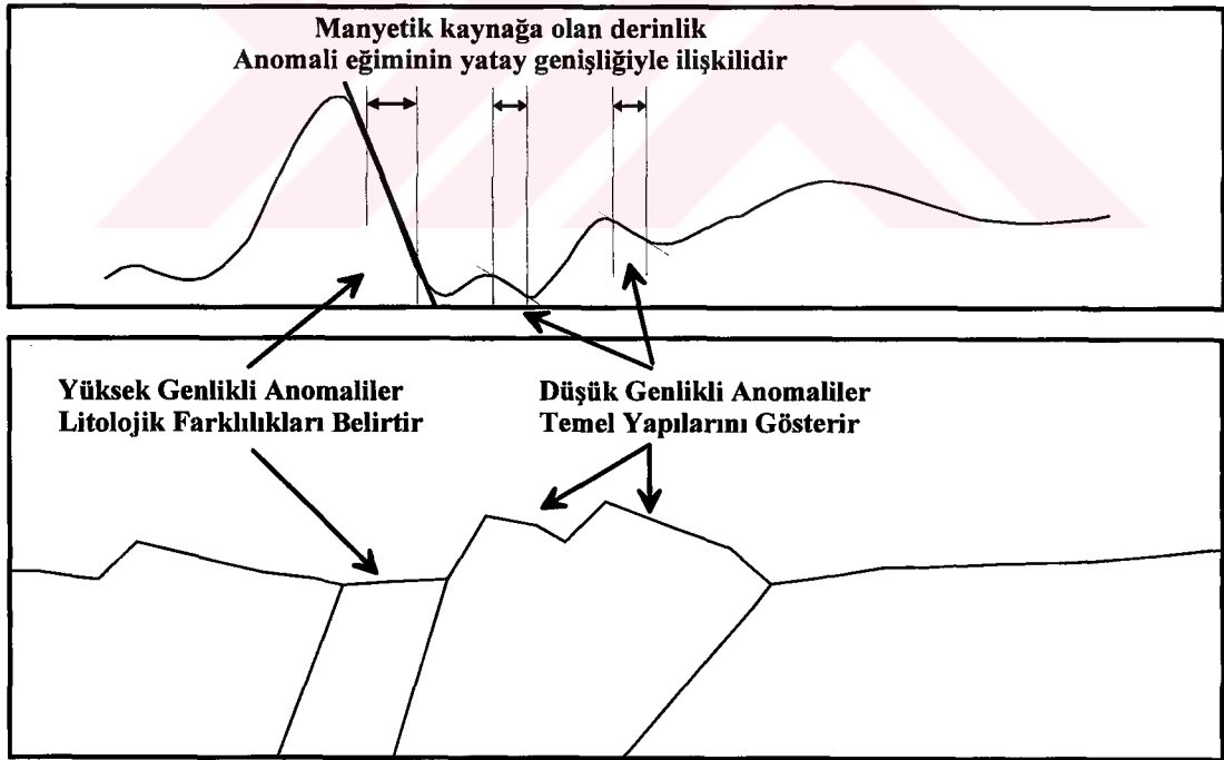
Şekil 1. Bir profil boyunca alınmış manyetik anomali değerlerinin litolojik değişim ve temelle olan ilişkileri (Bird, 1997).
