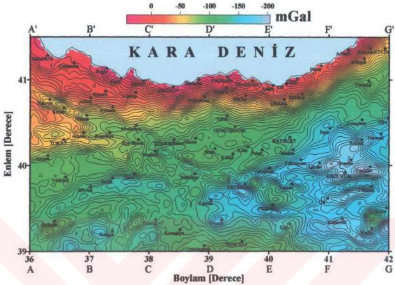
Şekil 6. Doğu Pontidlerin Bouguer Gravite anomali haritası. Kontur aralığı 5 mGal'dir
