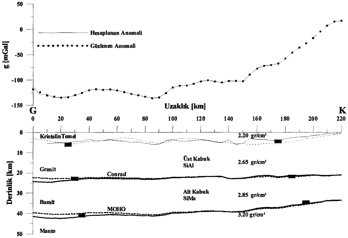
Şekil 73. Ters çözüm sonucu 38^\circ boylamına ait CC' gravite anomali profili (Şekil 6) altındaki iki boyutlu kabuk yapısı. Kesikli çizgiler başlangıç modelini, sürekli çizgiler ters çözüm sonucu elde edilen kabuk modelini, içi dolu dikdörtgenler güç spektrumu ile hesaplanan derinlikleri göstermektedir
