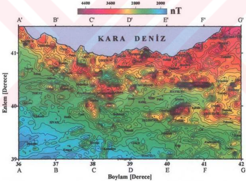
Şekil 7. Doğu Pontidlerin kutba indirgenmiş Manyetik anomali haritası. Kontur aralığı 100 nT'dır
