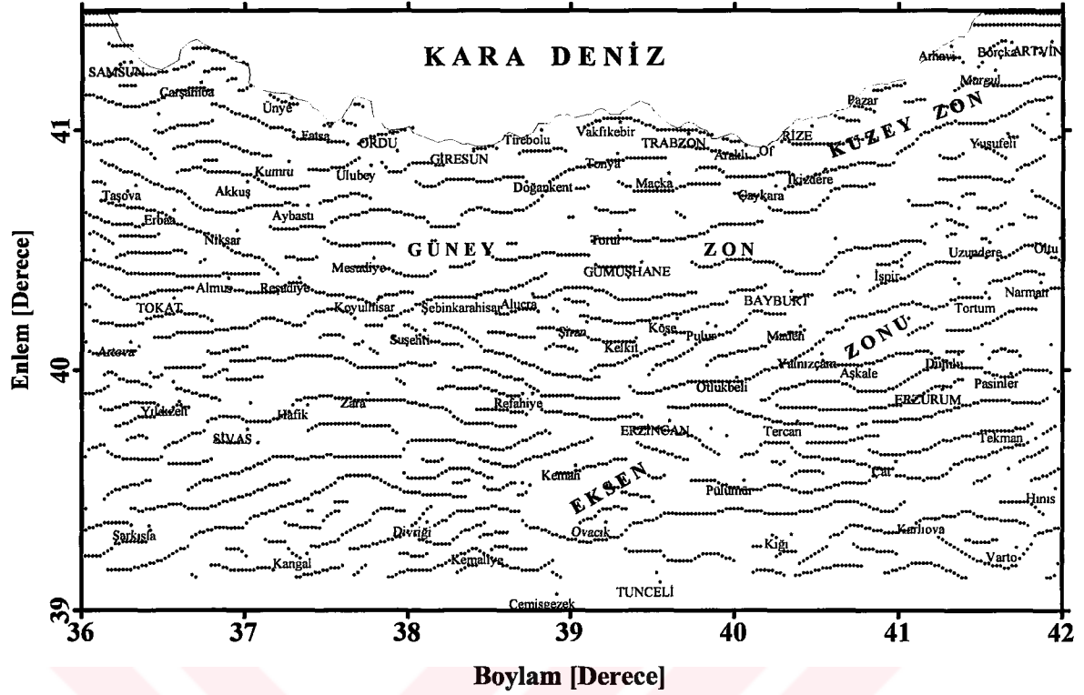
Şekil 13. Gravite anomali haritasına 20 km dalga boyu alçak geçişli süzgeç uygulanarak elde edilmiş tam yatay türev çizgisellik haritası
