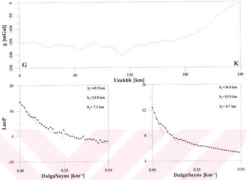
Şekil 54. 41^\circ boylamı üzerindeki FF' profiline (Şekil 6) ait gravite anomali değerleri ve bu profilin iki eşit parçaya bölünerek elde edilen güç spektrumu eğrileri. Güç spektrumu grafiklerinde görülen rakamlar kabuğa ait derinlik değerleri olup h_1 , Moho derinliğini; h_2 , Conrad süreksizliğinin derinliğini ve h_3 , Kristalin Temel derinliğini belirtmektedir
