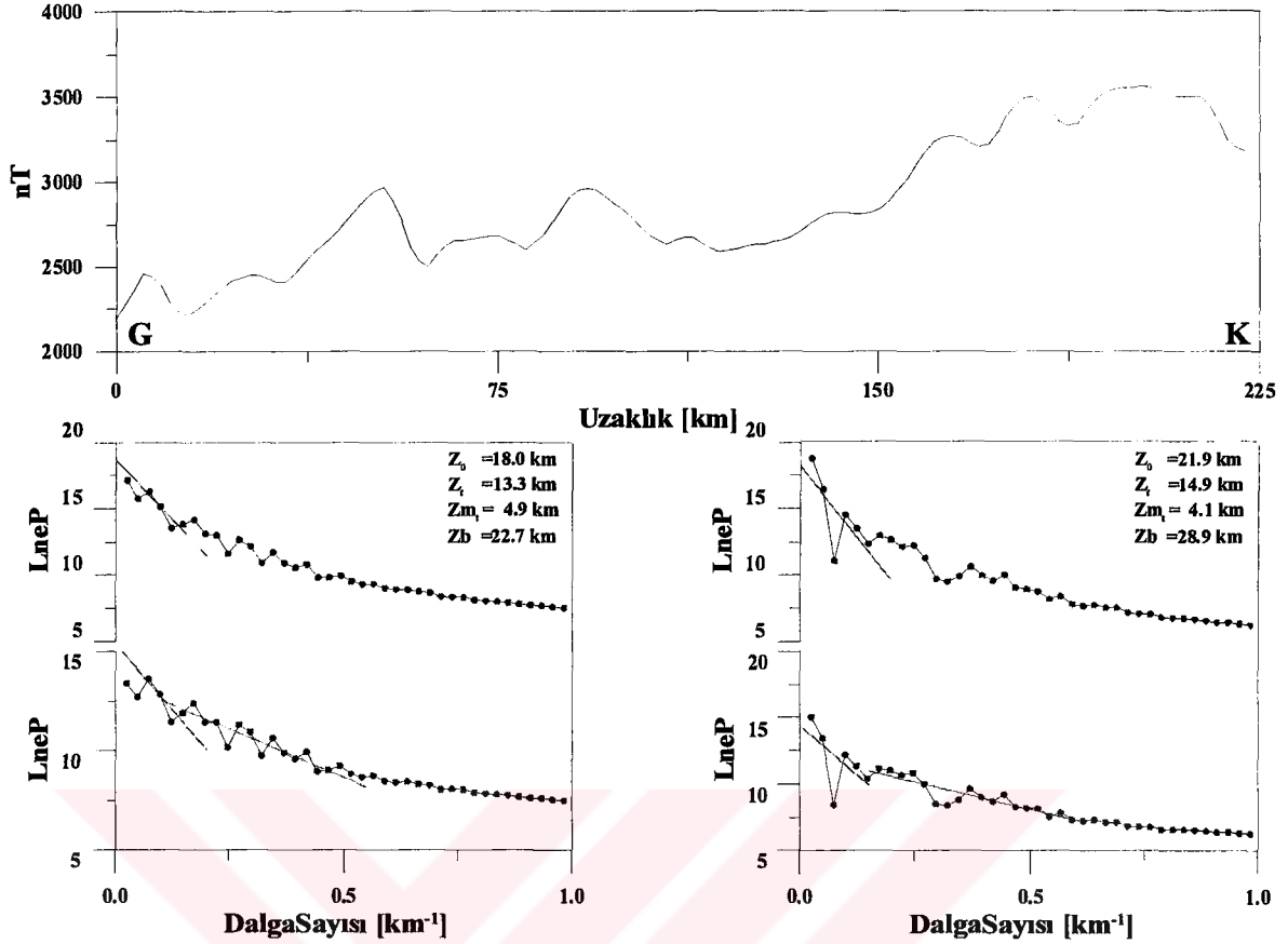
Şekil 65. Doğu Pontidlerin kutba indirgenmiş manyetik anomali haritasından 40° boylamı üzerinde alınan EE' profili (Şekil 7) ve bu profile ait güç spektrumu eğrileri. Güç spektrumu eğrilerinden belirlenen değerler, manyetik kaynağın ortalama derinliğini ( Z_0 ), üst yüzey derinliğini ( Z_1 ), manyetik tortulun temel derinliğini ( Z_m ) ve Curie noktası derinliğini ( Z_b ) göstermektedir
