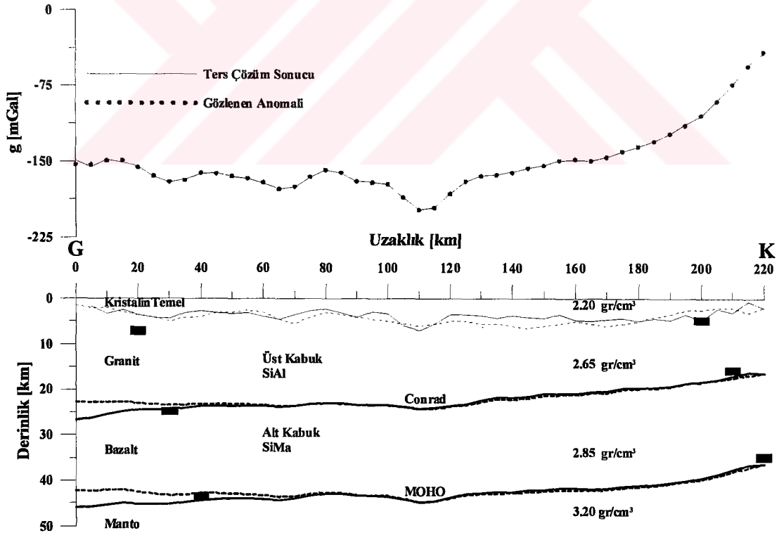
Şekil 76. Ters çözüm sonucu 41° boylamına ait FF' gravite anomali profili (Şekil 6) altındaki iki boyutlu kabuk yapısı. Kesikli çizgiler başlangıç modelini, sürekli çizgiler ters çözüm sonucu elde edilen kabuk modelini, içi dolu dikdörtgenler güç spektrumu ile hesaplanan derinlikleri göstermektedir
