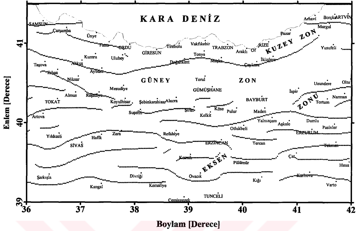
Şekil 19. Bouguer gravite verisine 80 km dalga boyu alçak geçişli süzgeç uygulanarak hesaplanan gravite verisinin tam yatay türev çizgisellik haritası
