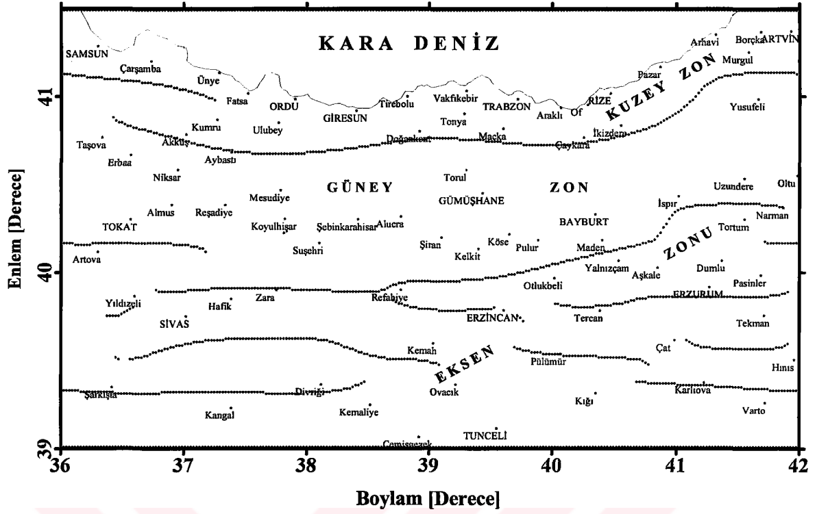
Şekil 21. Bouguer gravite anomali verisine 120 km dalga boyu alçak geçişli süzgeç uygulanarak hesaplanan gravite verilerinin tam yatay türev çizgisellik haritası
