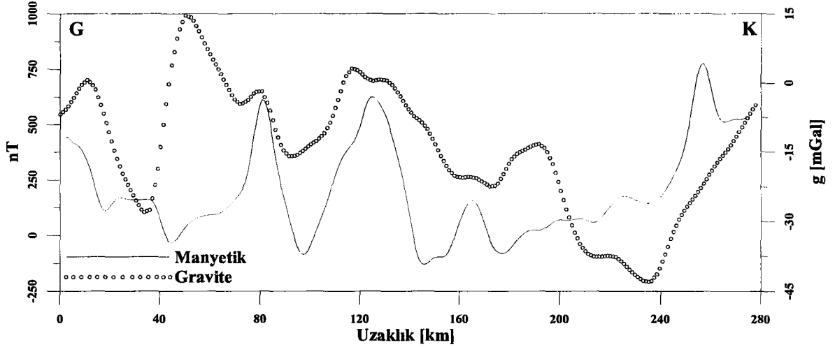
Şekil 42. Doğu Pontidlerin Bouguer gravite ve manyetik anomali haritalarından GG' kesiti (Şekil 34, 35) boyunca alınan profillere ait verilere yüksek geçişli süzgeç uygulanarak elde edilen rezidüel gravite ve manyetik anomali değerleri
