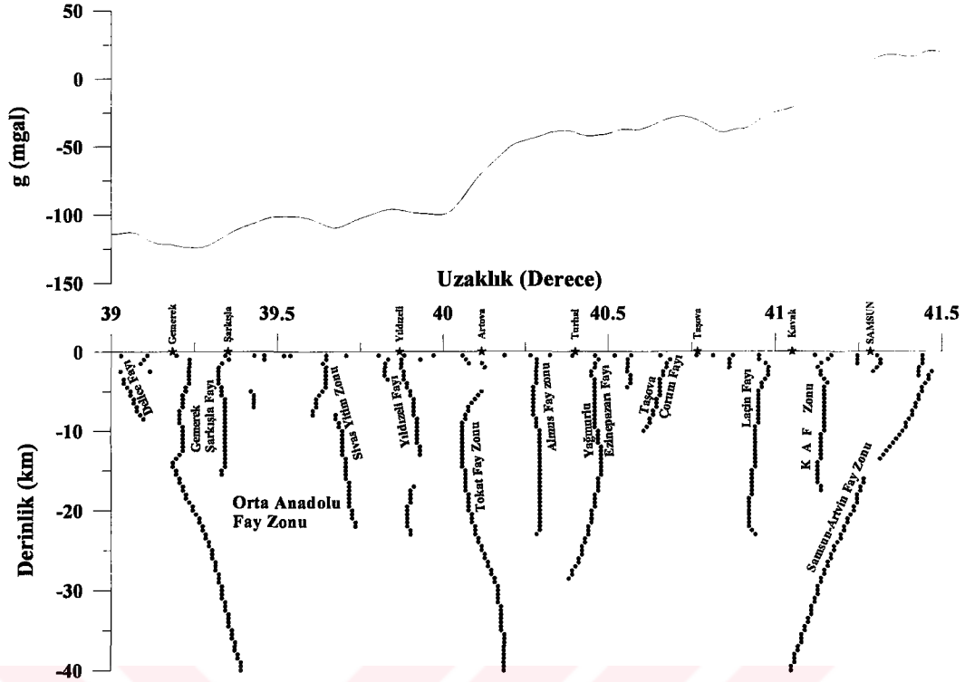
Şekil 25. 36° boylamı üzerinde alınan AA' gravite anomali profilinin (Şekil 12) alçak geçişli süzgeç anomalilerinin tam yatay türevleri alınarak oluşturulan iki boyutlu kırık yapısı
