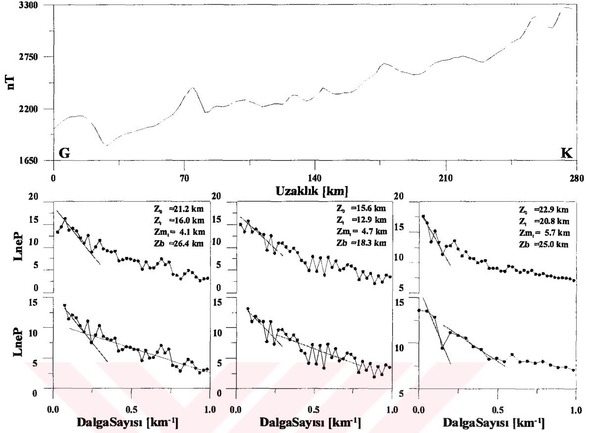
Şekil 61. Doğu Pontidlerin kutba indirgenmiş manyetik anomali haritasından 36° boyları üzerinde alınan AA' profili (Şekil 7) ve bu profile ait güç spektrumu eğrileri. Güç spektrumu eğrilerinden belirlenen değerler, manyetik kaynağın ortalama derinliğini ( Z_0 ), üst yüzey derinliğini ( Z_t ), manyetik tortulun temel derinliğini ( Z_{mt} ) ve Curie noktası derinliğini ( Z_b ) göstermektedir
