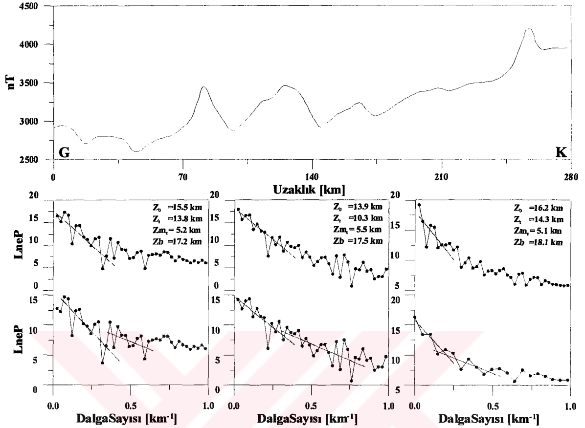
Şekil 67. Doğu Pontidlerin kutba indirgenmiş manyetik anomali haritasından 42^\circ boyları üzerinde alınan GG' profili (Şekil 7) ve bu profile ait güç spektrumu eğrileri. Güç spektrumu eğrilerinden belirlenen değerler, manyetik kaynağın ortalama derinliğini ( Z_0 ), üst yüzey derinliğini ( Z_t ), manyetik tortulun temel derinliğini ( Z_{mt} ) ve Curie noktası derinliğini ( Z_b ) göstermektedir
