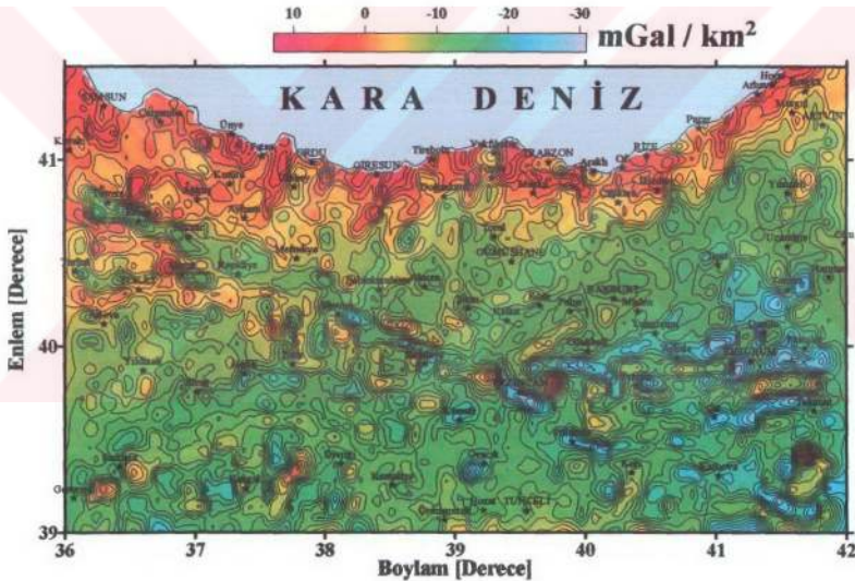
Şekil 32. Doğu Pomidlerin Bouguer gravite verilerinin Elkins (1951) bağıntısıyla hesaplanmış düşey ikinci türev anomali haritası. Kontur aralığı 2 mGal/km 2 'dir
