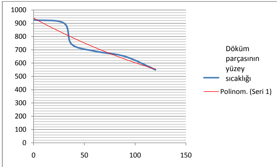
řekil.12 Dokm parasının yzey sıcaklıęı ve ona en yakın ikinci dereceden polinom eęrisini birlikte gsteren grafik
