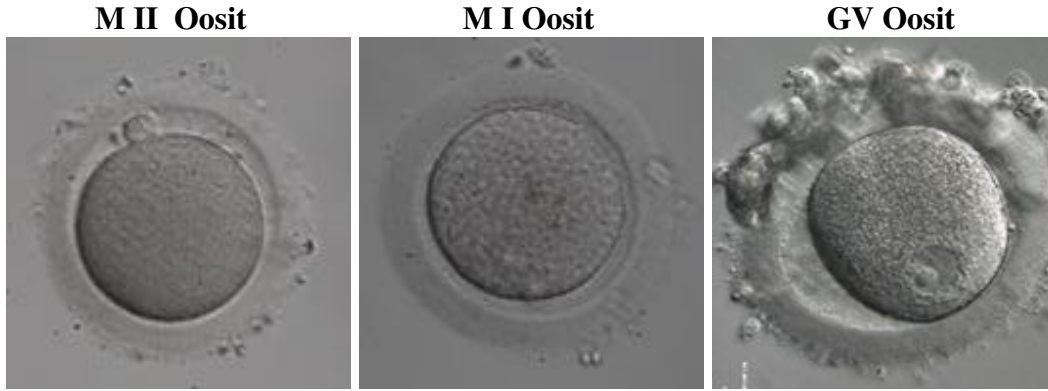
Şekil 6. Oosit matürasyonu
