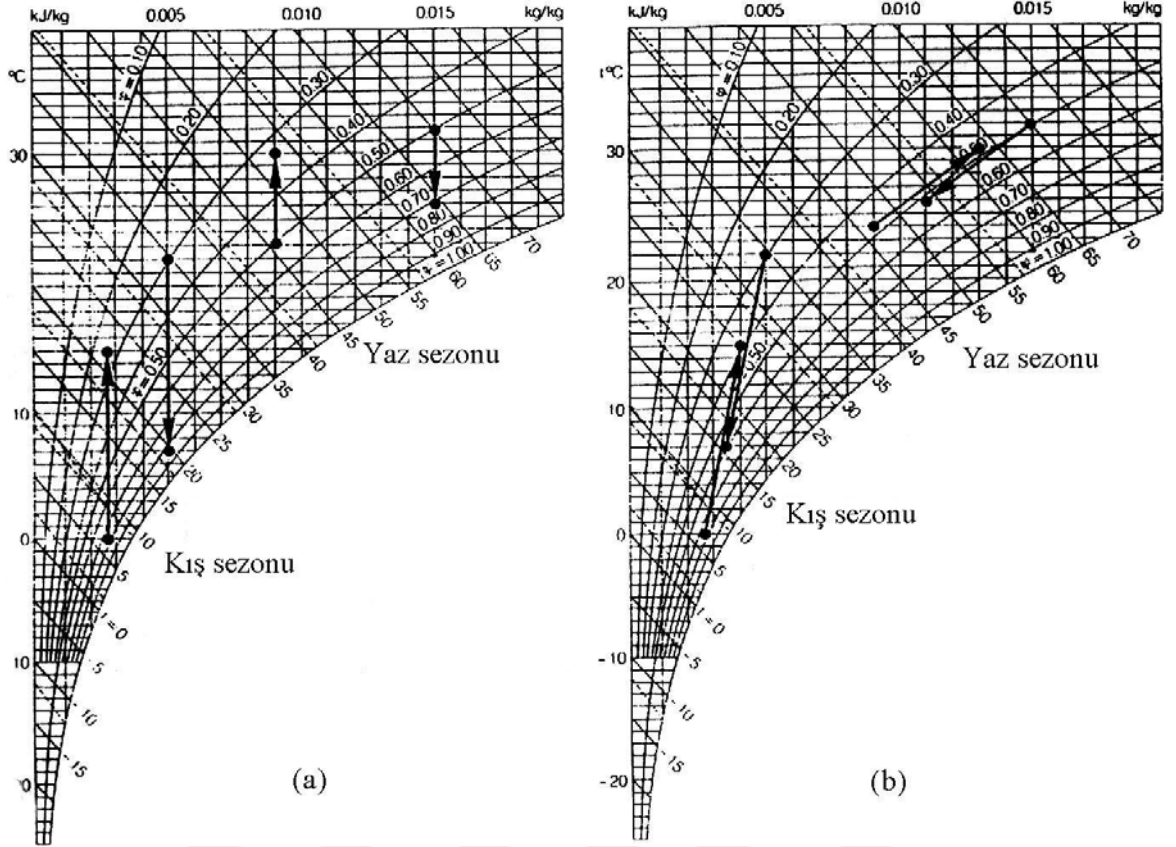
Şekil 5.1. Higroskopik olan ve olmayan döner tip ısı değiştiricilerde hal değişimi
