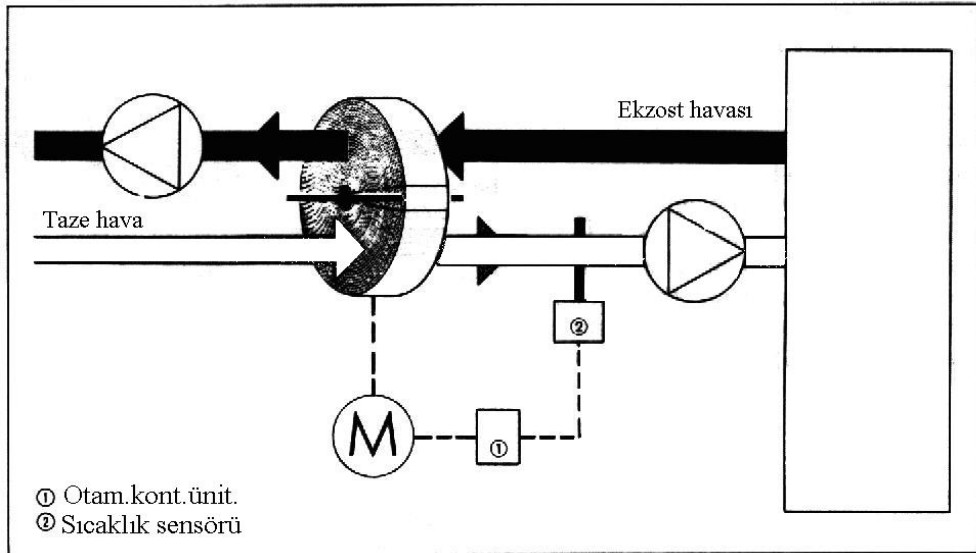
Şekil 5.11. Döner tip ısı değiştiricilerde rotor hız kontrol devresi.
