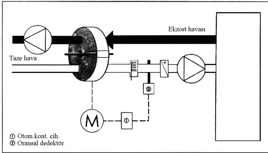
Şekil 5.10. Döner tip ısı değiştirgeçlerinde don kontrol devresi.
