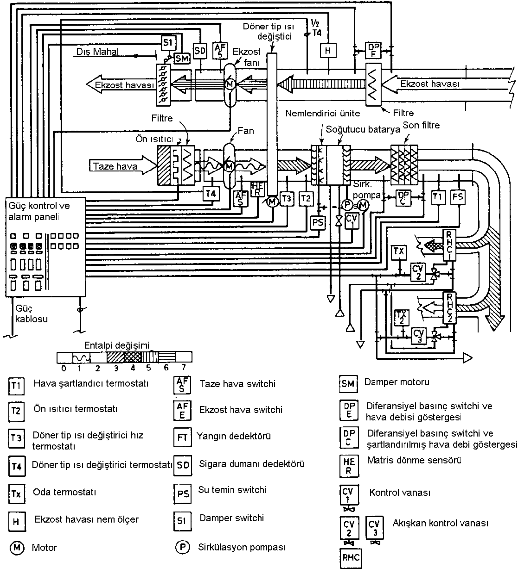
Şekil 5.12. Döner tip ısı değiştirici kullanılan klima santralinde otomatik kontrol sistemi
