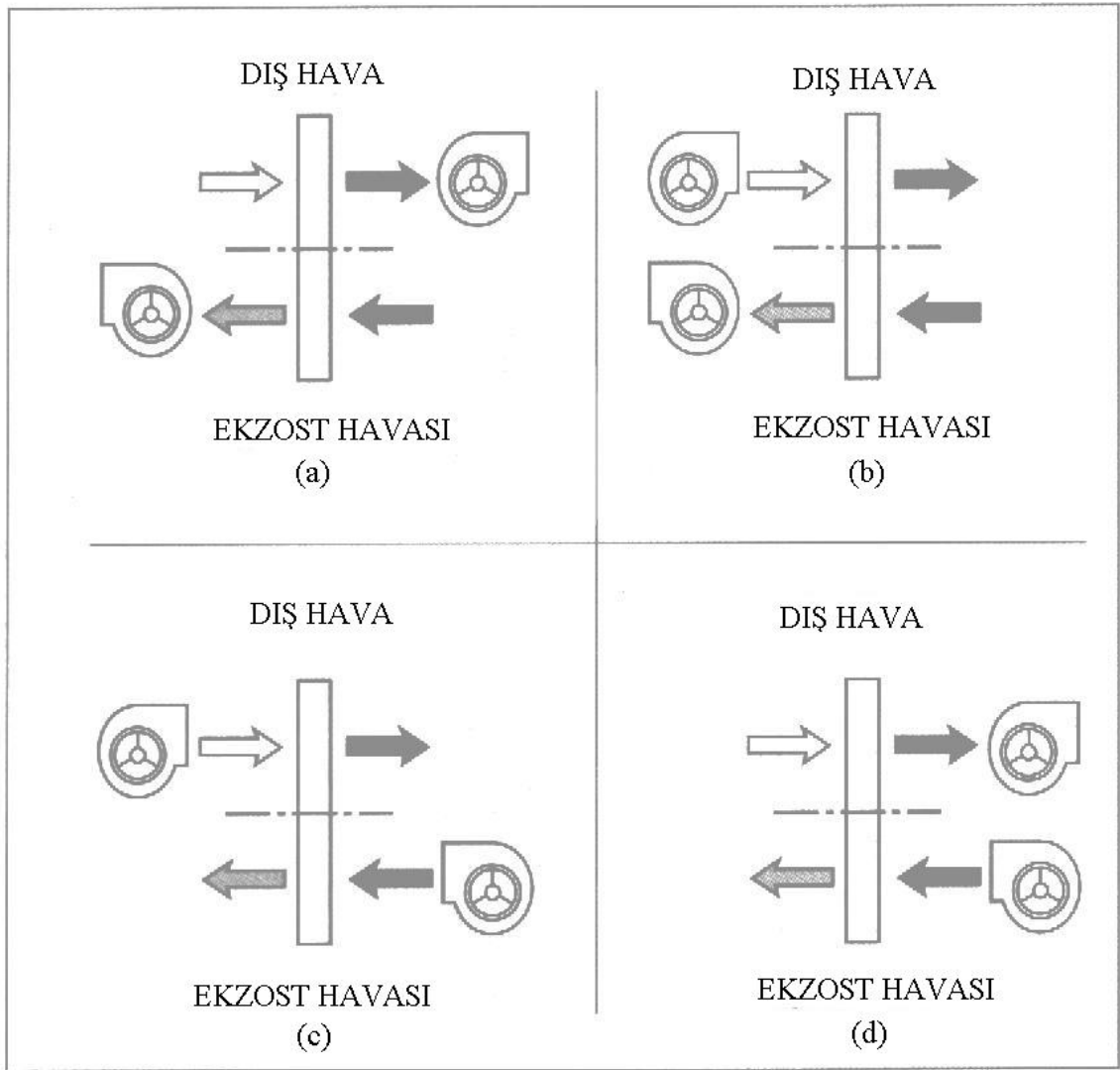
Şekil 5.7. Fanların yerleştirilme şekilleri.
