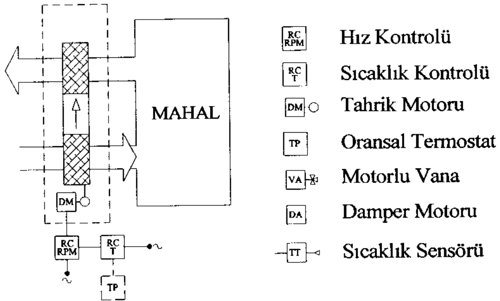
Şekil 5.8.Döner tip ısı değiştirgecinin hız kontrolü
