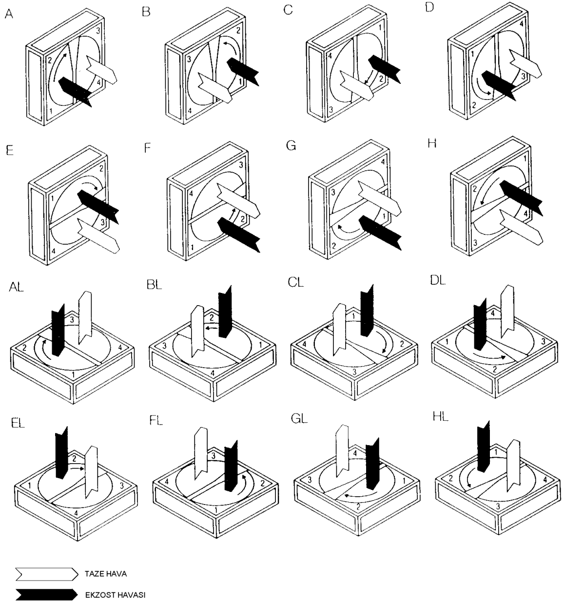
Şekil 5.13. Rotor pozisyonları
