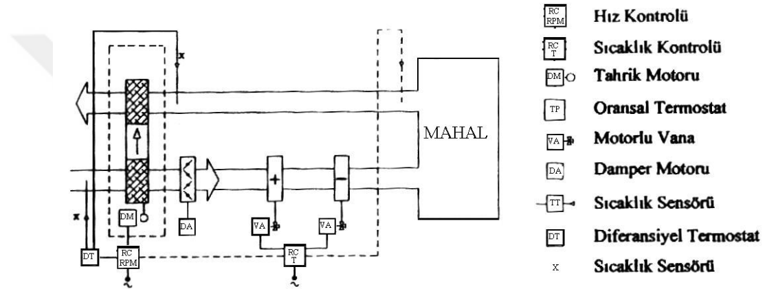
Şekil 5.9. Döner tip ısı değiştirgeçlerde ısı ve soğu geri kazanımı
