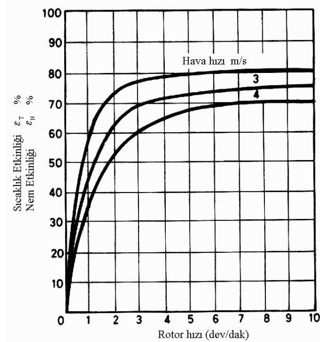
Şekil 5.4 Matrisin devir sayısına göre değişik hava hızlarında etkinlik değeri
