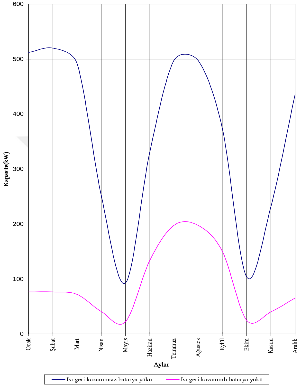
Şekil8.3.Isıtma ve soğutma sezonlarında, döner tip ısı değıştirici kullanılması ve kullanılmaması halindeki batarya yükleri
