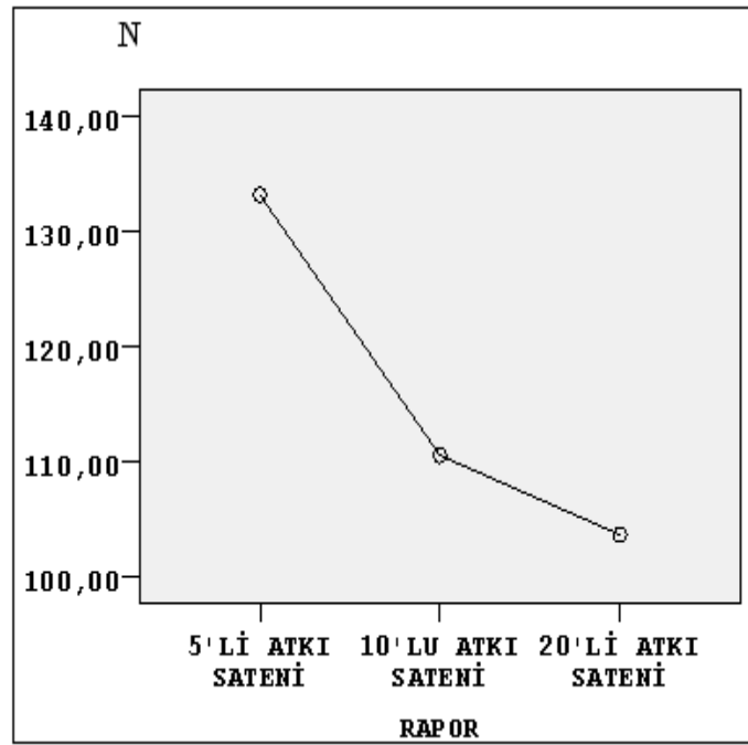
Şekil 4.24 Poliester çözgülü kumaşların rapor-çözgü doğrultusunda ipliklerin dikiş kaymasına karşı mukavemeti grafiği
