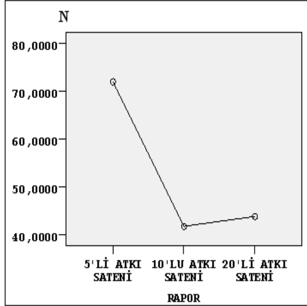
Şekil 4.39 Rayon çözgülü kumaşların rapor-atkı doğrultusunda yırtılma mukavemeti grafiği
