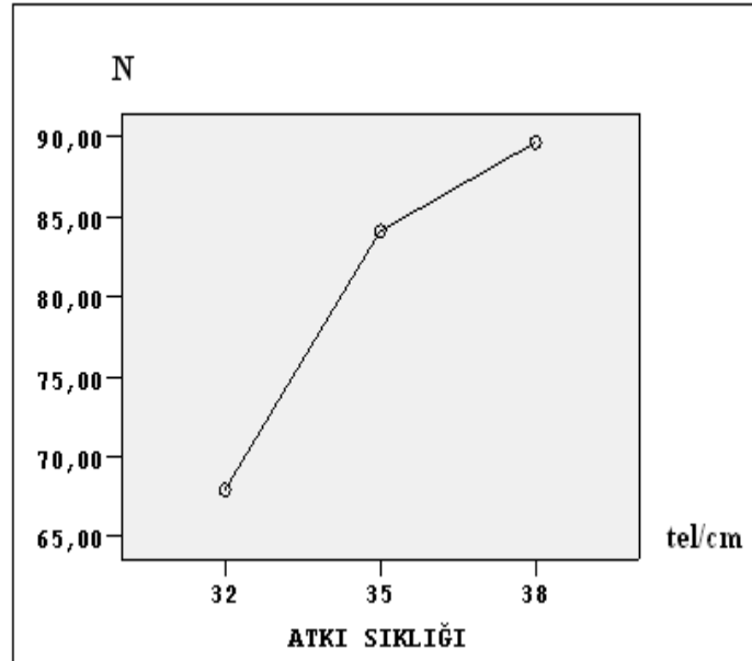
Şekil 4.42 Rayon çözgülü kumaşların atkı sıklığı-atkı doğrultusunda ipliklerin dikiş kaymasına karşı mukavemeti grafiği
