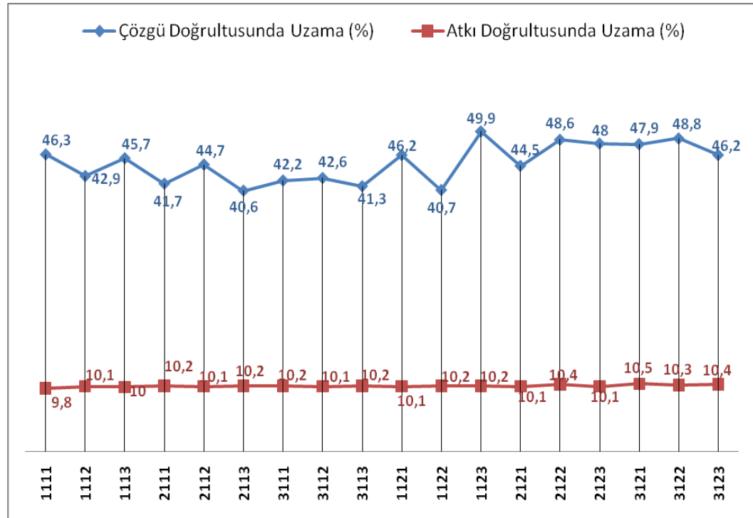
Şekil 4.2 1111- 3123 arası Poliester çözgülü döşemelik kumaşların kopma uzaması
