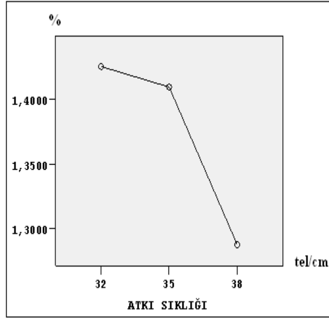
Şekil 4.44 Rayon çözgülü kumaşların atkı sıklığı-ağırlık kaybı grafiği
