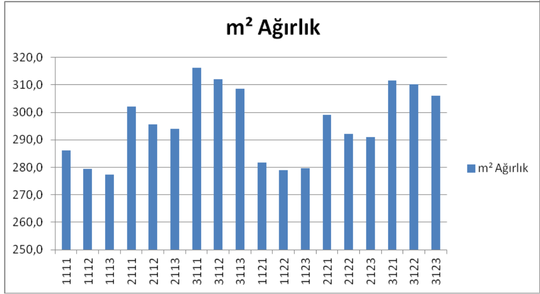
Şekil 3.1 1111-3123 arası (Poliester çözgülü) döşemelik kumaşların metrekare ağırlıkları
