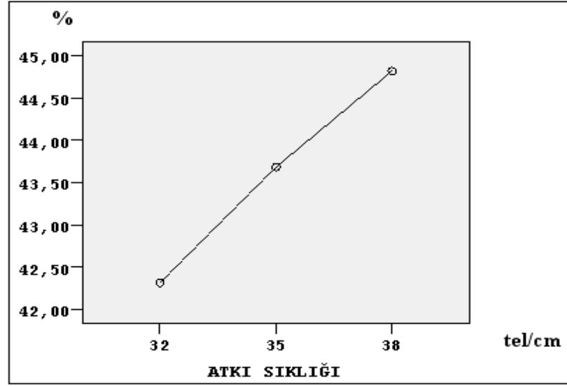
Şekil 4.15 Poliester çözgülü kumaşların atkı sıklığı-çözü doğruğultusunda kopma uzama grafiğı
