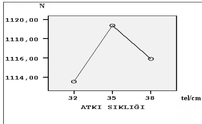
Şekil 4.29 Rayon çözgülü kumaşların atkı sıklığı-çözgü doğrultusunda kopma mukavemeti grafiği
