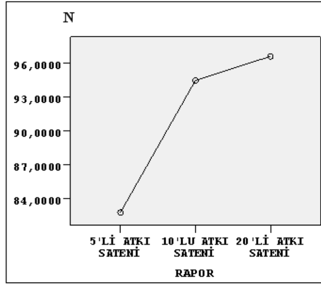
Şekil 4.22 Poliester çözgülü kumaşların rapor-atkı doğrultusunda yırtılma mukavemeti grafiği
