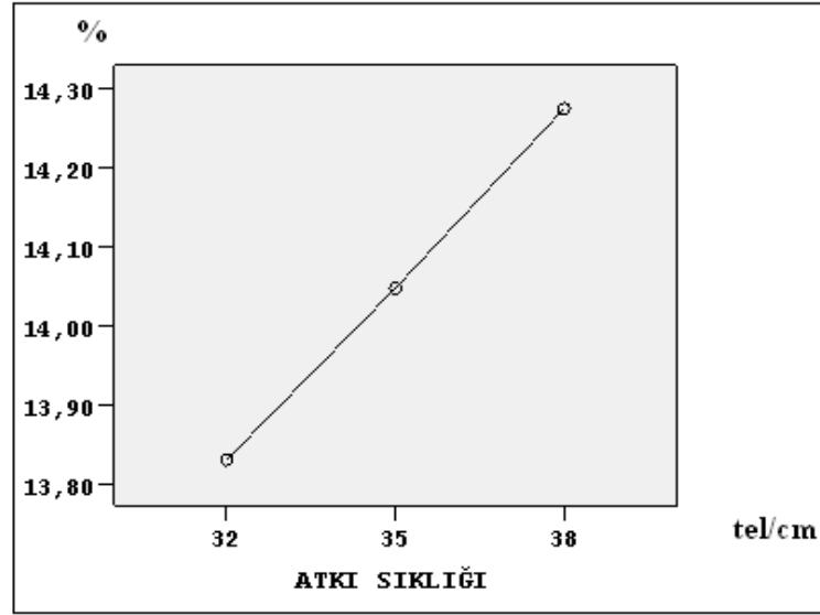
Şekil 4.17 Poliester çözgülü kumaşların atkı sıklığı-atkı doğrultusunda kopma uzama grafiği
