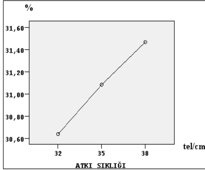
Şekil 4.33 Rayon çözgülü kumaşların atkı sıklığı-çözgü doğrultusunda uzama grafiği
