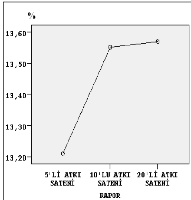
Şekil 4.35 Rayon çözgülü kumaşların rapor-atkı doğrultusunda uzama grafiği
