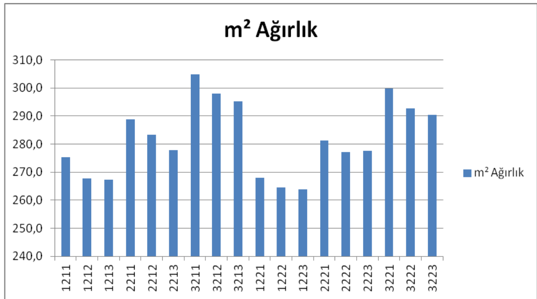
Şekil 3.2 1211-3223 arası (Rayon çözgülü) döşemelik kumaşların metrekare ağırlıkları
