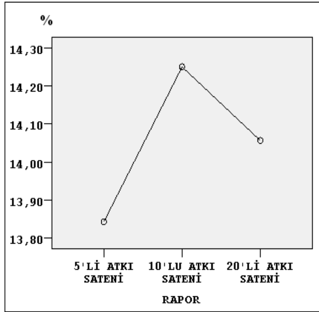
Şekil 4.18 Poliester çözgülü kumaşların rapor-atkı doğrultusunda kopma uzama grafiği
