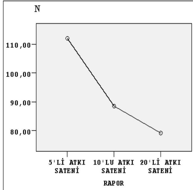
Şekil 4.26 Poliester çözgülü kumaşların rapor-atkı doğrultusunda ipliklerin dikiş kaymasına karşı mukavemeti grafiği
