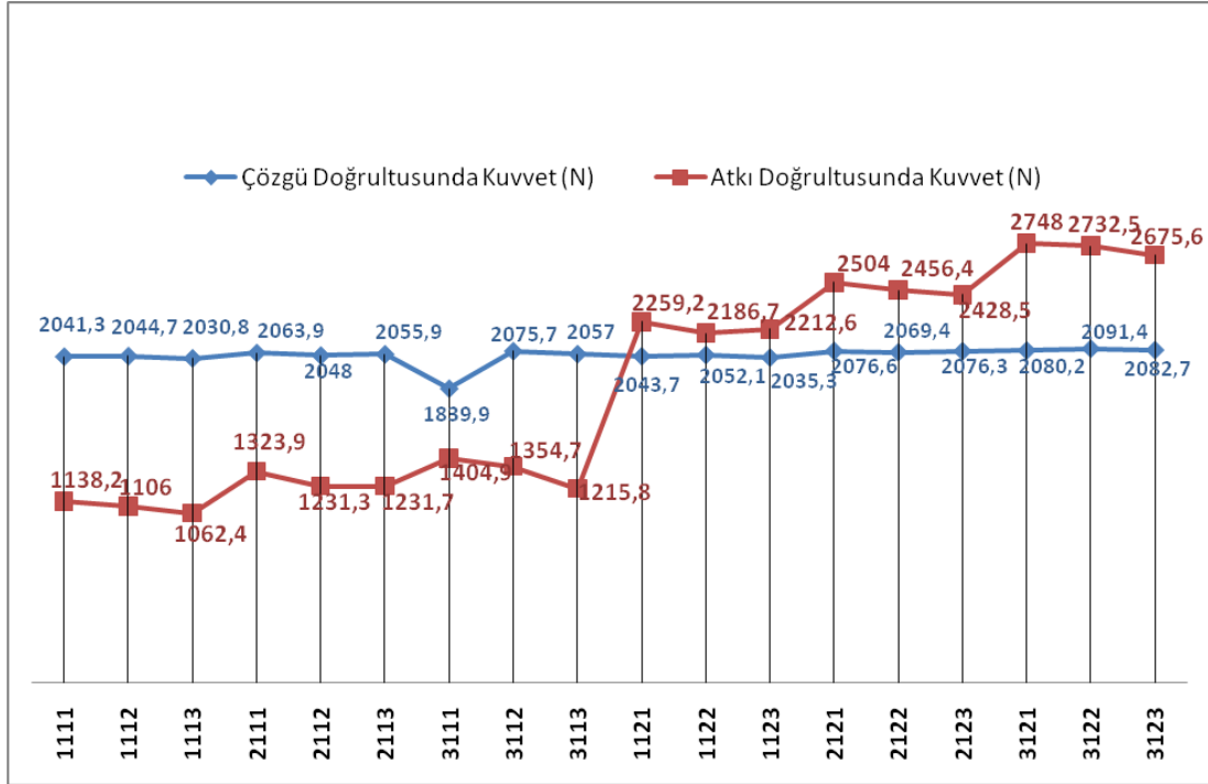
Şekil 4.1 1111- 3123 arası Poliester çözgümlü dşşemelik kumaşların kopma mukavemeti
