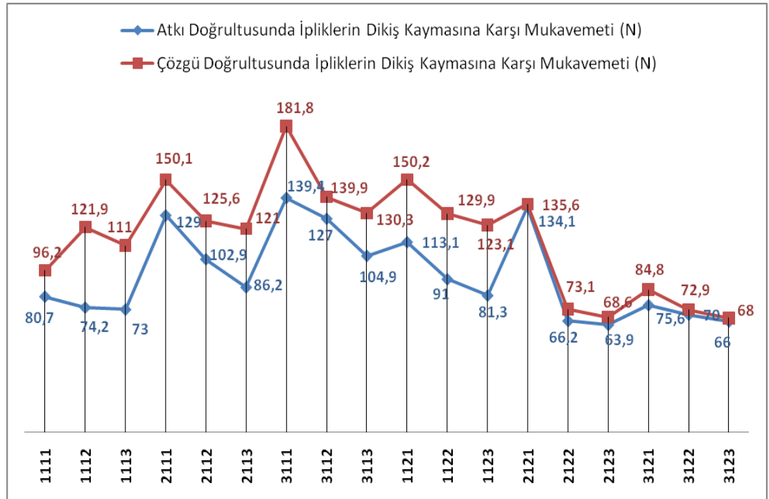
Şekil 4.4 1111- 3123 arası Poliester çözgülü döşemelik kumaşlardaki ipliklerinin dikiş kaymasına karşı mukavemeti
