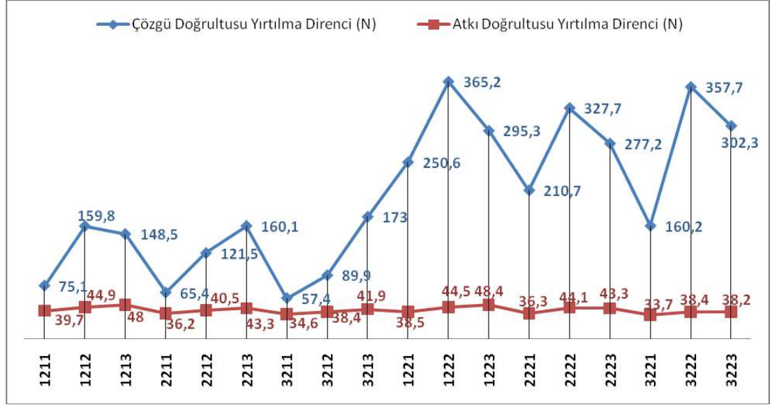
Şekil 4.8 1211- 3223 arası Rayon çözgü dōşemelik kumaşların yırtılma mukavemeti
