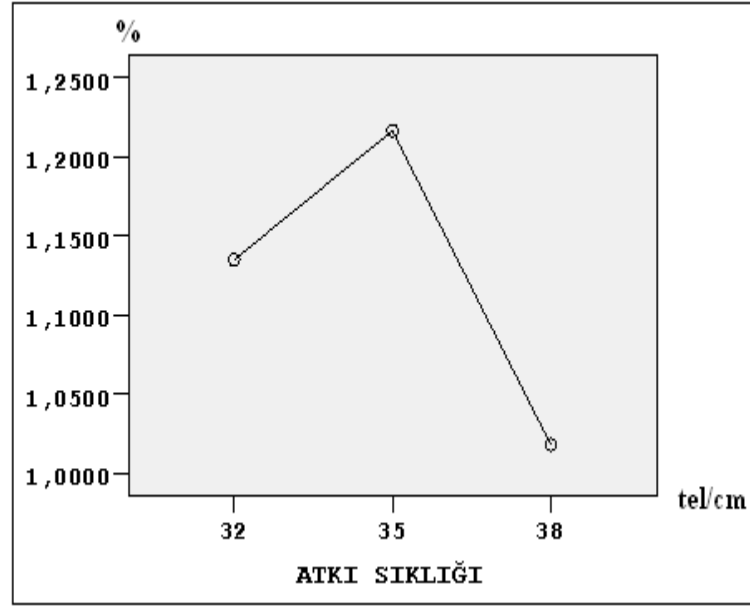
Şekil 4.27 Poliester çözgülü kumaşların atkı sıklığı-ağırlık kaybı grafiği
