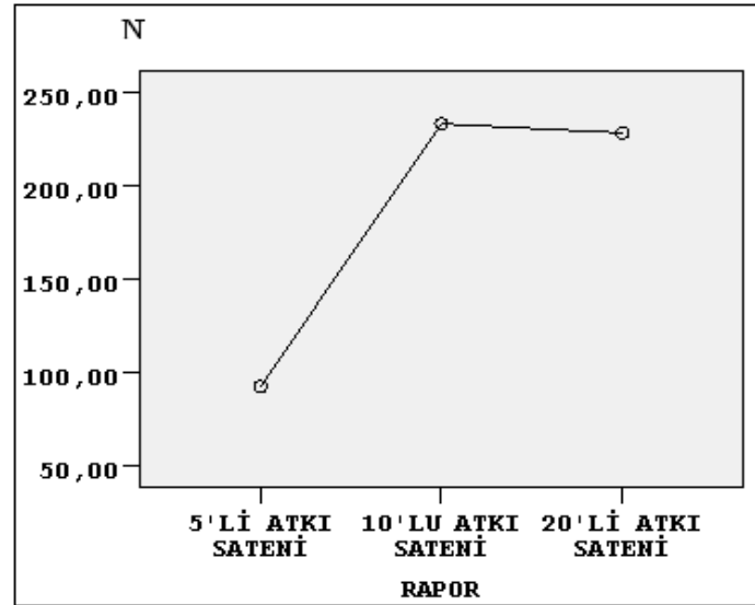
Şekil 4.20 Poliester çözgülü kumaşların rapor-çözgü doğrultusunda yırtılma mukavemeti grafiği
