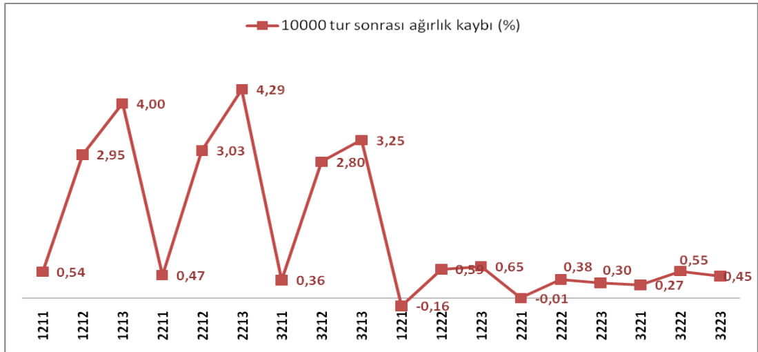
Şekil 4.10 1211- 3223 arası Rayon çözgümlü döşemelik kumaşların ağırlık kaybı
