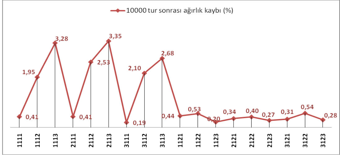
Şekil 4.5 1111- 3123 arası Poliester çözgülü döşemelik kumaşların ağırlık kaybı
