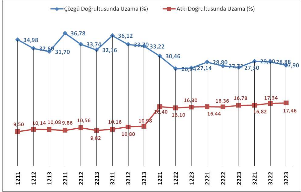
Şekil 4.7 1211- 3223 arası Rayon çözgü dökemelik kumaşların kopma uzama
