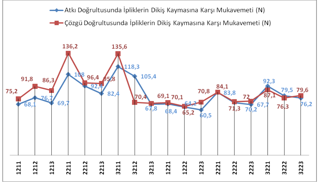
Şekil 4.9 1211-3223 arası Rayon çözgü dökşemelik kumaşlardaki ipliklerinin dikiş kaymasına karşı mukavemeti
