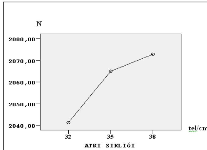
Şekil 4.11 Poliester çözgülü kumaşların atkı sıklığı-çözgü doğrultusunda kopma mukavemeti grafiği
