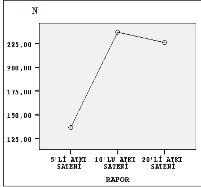
Şekil 4.37 Rayon çözümlü kumaşların rapor-çözgü doğrultusunda yırtılma mukavemeti grafiği
