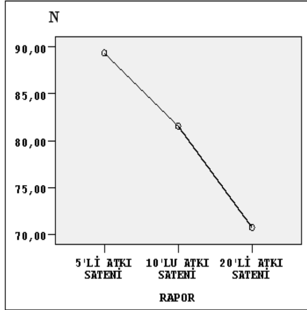
Şekil 4.43 Rayon çözgülü kumaşların rapor-atkı doğrultusunda ipliklerin dikiş kaymasına karşı mukavemeti grafiği
