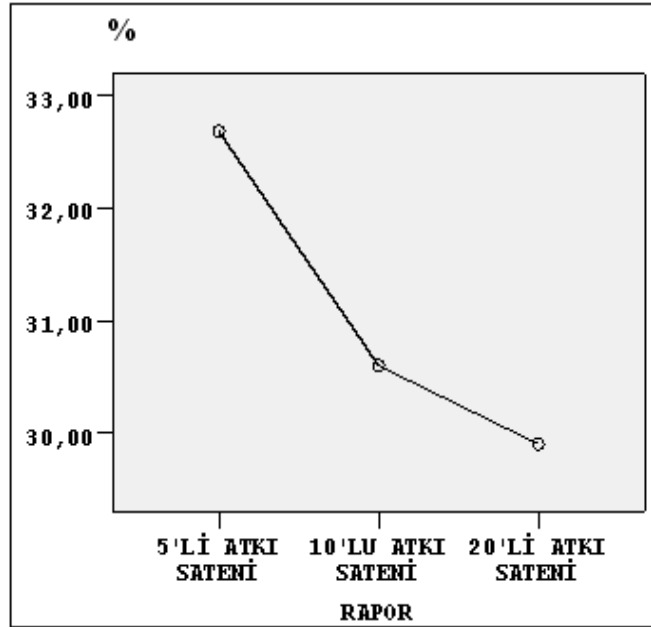
Şekil 4.34 Rayon çözgülü kumaşların rapor-çözgü doğrultusunda uzama grafiği
