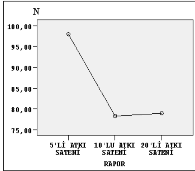
Şekil 4.41 Rayon çözgülü kumaşların rapor-çözgü doğrultusunda ipliklerin dikiş kaymasına karşı mukavemeti grafiği
