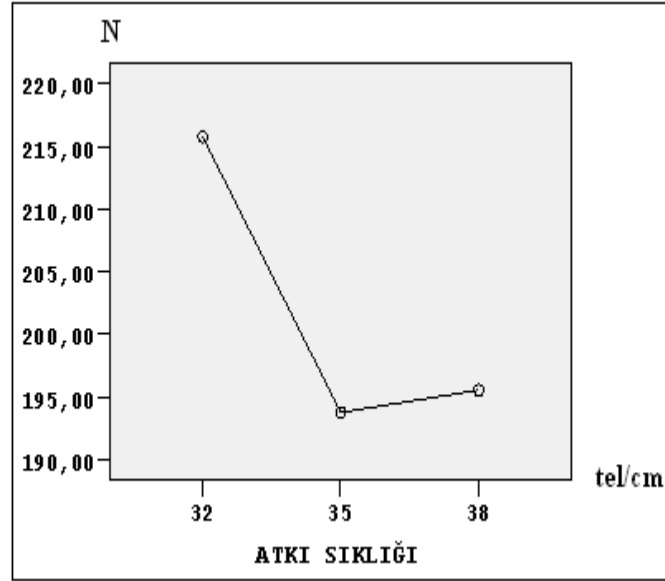
Şekil 4.36 Rayon çözgülü kumaşların atkı sıklığı-çözgü doğrultusunda yırtılma mukavemeti grafiği
