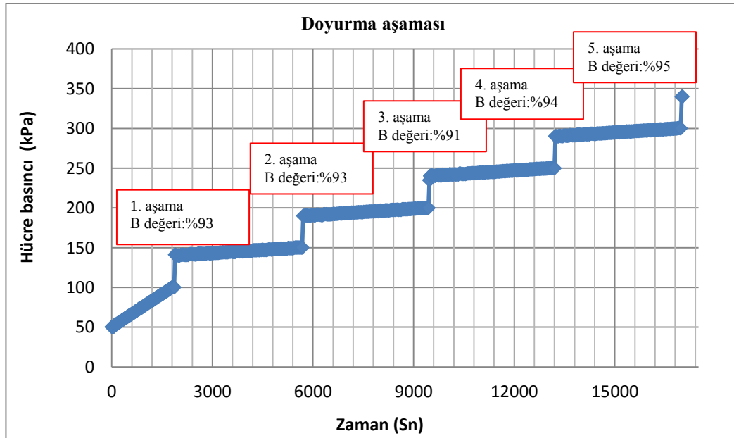
Şekil 5.4. Doyurma aşamasında hücre basıncı değerine karşılık numunenin doyma yüzdesi ilişkisi.
