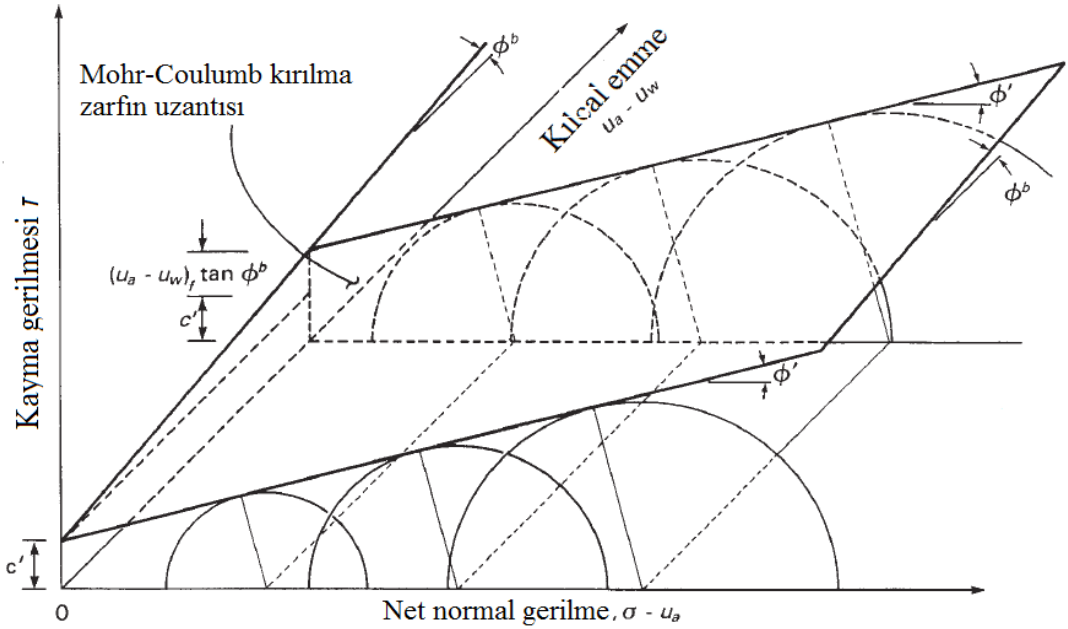
Şekil 3.3. Doymun olmayan zeminlerin Mohr-Dairenin kırılma zarfı [8]
