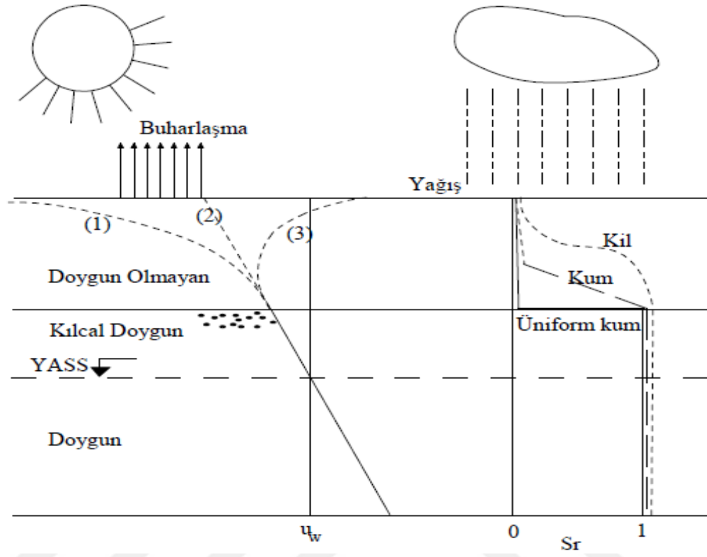
Şekil 1.5. Yer yüzeyin akıntı durumu gösteren zemin mekaniğin görselleştirmesi [5]
