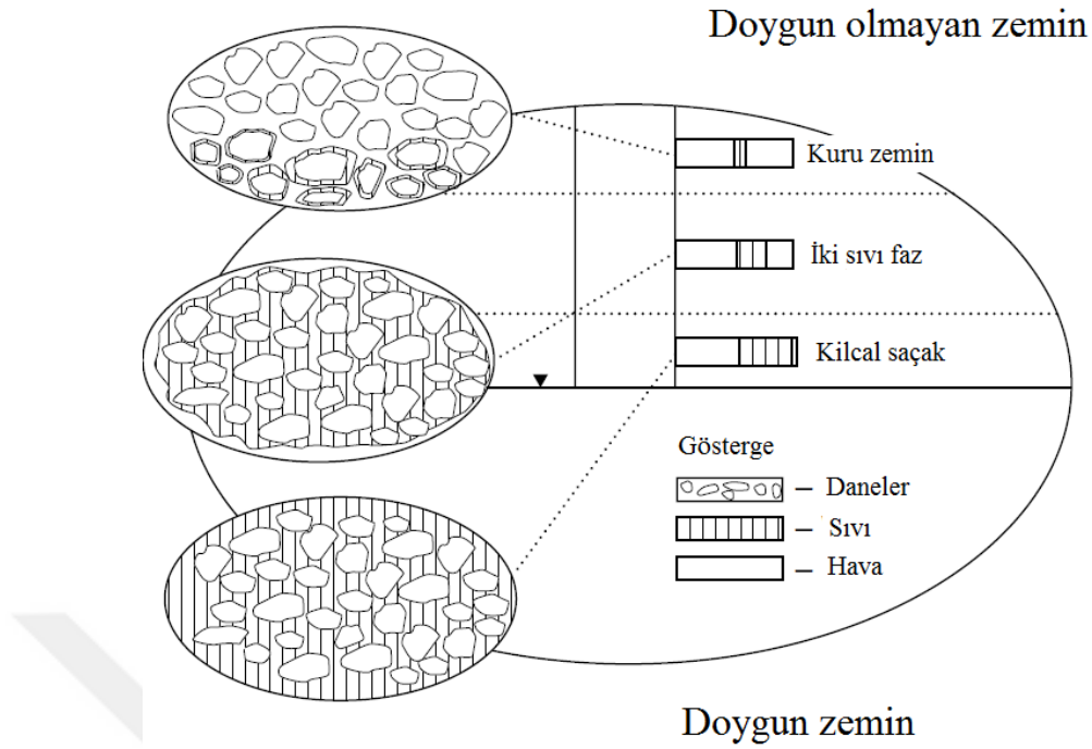
Şekil 1.2. Yeraltı su tabakasının üstündeki zeminin doygunluk derece değişimine göre kategorizasyonu [4]
