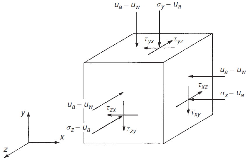
Şekil 3.1. Doygun olmayan zeminde gerilme durum değişkenleri [8]
