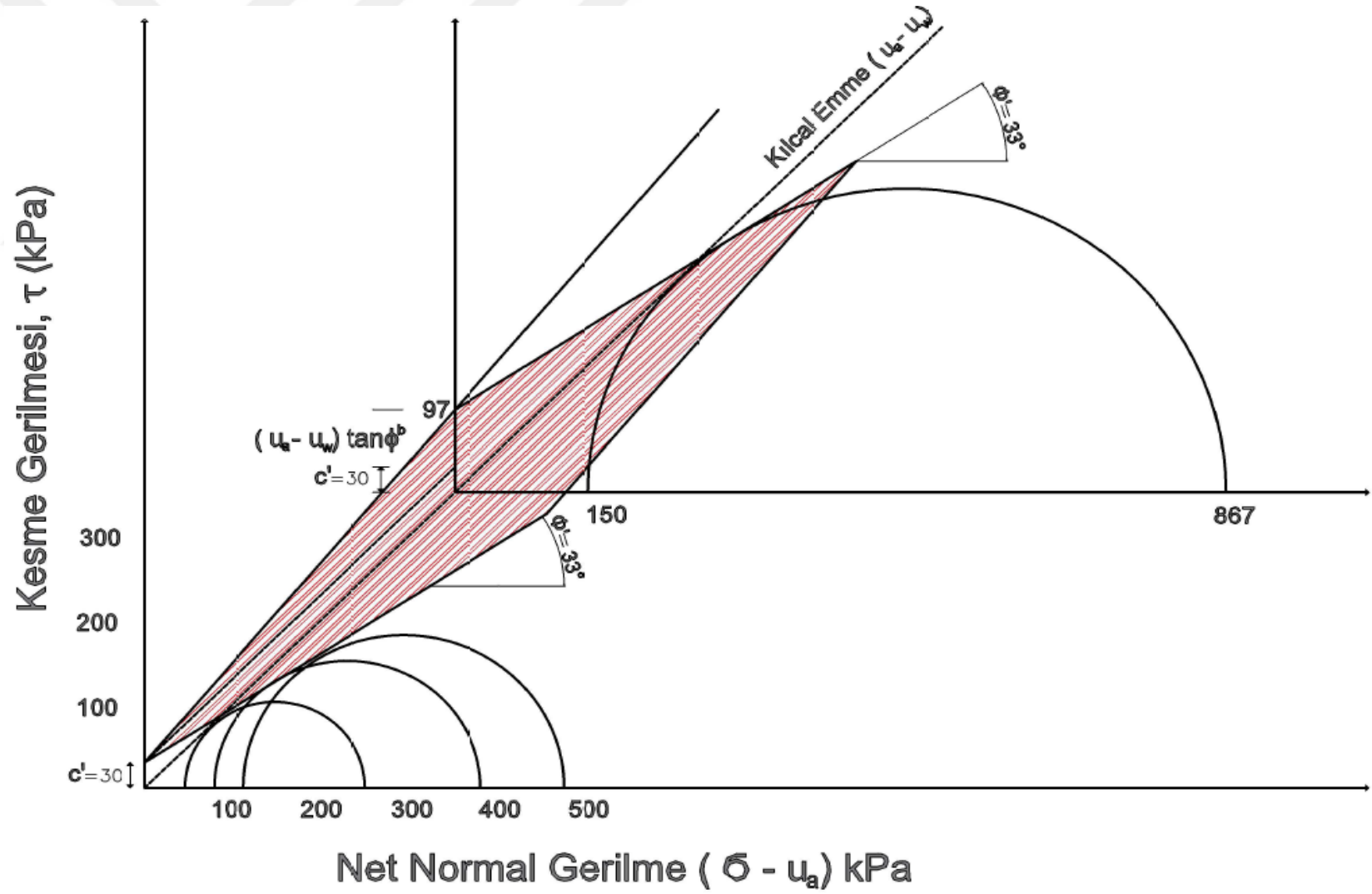
Şekil 6.1. Doymun olmayan zemin deneylerin mohr daire uzantısı
