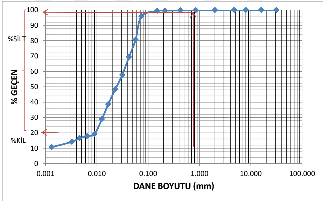
Şekil 4.1. Çalışmada kullanılan numunenin hidrometre deneyi sonucu
