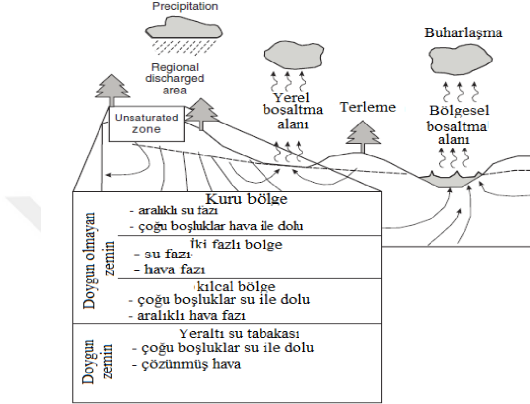
Şekil 1.3. Doygun olmayan bölgenin (Vadoz bölgesi) yerel ve ya bölgesel olarak bölünmesi [3]
