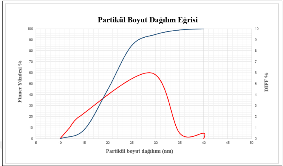
Şekil 4.2. \text{Fe}_3\text{O}_4 NP (14-29 nm) PSD analiz sonuç grafiği
