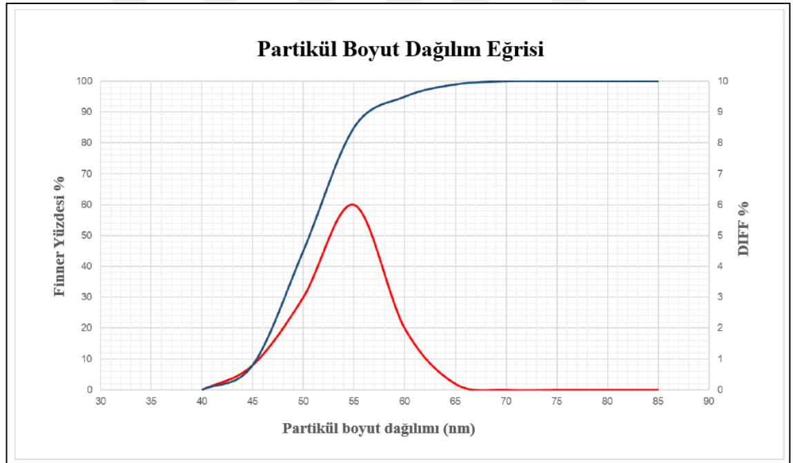
Şekil 4.3. \text{MnFe}_2\text{O}_4 (55 nm) PSD analiz sonuç grafiği
