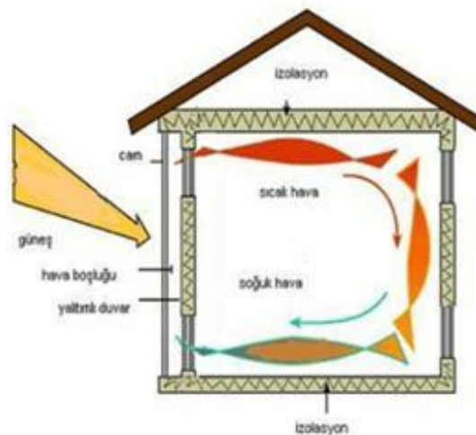
Şekil 2.2 : Dolaylı kazanım sistemlerinden biri olan Güneş duvarının prensip şeması [13].
