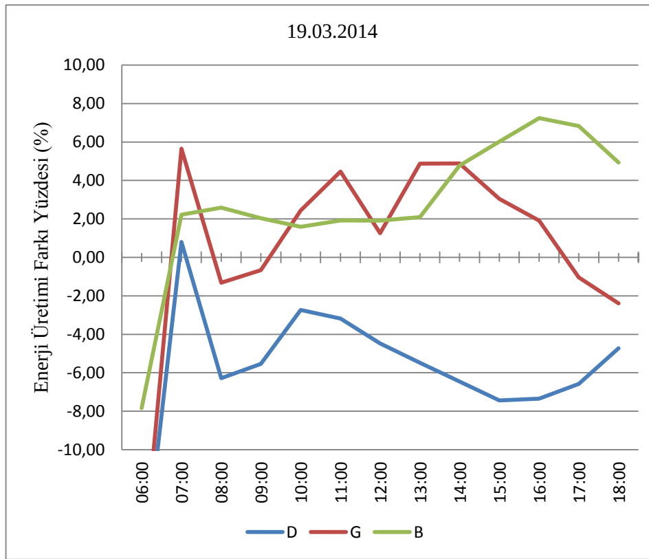
Şekil 5.17 : Mart ayının en soğuk (a) ve en sıcak (b) günlerinde, farklı yönlerde gerçekleşen enerji üretimi farklılıkları.
