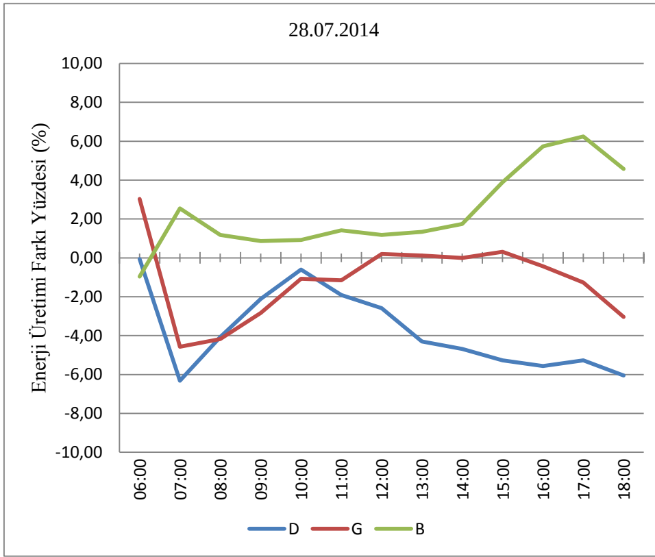
Şekil 5.19 : Temmuz ayının en soğuk (a) ve en sıcak (b) günlerinde, farklı yönlerde gerçekleşen enerji üretimi farklılıkları.
