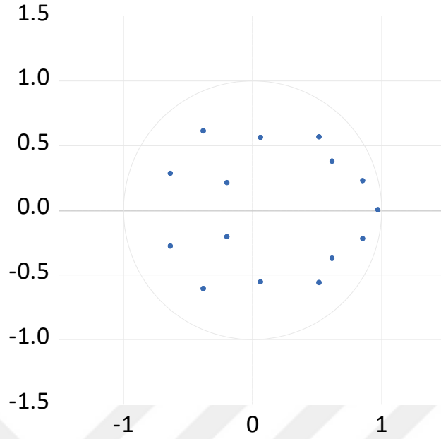
Şekil 10. VAR Modelinin Karakteristik Ters Kökleri
