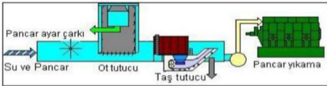
Şekil 2: Pancar Ayrıştırma İşlemi
