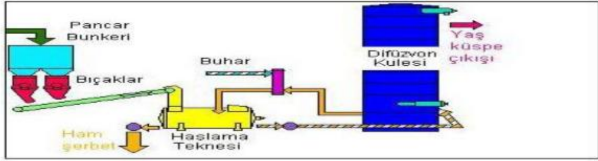
Şekil 3: Pancar Kıyım ve Haşlama İşlemi
