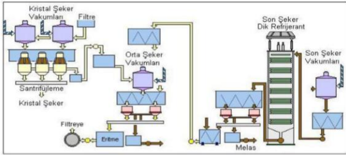
Şekil 7: Kristal Lapa Pişirim İşlemi
