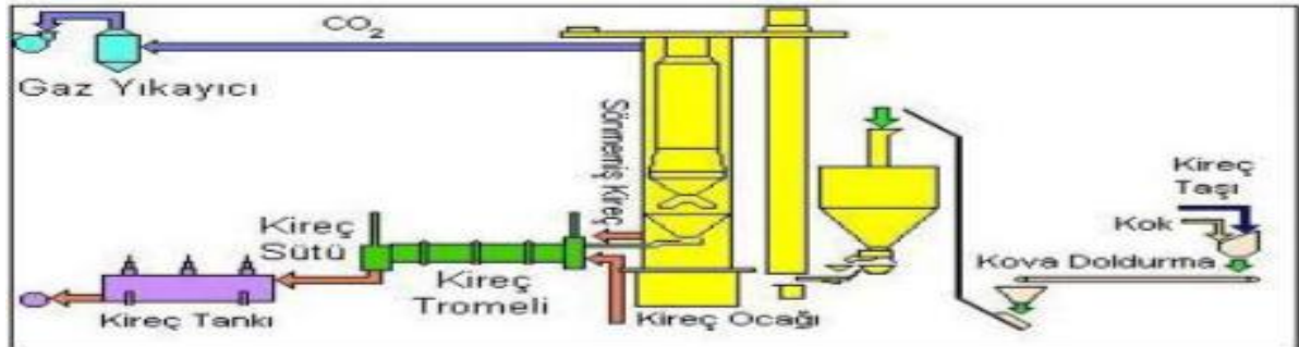
Şekil 4: Birinci Kireçleme İşlem
