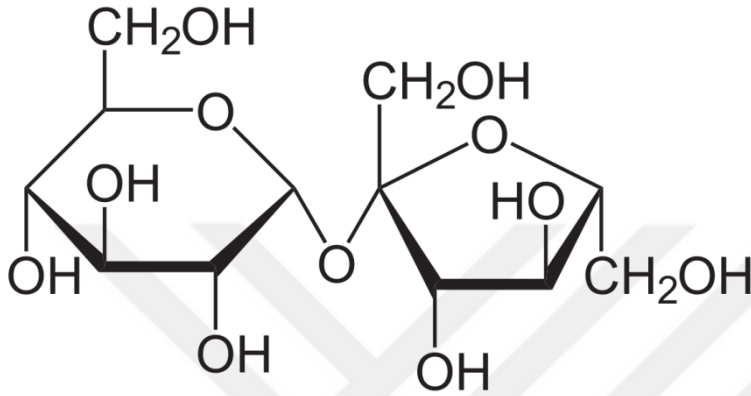
Şekil 1: Şekerin Kimyasal formülü
