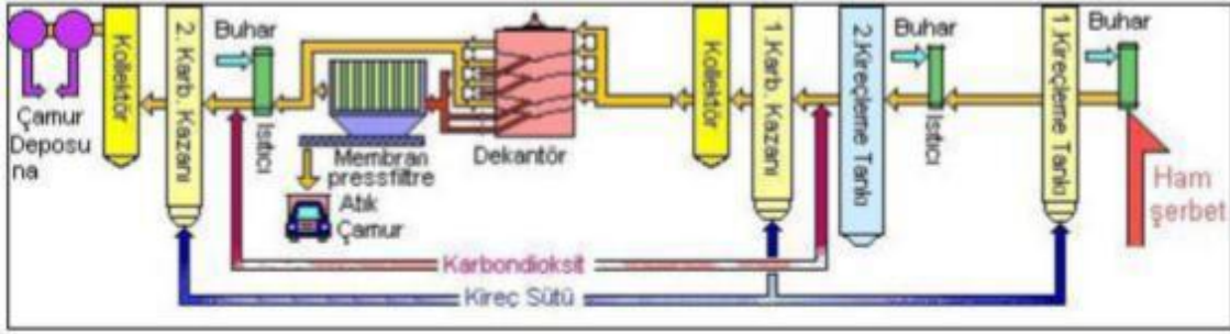
Şekil 5: İkinci Kireçleme İşlemi
