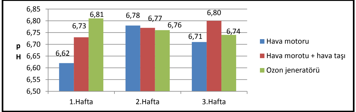
Çizelge 4.29. Farklı oksijen uygulamalarına ait haftalara göre pH değişimleri
