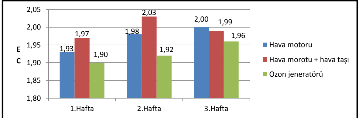
Çizelge 4.30. Farklı oksijen uygulamalarına ait haftalara göre EC değişimi
