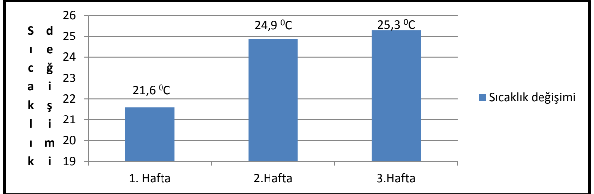
Çizelge 4.33. Haftalara göre sera içi sıcaklık değişimi
