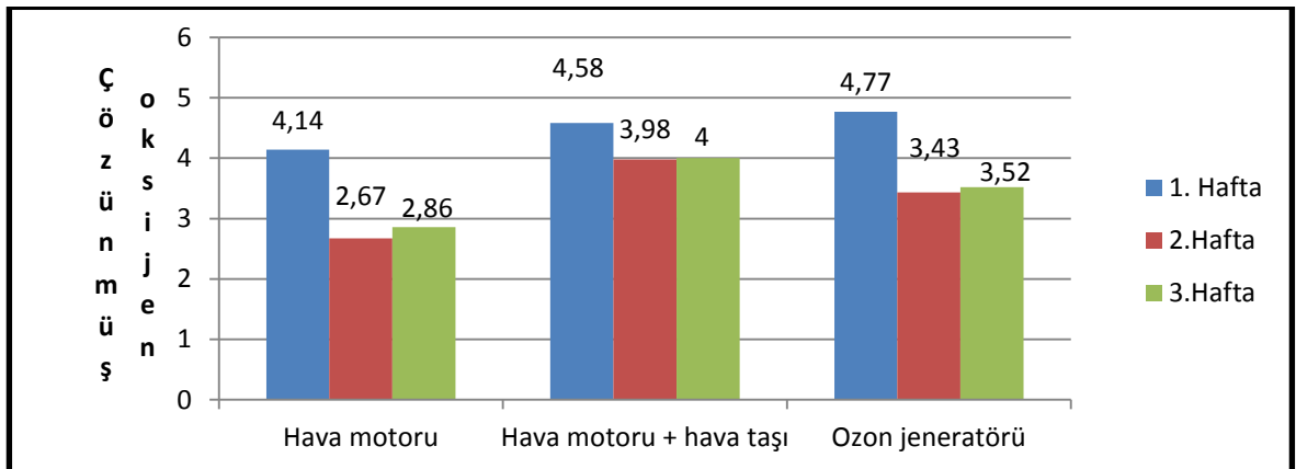
Çizelge 4.32. Farklı oksijen uygulamalarına ait haftalara göre besin solüsyonundaki çözünmüş oksijen değişimi
