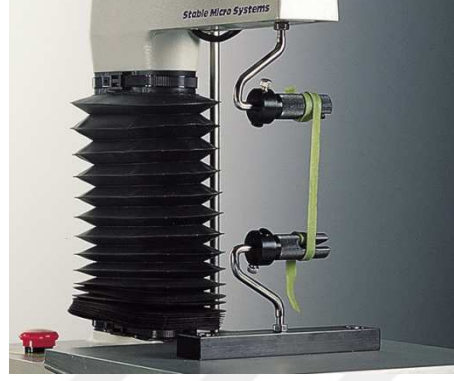
Şekil 3.6: Elastikiyet Testi Donanımı
