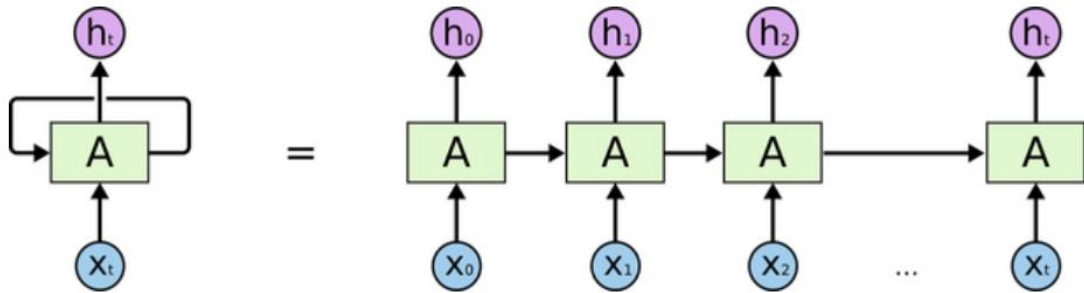
Şekil 3. 1. Döngü ile Temel RNN'lerin Yapısı
