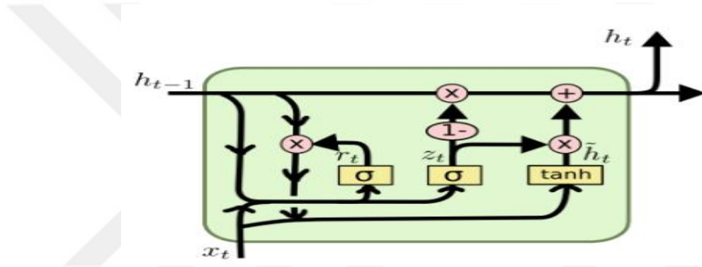
Şekil 3. 5. GRU Yapısı
