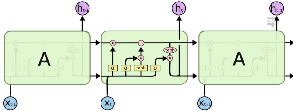
Şekil 3. 3. LSTM Yapısı
