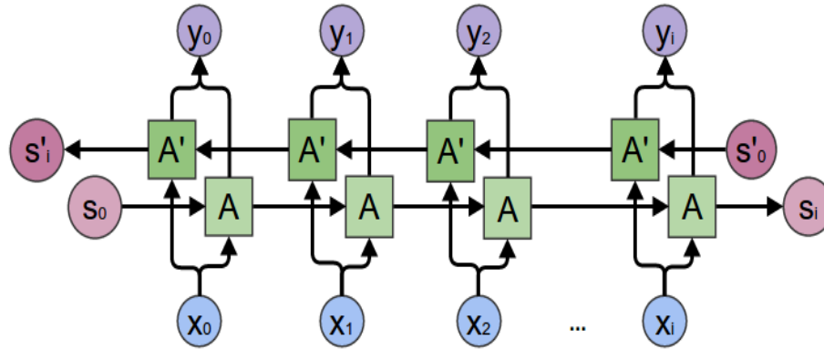
Şekil 3. 4. Bi-LSTM Yapısı
