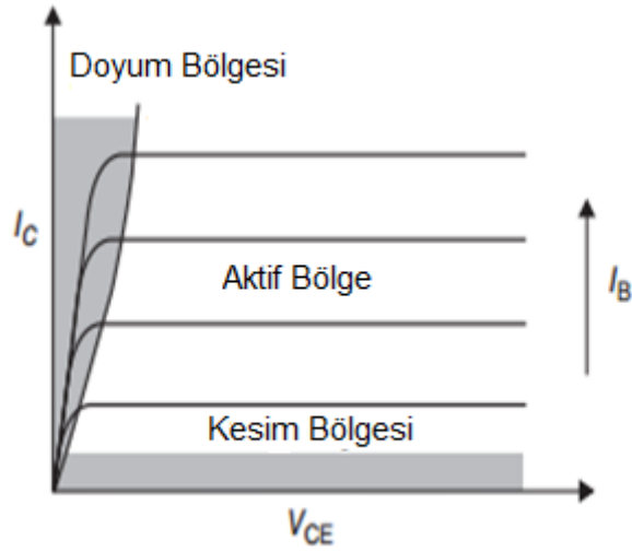
Şekil 2.7. npn transistörde çıkış karakteristiği [22]
