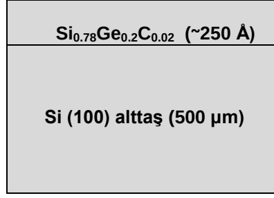
Şekil 3.2. Silisyum pul yüzeyine epitaksiyel SiGeC film büyütme şematik gösterimi
