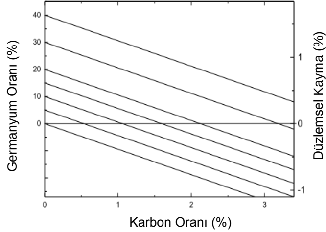
Şekil 2.13. Kristal kafes yapısı içerisinde karbon-germanyum oranının kristal kusurlar üzerindeki etkisi [39]
