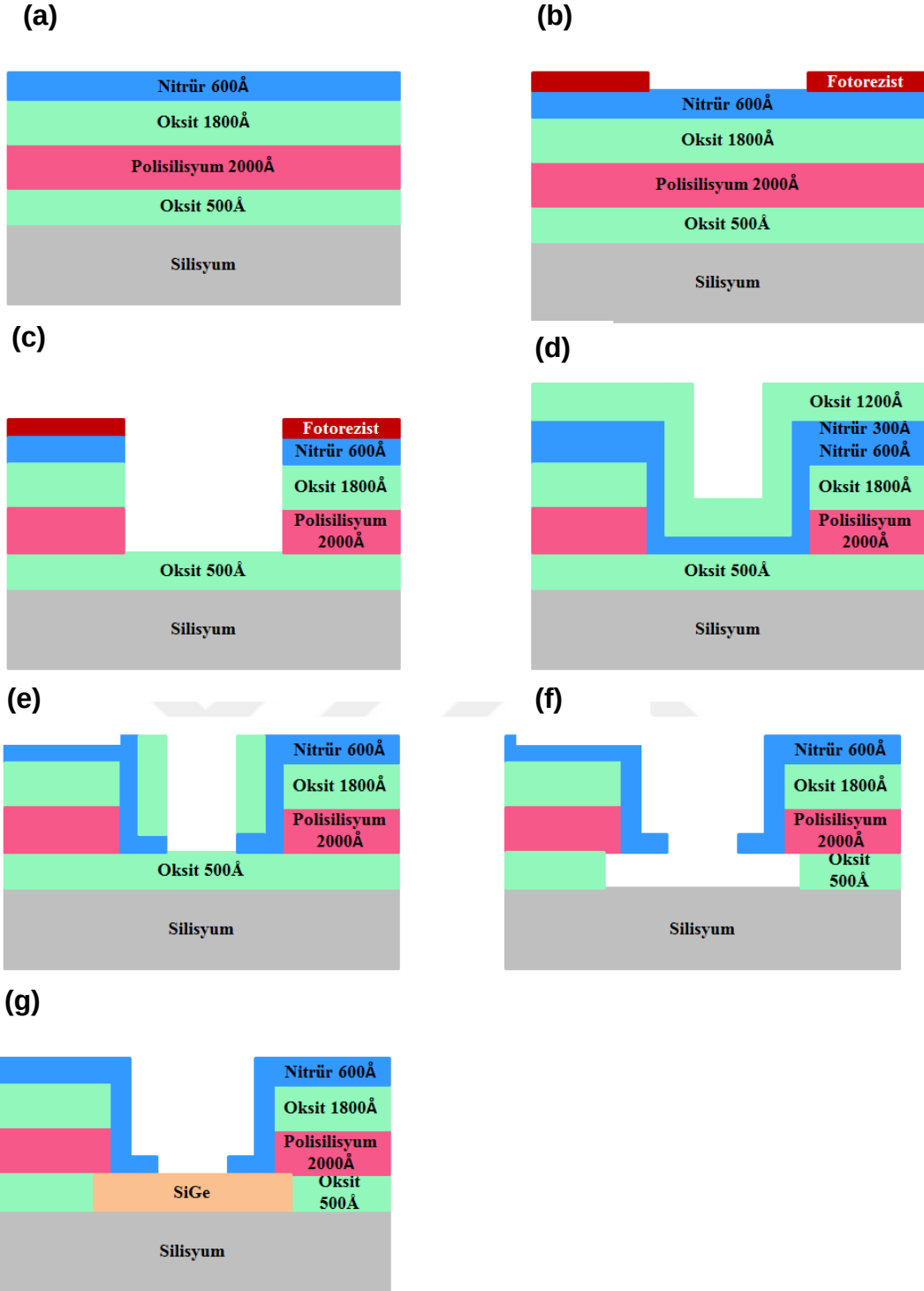
Şekil 3.4. Seçici epitaksiyel SiGeC film büyütme işlem basamaklarının şematik gösterimi; (a) Silisyum pul üzerine sırasıyla 500 Å silisyumdioksit, 2000 Å polisilisyum, 1800 Å silisyumdioksit, 600 Å silisyum nitrid filmleri büyütme (b) Baz çukuru fotorezist şekillendirme (c) Baz çukuru kuru aşındırma (d) Yan duvar 300 Å silisyum nitrid ve 1200 Å silisyumdioksit filmleri büyütme (e) Yan duvar kuru aşındırma (f) Polisilisyum altı silisyumdioksit filmi ıslak aşındırma (g) Seçici epitaksiyel SiGeC film büyütülen pul örneği
