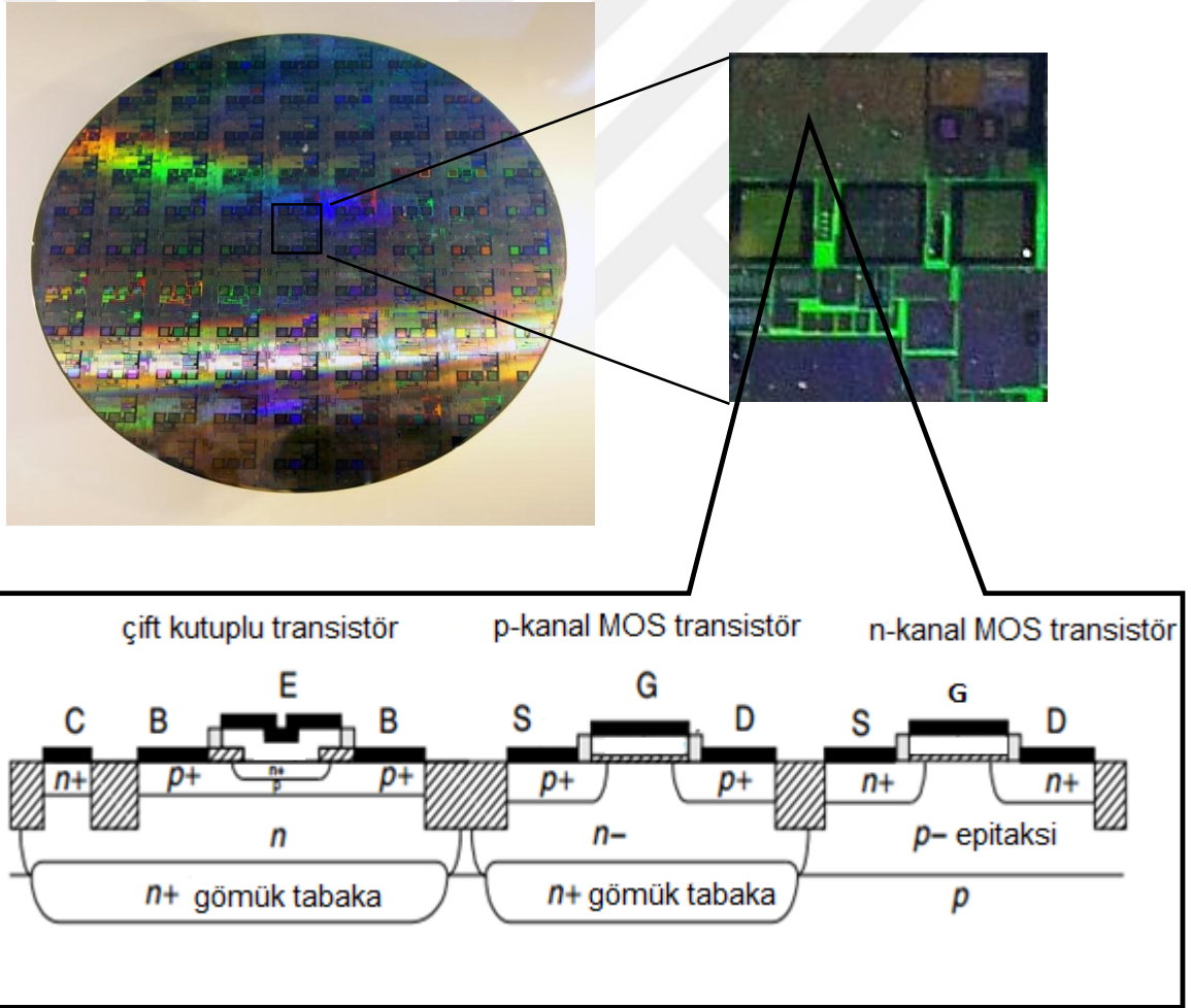
Şekil 2.8. Tümdevre üretiminin şematik gösterimi (a) SiGeC BiCMOS üretilmiş 100 mm silisyum pul (b) Silisyum pulda bulunan birinin aynısı olan 94 kırmıktan biri (c) SiGeC BiCMOS transistör yapısı [20]
