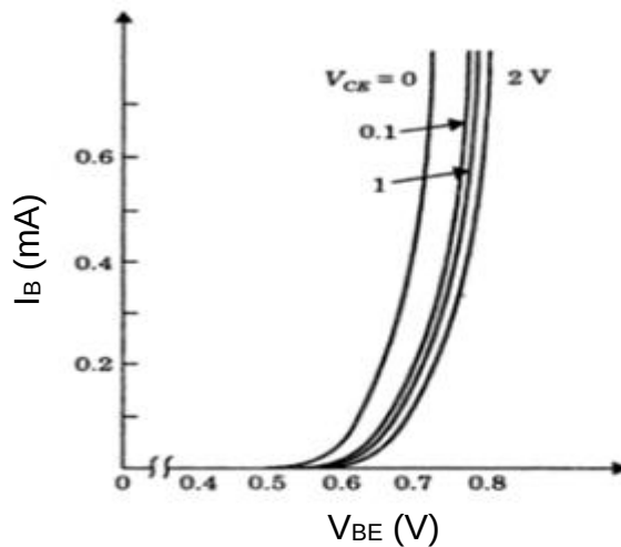
řekil 2.6. npn transistrde giriř karakteristiėi [21]
