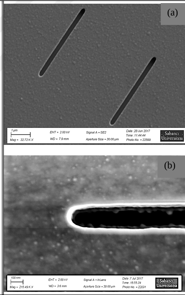
Şekil 4.4. 20 ml/dk HCl akış hızı ile transistor baz çukuruna büyütülen filmin SEM görüntüleri (a) ikili transistor (b) tek transistor
