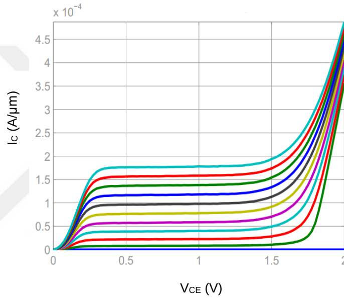
Şekil 4.17. Transistör çıkış karakteristiği (a) kutuplanma (b) kolektör-emiter gerilimine karşı kolektör akımı değişim grafiği
