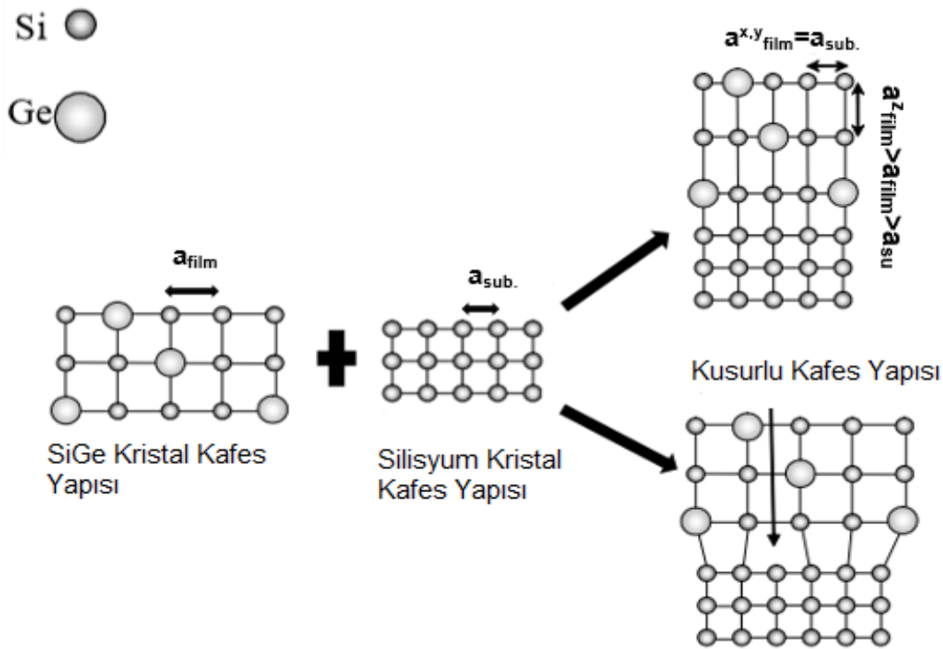
Şekil 2.11. Silisyum üzerine büyütülen gerinmiş ve kusurlu formda \text{Si}_{1-x}\text{Ge}_x film yapısı [36]
