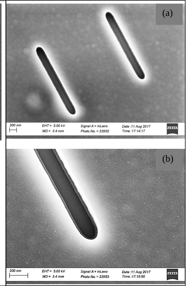
Şekil 4.5. 25 ml/dk HCl akış hızı ile transistor baz çukuruna büyütülen filmin SEM görüntüleri (a) ikili transistor (b) tek transistor
