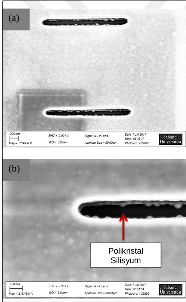
Şekil 4.9. 15ml/dk HCl akış hızı ile transistör baz çukuruna büyütülen filmin SEM görüntüleri (a) ikili transistör (b) tek transistör
