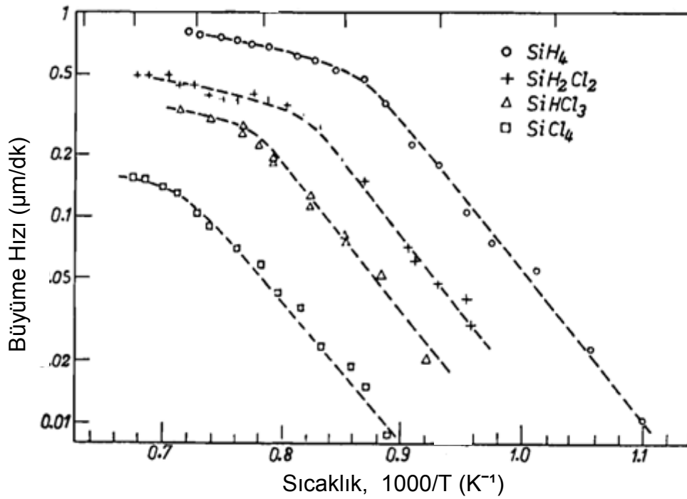
Şekil 2.16. Farklı silisyum kaynaklarında sıcaklığa bağlı film büyüme hızı değişim grafiği (Bütün reaktantlar ~0.1 mol \text{H}_2 gazı içerir) [25]
