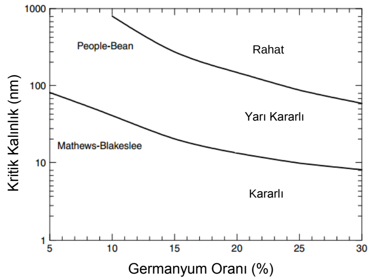
Şekil 2.12. SiGe kafes yapısında germanyum oranına bağı kritik SiGe film kalınlığı değişimi [36]
