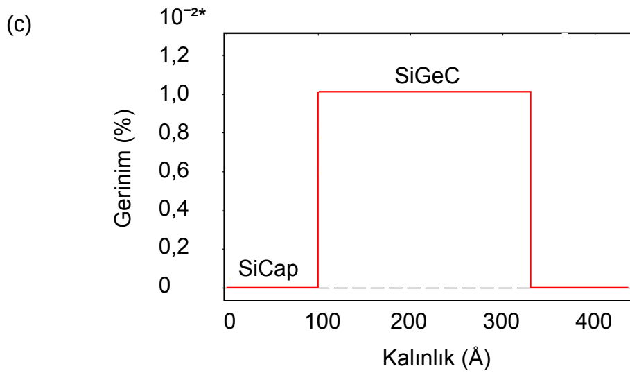
Şekil 4.13. Benzetim programıyla elde edilen veriler (a) Ölçüm (kırmızı) ve benzetim (yeşil) \omega/2\theta verilerinin karşılaştırılması (b) SiGeC film içerisindeki germanyum oranı ve profili (c) Film gerinim yüzdesi
