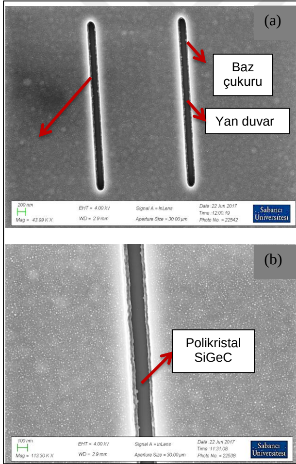
Şekil 4.3. 15 ml/dk HCl akış hızı ile transistor baz çukuruna büyütülen filmin SEM görüntüleri (a) ikili transistor (b) tek transistor
