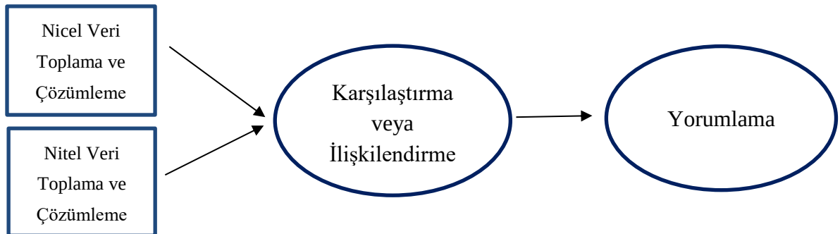
Şekil 2. Yakınsayan paralel desen modeli
