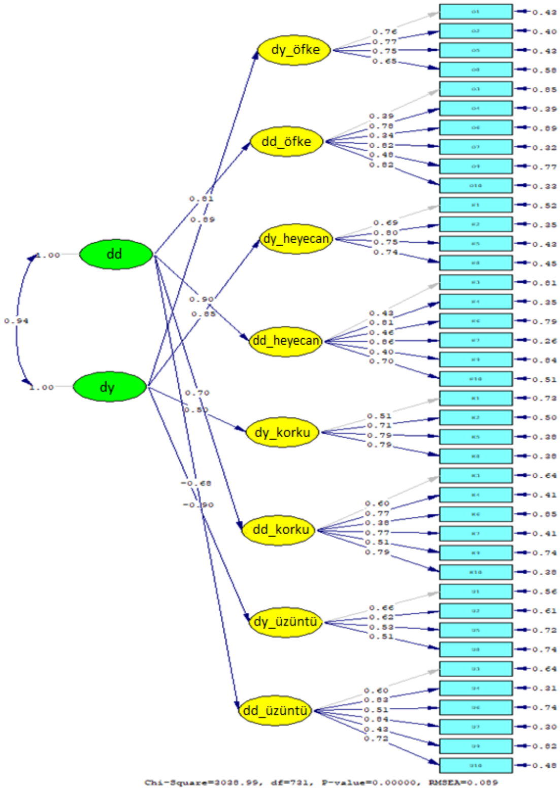
Şekil 7. ÇDDÖ-YF'na ilişkin ikinci düzey DFA sonucu elde edilen yol diyagramı (Standartlaştırılmış değerler)
