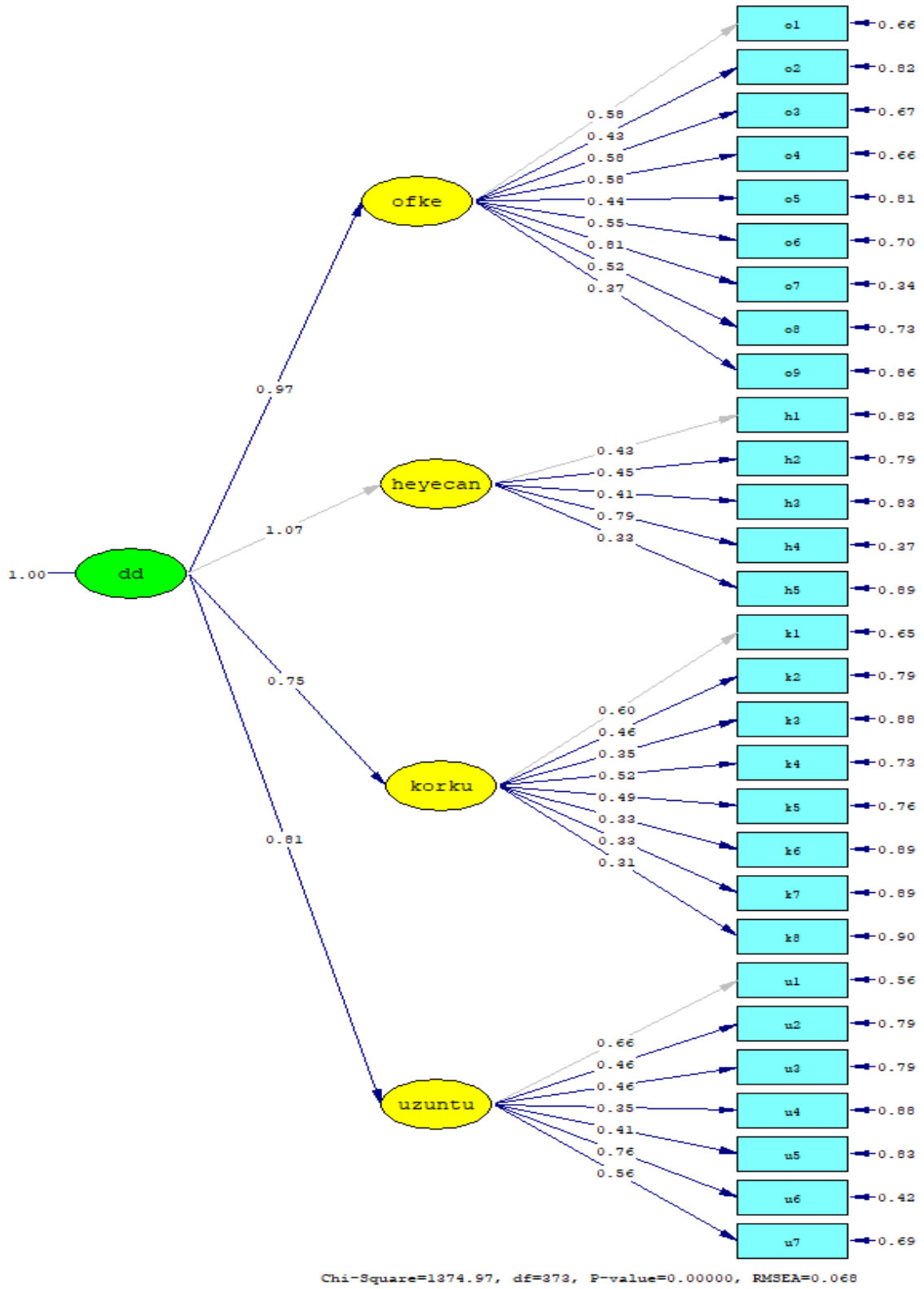
Şekil 5. ÇDDÖ'ne ilişkin ikinci düzey DFA sonucu elde edilen yol diyagramı (Standartlaştırılmış değerler)
