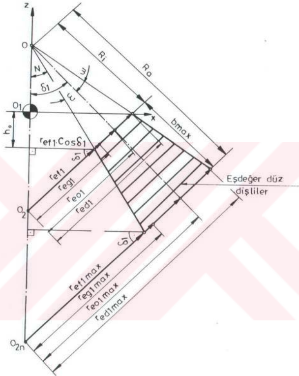
Şekil 4.17. Tredgold yaklaşımı dikkate alınarak konik düz dişi üzerinde eşdeğer düz dişlilerin oluşturulması.
