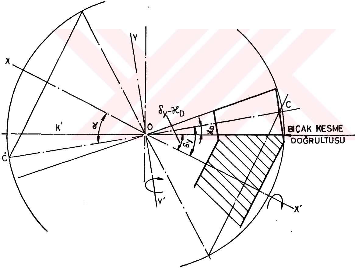
Şekil 3.10. Bilgram sistemi, yuvarlanma metoduna göre konik dişli imalatı.
