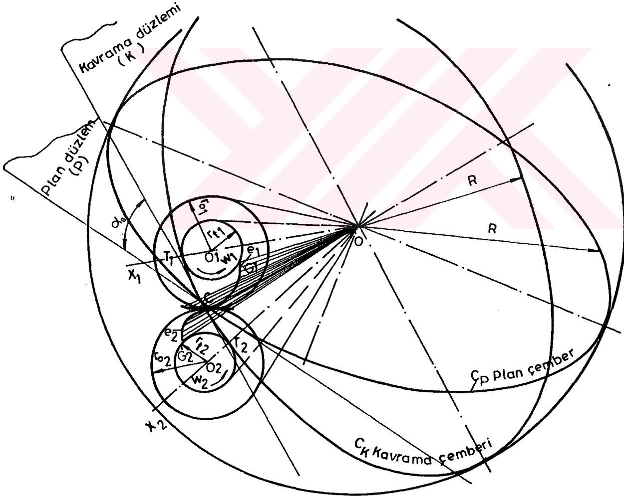
Şekil 2.4. Konik dişli taslaklarının yuvarlanma düzlemleri.
