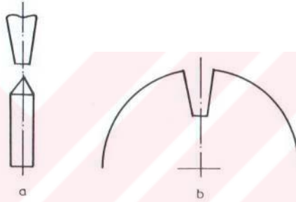
Şekil 3.19. Konik dişli kesmek için, a) kalemin eksilenmesi, b) ilk diş boşluklarının açılması.
