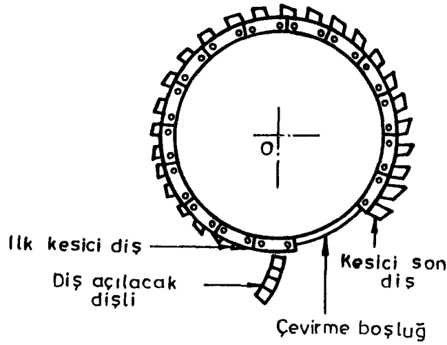
Şekil 3.5. Boşaltma usulü konik dişli kesme ( Tığ çekme ).
