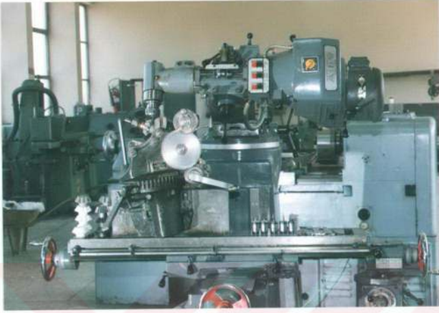
Şekil 4.2b. Aparatın kalıpcı freze tezgahına bağlanması.
