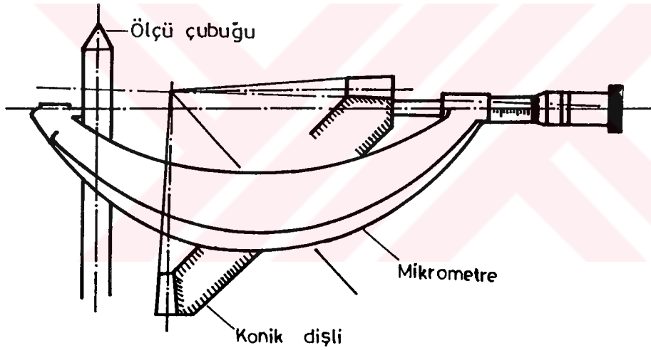
Şekil 3.24. Koni uzunluğunun ölçülmesi.
