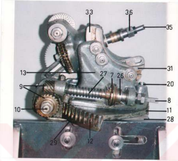
Şekil 3.17b. Matterson aparatının sol yan görünüşü.
