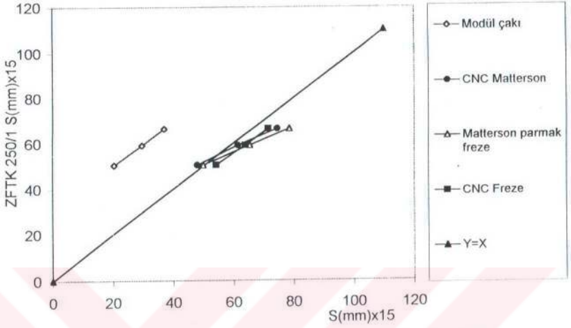
Şekil 5.1. ZFTK 250/1 Referans dişlisine göre S_1 , S_2 ve S_3 değerlerinin değişimi.
