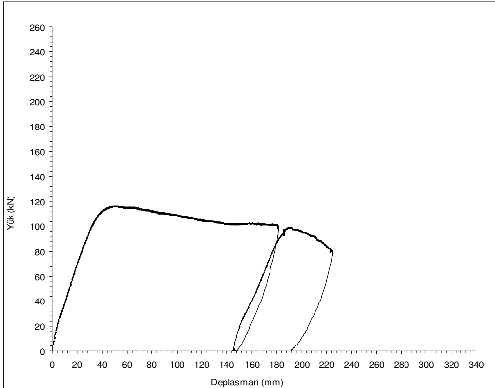
řekil 5.7. R_N kiriři yk-deplasman grafiđi
