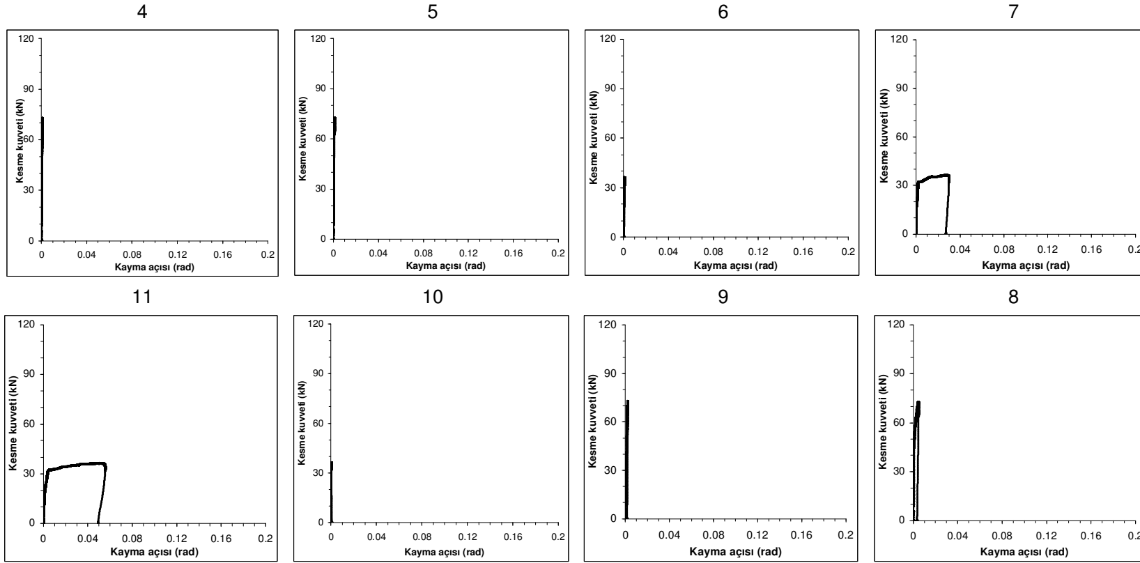
Şekil 2.2. B N kirişi kesme kuvveti-kayma açısı grafikleri
