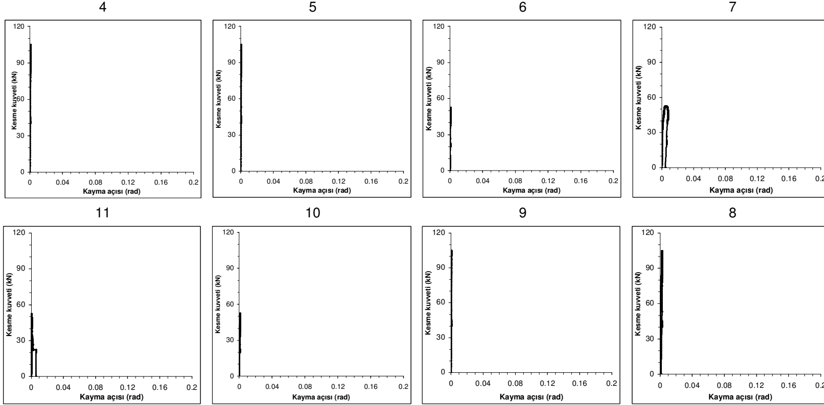
Şekil 2.3. B B kirişi kesme kuvveti-kayma açısı grafikleri
