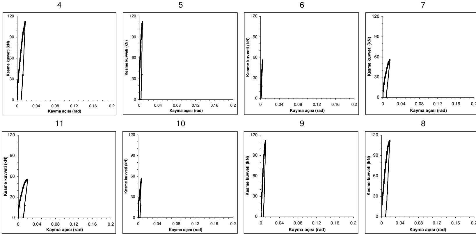
Şekil 2.6. C_{BX} kirişi kesme kuvveti-kayma açısı grafikleri
