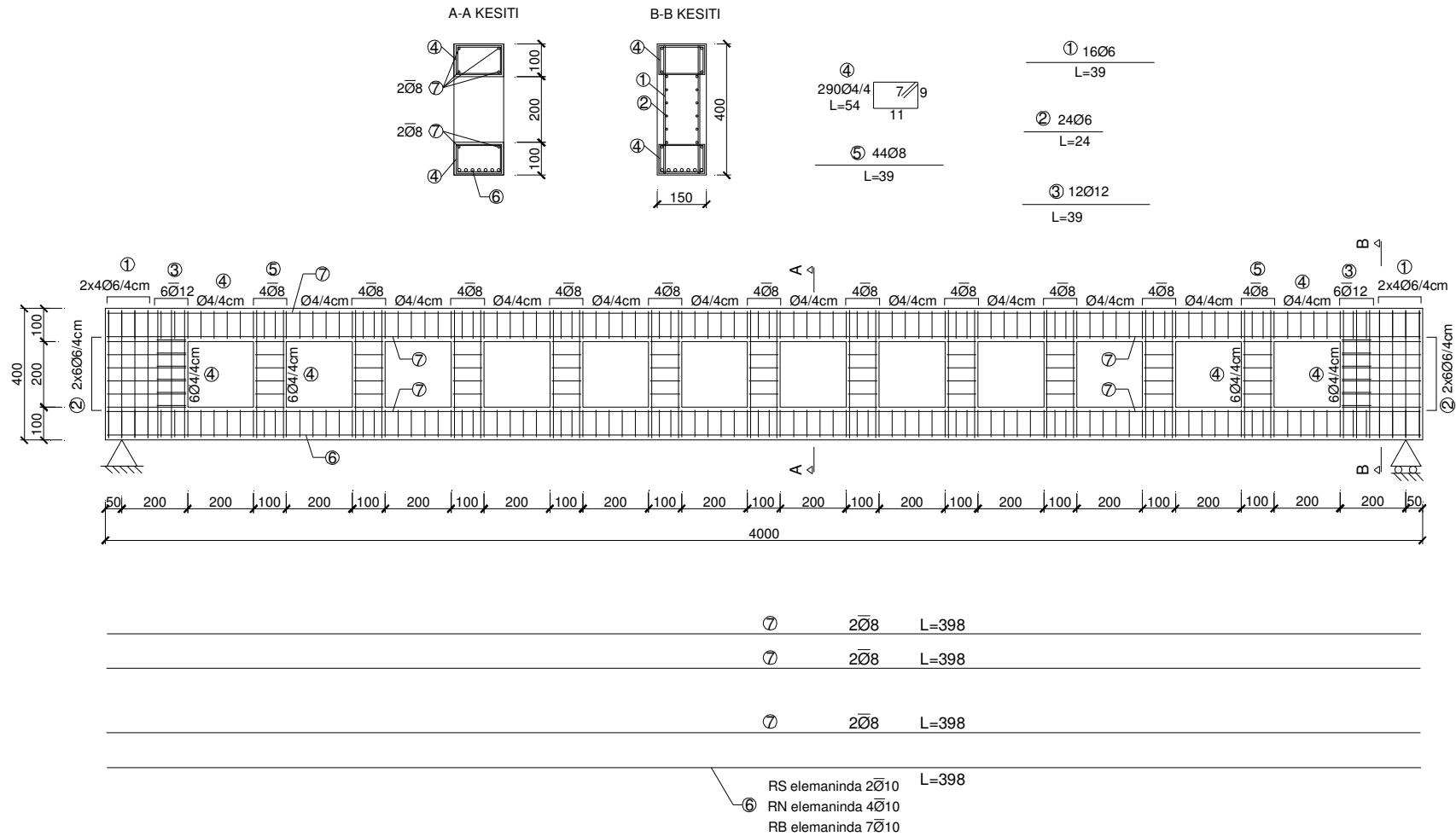
Şekil 1.2. R kodlu giriş donatı detay çizimi
