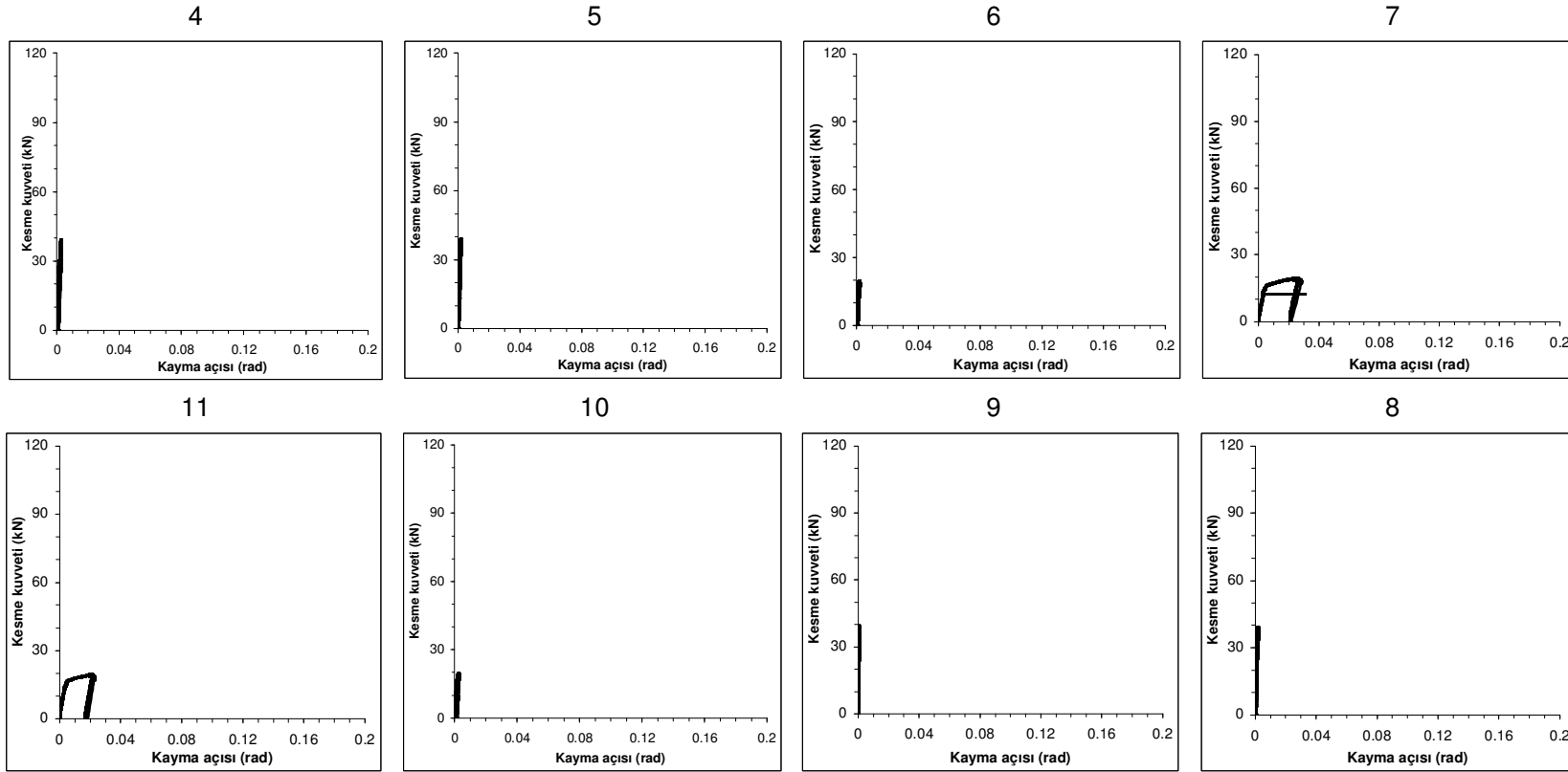
Şekil 2.4. C_{SX} kirişi kesme kuvveti-kayma açısı grafikleri
