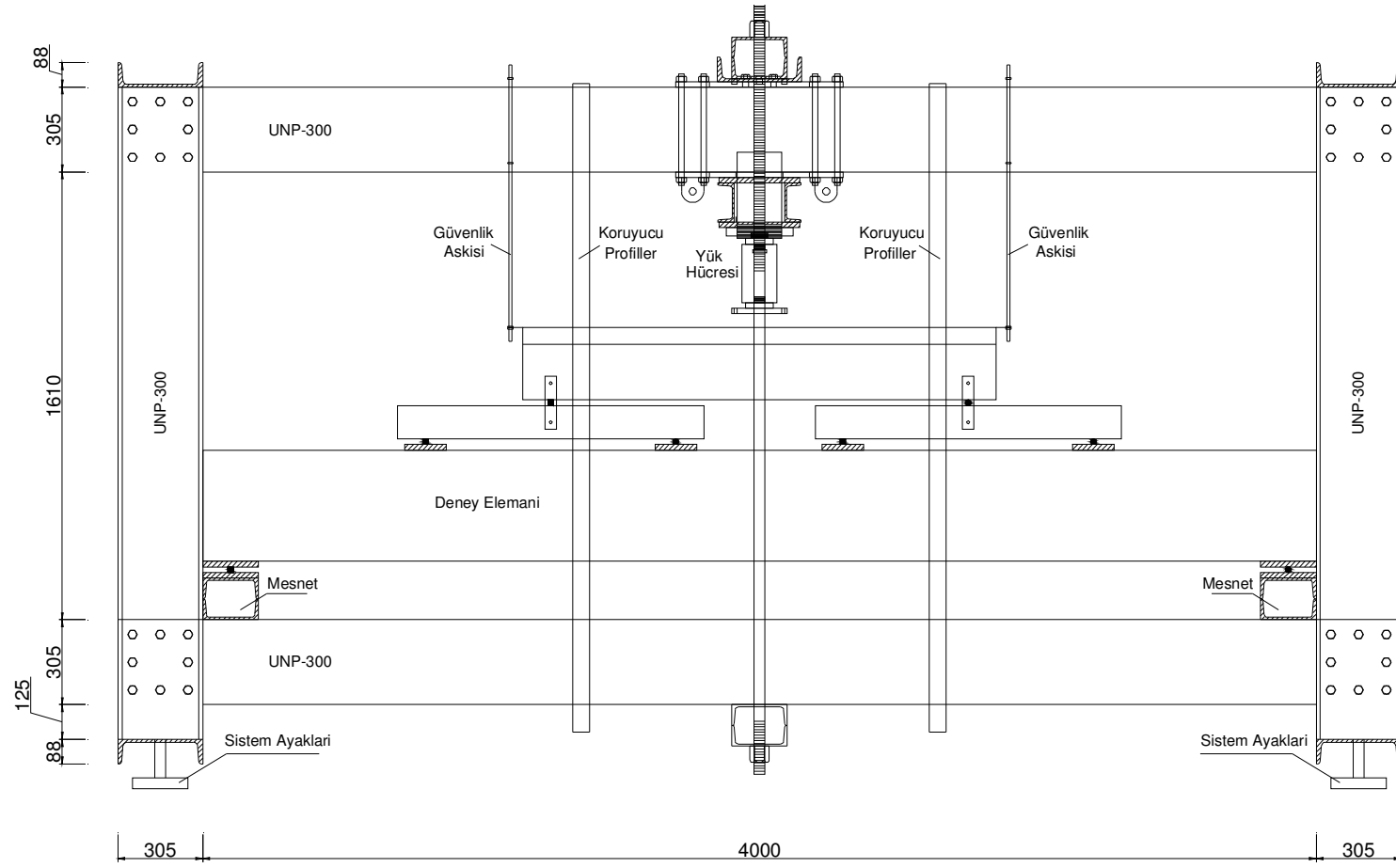
Şekil 4.3. Yükleme Düzeneği Genel Görünüşü
