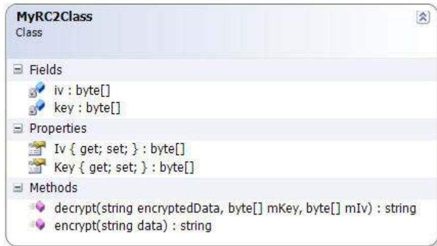
Şekil 4.10. MyRC2Class sınıf diyagramı
