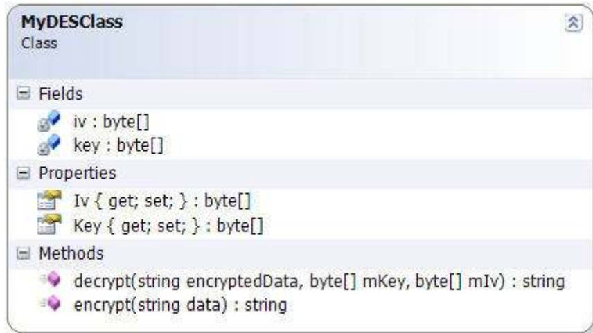
Şekil 4.8. MyDESClass sınıf diyagramı
