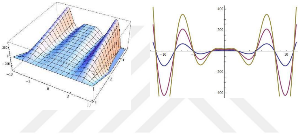
Şekil 4.3. (r - \varepsilon_t \varepsilon_T \varepsilon_N \kappa)(s, t) evolüsyon
