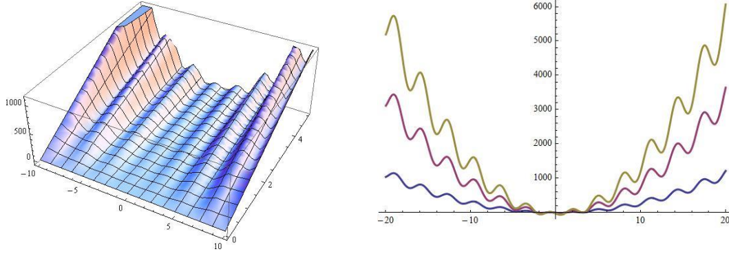
Şekil 4.2. k(s, t) evolüsyonu
