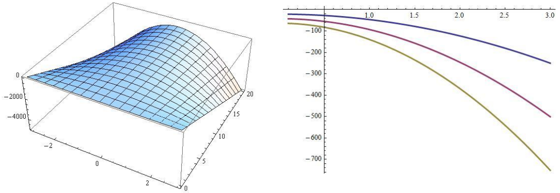
Şekil 4.6. (r - \varepsilon_t \varepsilon_T \varepsilon_N \kappa)(s, t) evolüsyonu
