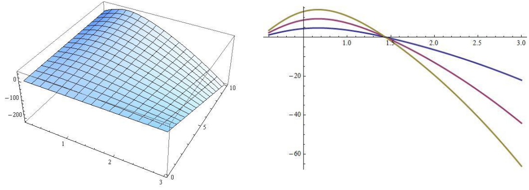
Şekil 4.4. \kappa(s, t) evolüsyonu
