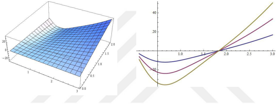
Şekil 4.5. \kappa(s, t) evolüsyonu
