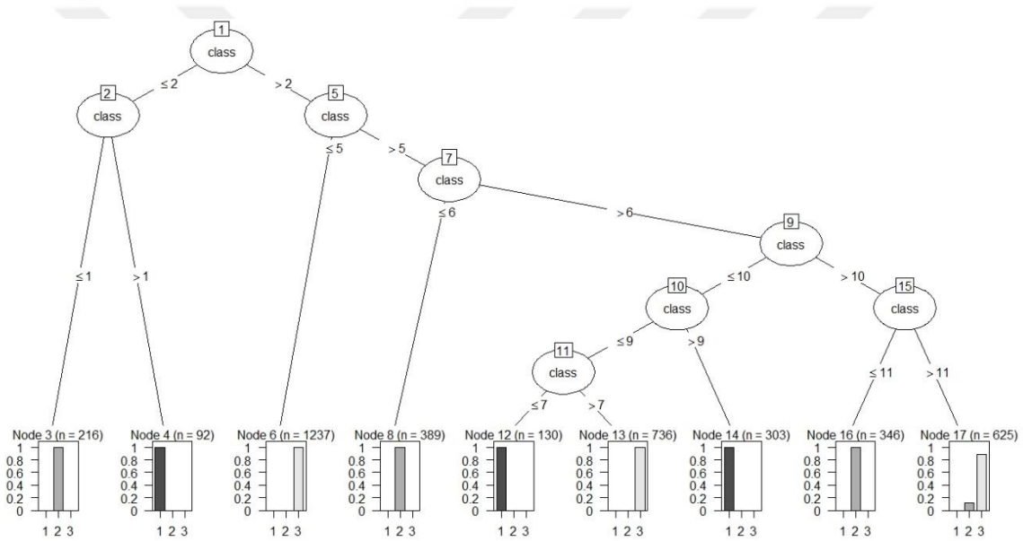
Şekil 4. 1. C5.0 Karar Ağacı Modeli
