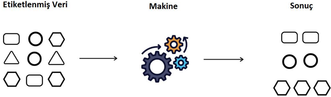
Şekil 1. 5. Denetimsiz Öğrenme
