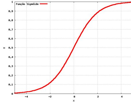
Şekil 2. 6. Sigmoid Fonksiyonu
