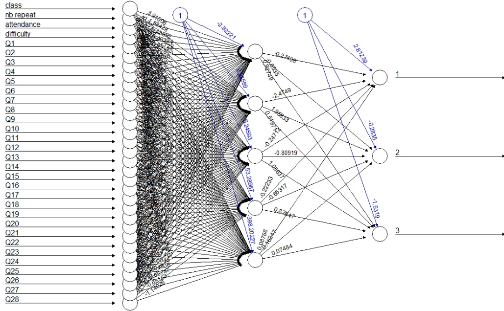
Şekil 4. 2. Yapay Sinir Ağları Modeli
