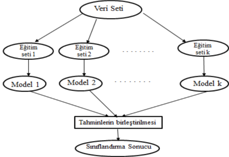
Şekil 2. 3. Rastgele Orman
