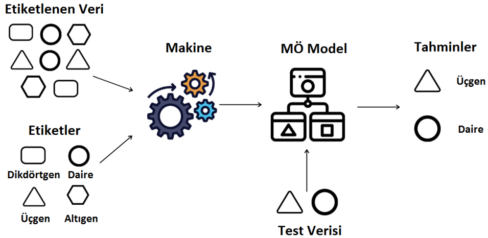
Şekil 1. 8. Denetimli Öğrenme
