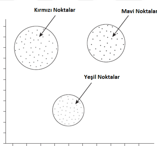
Şekil 1. 7. Kümeleme Grafiği
