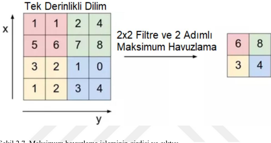
Şekil 2.7. Maksimum havuzlama işleminin girdisi ve çıktısı.
