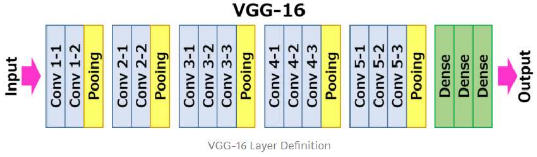
Şekil 4.1. VGG-16 mimarisi
