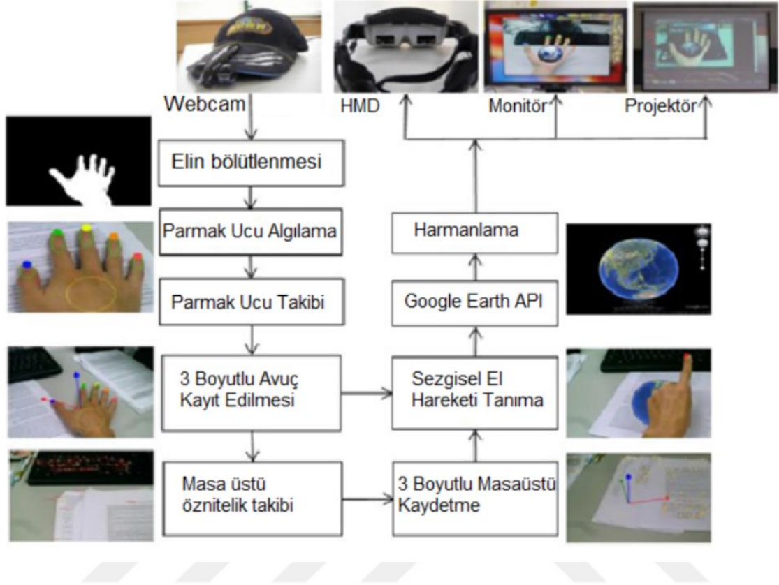
Şekil 1.6. VECAR sisteminin akış şeması görseli [16]
