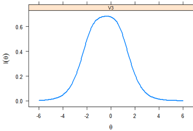
Şekil 10. Üçüncü Maddenin Bilgi Fonksiyonu Grafiği
