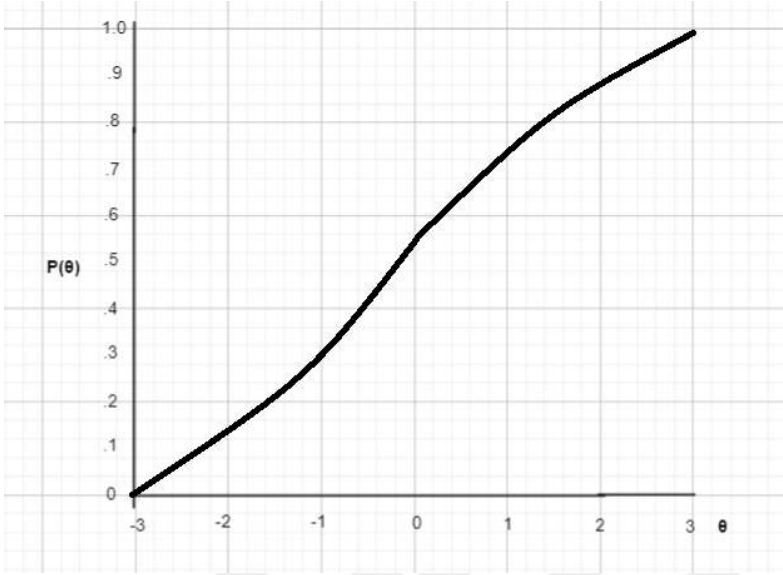
Şekil 3. b Parametresi 0 ve a Parametresi 1.7 olan MKE
