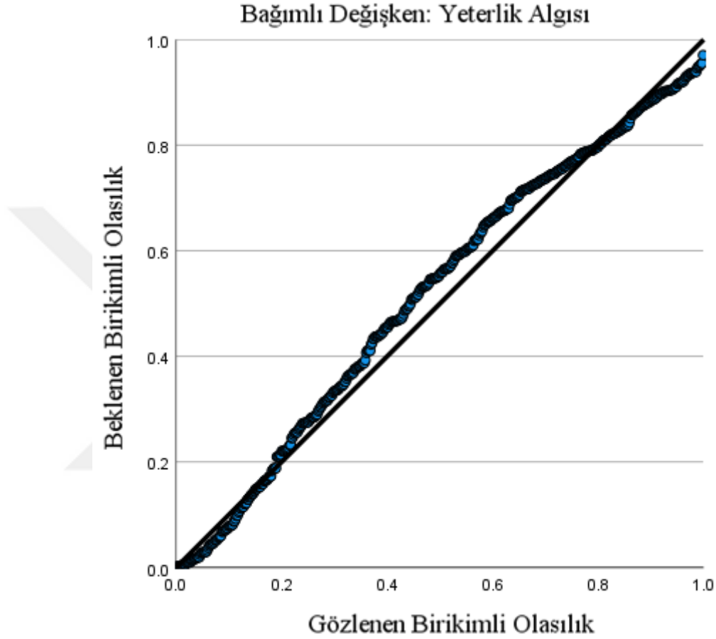
Şekil 4.2. Beklenen ve gözlenen birikimli olasılık değerlere ait P-P grafiği
