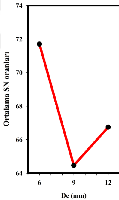
Şekil 4.5. Basma testi sonuçlarına göre Dc faktörü için ortalama SN oranları grafiği
