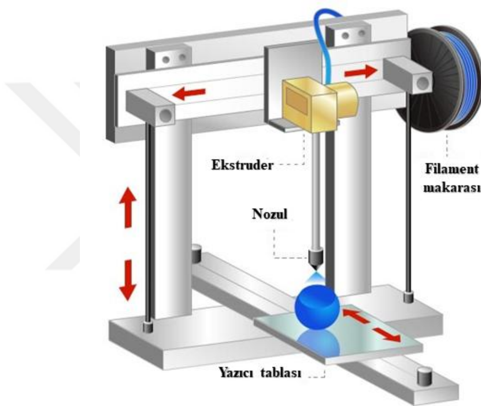
Şekil 1.1. 3D yazıcının çalışma prensibi (Nanoteknoloji, 2023).
