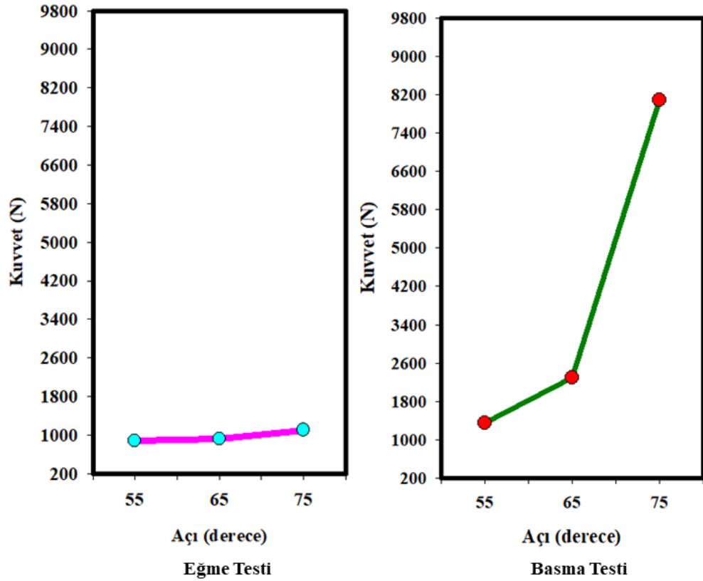
Eğme ve Basma testi ortalama sonuçlarının Açı faktörü açısından kıyaslanması
