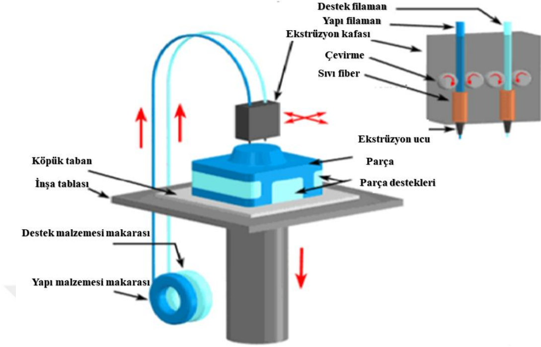
Şekil 1.7. FDM makinesinin bileşenleri (Chua et al., 2014).
