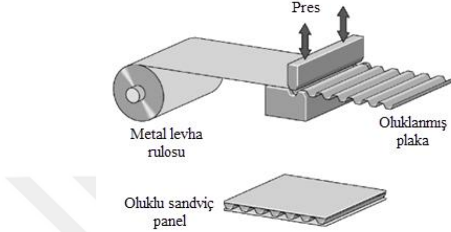
Şekil 1.16. Oluklu sandviç panel plakaların üretimi (Wadley, 2006).
