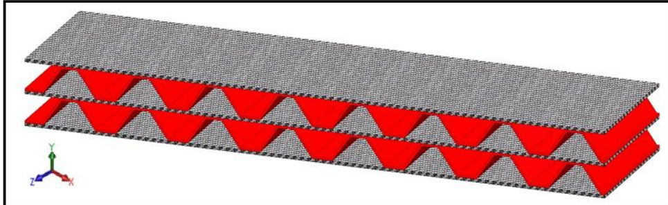
Şekil 3.16. İki Katlı PLA-carbon fiber plaka ve PLA çekirdek hücrenin iki bileşenli epoksi yapıştırıcı ile yapıştırıldıktan sonraki montaj hali
