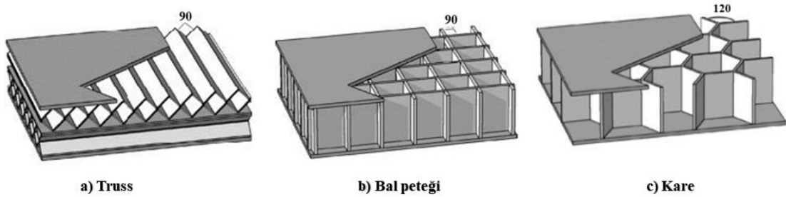
Şekil 1.13. Periyodik hücre dizilimine sahip hücreli yapılar (Wadley, 2006).
