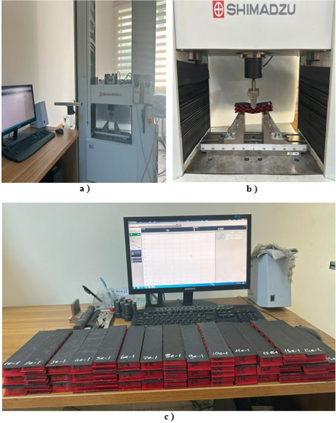
Şekil 3.24. a) Shimadzu AG-IC eğme testi cihazı eğme ünitesi b) Eğme numunesinin test cihazındaki konumu c) Numunelerin deney öncesi görüntüleri
