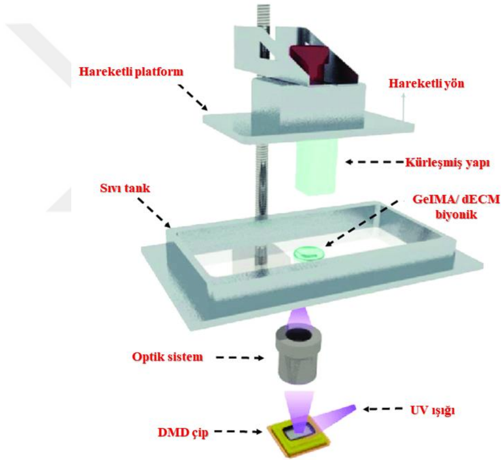
Şekil 1.4. DLP yazıcısının ana bileşenleri (Williams & Zhang 2021).
