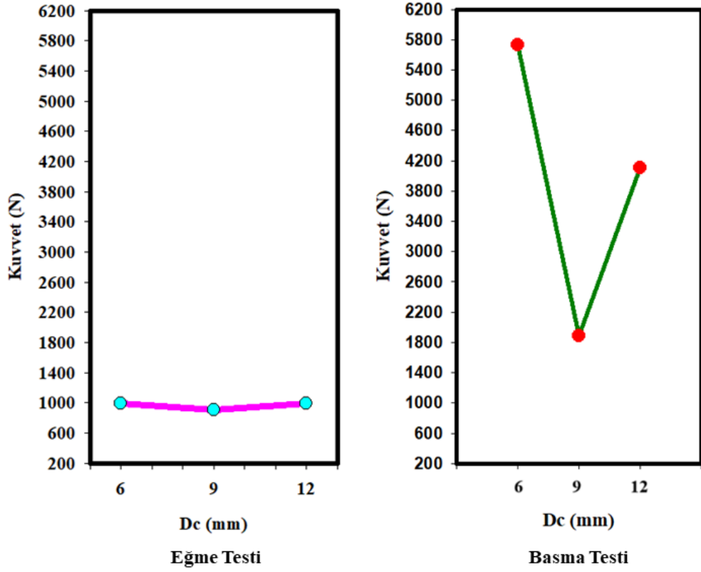
Şekil 4.42. Üç nokta eğme ve basma deneylerinden ortaya çıkan mukavemet sonuçlarının Dc faktörüne göre kıyaslanması
