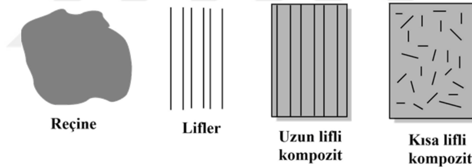
Şekil 1.12. Polimer matrisli kompozit malzemenin şematik gösterimi (Dursun ve Ozbay 2008).
