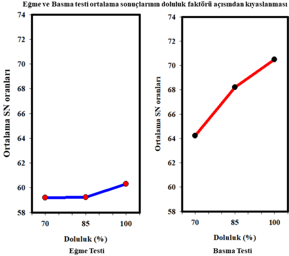
Şekil 4.38. Üç nokta eğme ve basma deneylerinden ortaya çıkan ortalama sonuçların SN oranlarının Doluluk faktörüne göre kıyaslanması
