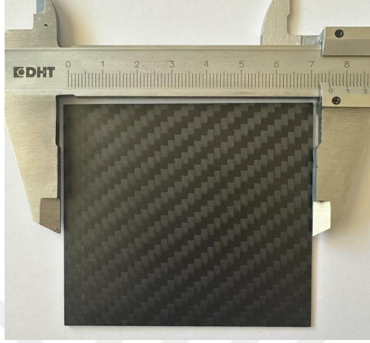
Şekil 4.49. Eni boyu 75X75 mm ve 1 mm kalınlıĝa sahip %100 karbon fiber plaka
