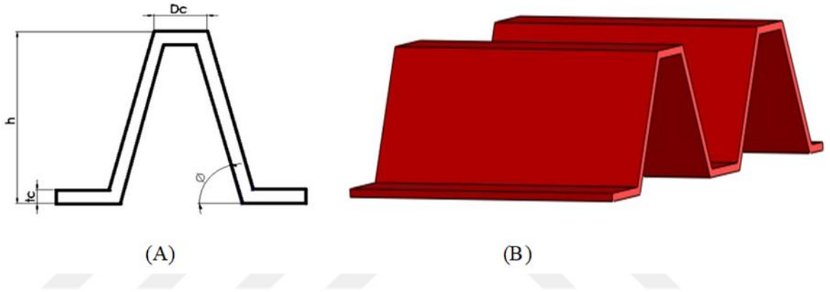
Şekil 3.2. A) Trapezoid hücre ölçülerinin şekil üzerinde gösterilmiş hali B) Eni boyu 75X75mm trapezoid hücrenin katı modeli
