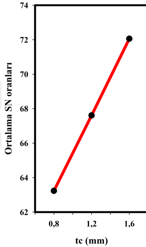
Şekil 4.6. Basma testi sonuçlarına göre tc faktörü için ortalama SN oranları grafiği
