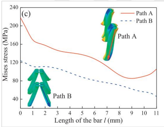
Şekil 2.62. Yapı üzerindeki kirişlerdeki gerilme dağılımı [114]
