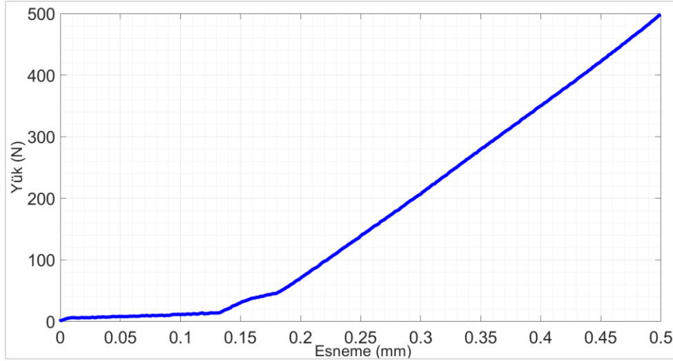
Şekil 4.1. Alüminyum plaka için yük-esneme grafiği
