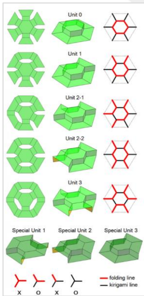
Şekil 2.16. Kafes kiriş yapısı temelli krigami [74]
