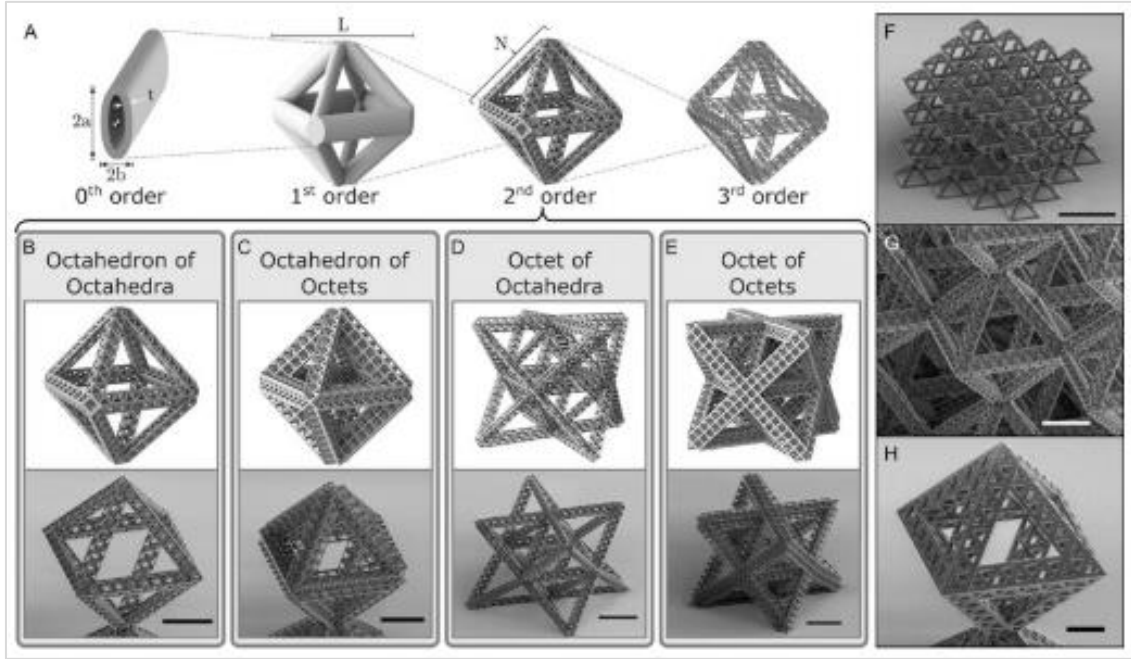
Şekil 2.7. Çeşitli tiplerde nano boyuttaki kafes kiriş yapılar [40]
